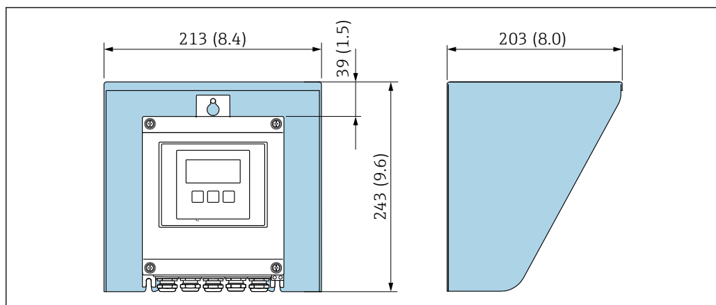
図 28 Proline 500 – デジタル用の日除けカバー、単位 mm (in)
