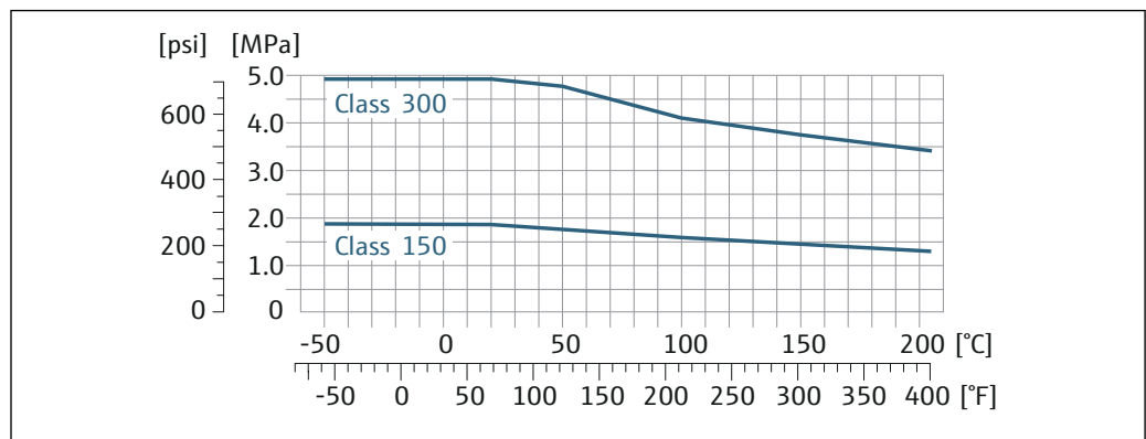
図 32 フランジ材質 1.4301 (SUS 304 相当) ; 接液部 : ジルコニウム 702、タンタル
