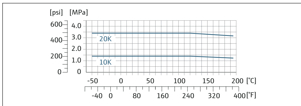
図 33 フランジ材質 1.4301 (SUS 304 相当) ; 接液部 : ジルコニウム 702、タンタル
