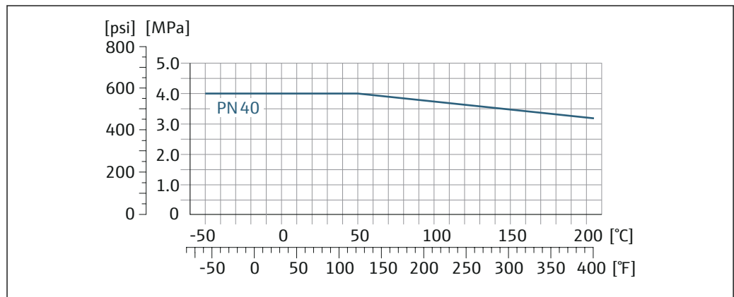
図 31 フランジ材質 1.4301 (SUS 304 相当) ; 接液部 : ジルコニウム 702、タンタル
