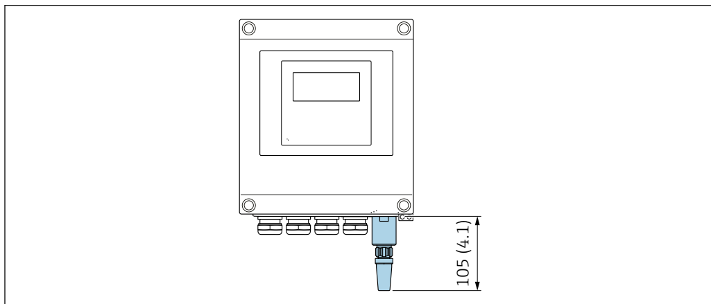
図 37 単位 mm (in)
