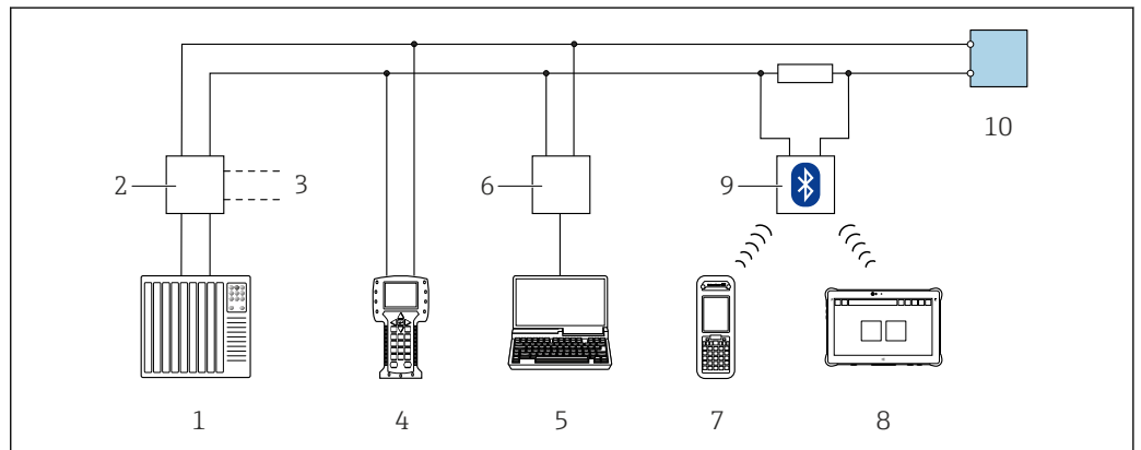
図 50 HART プロトコル経由のリモート操作オプション（パッシブ）
