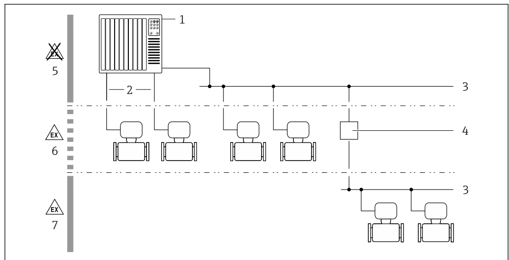
1 機器のシステムへの統合例
