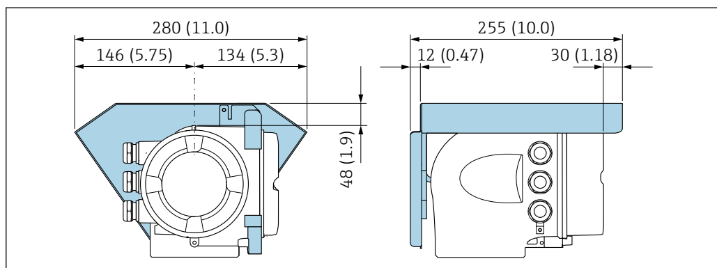
図 29 Proline 500 用の日除けカバー、単位 mm (in)
