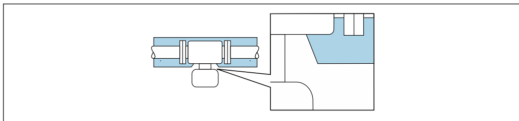
図 40 伸長ネックを覆わない断熱
