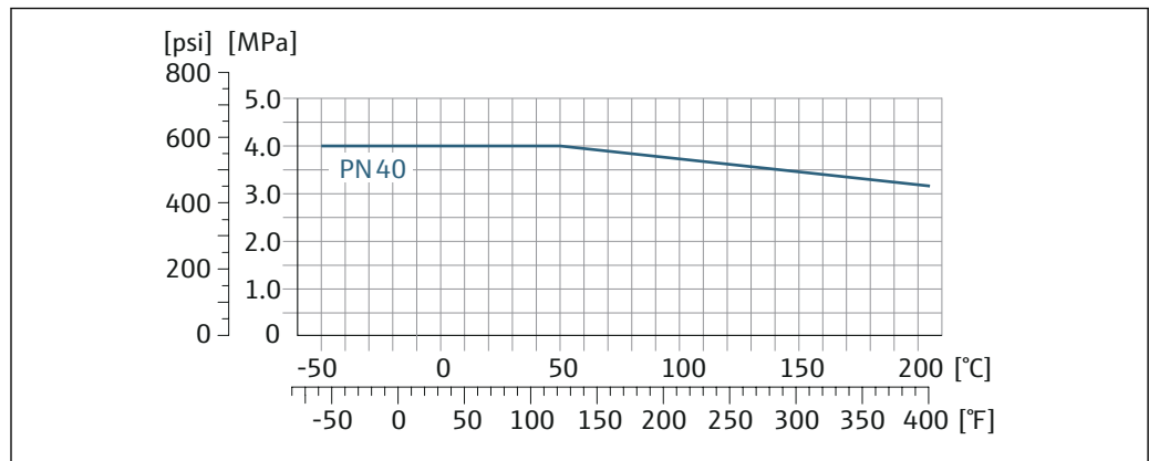
図 31 フランジ材質 1.4404 (SUS F316 または F316L 相当)
