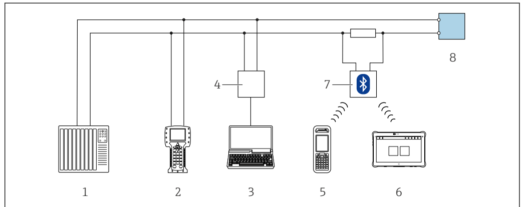
図 59 HART プロトコル経由のリモート操作用オプション (アクティブ)
