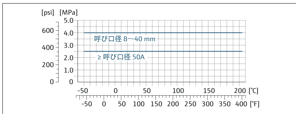
図 39 接続部の材質 1.4435 (SUS 316L 相当)
