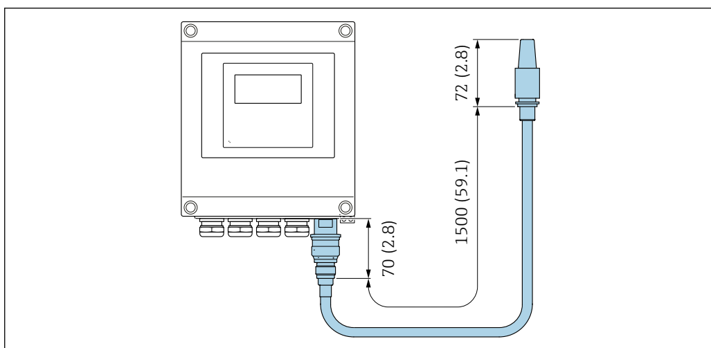
☐ 47 単位 mm (in)
