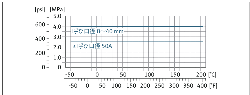
図 35 フランジ材質 1.4435 (SUS 316L 相当)
