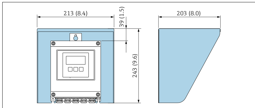
図 51 Proline 500 – デジタル用の日除けカバー、単位 mm (in)
