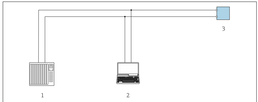
図 32 Modbus-RS485 プロトコル経由のリモート操作オプション (アクティブ)
