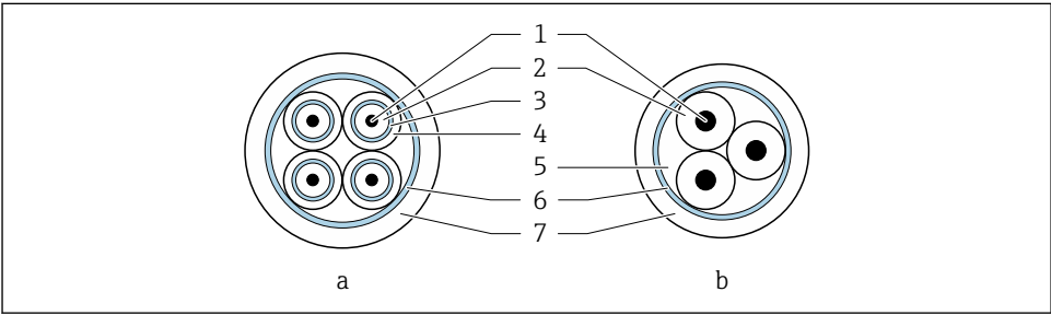
图 3 电缆横截面
