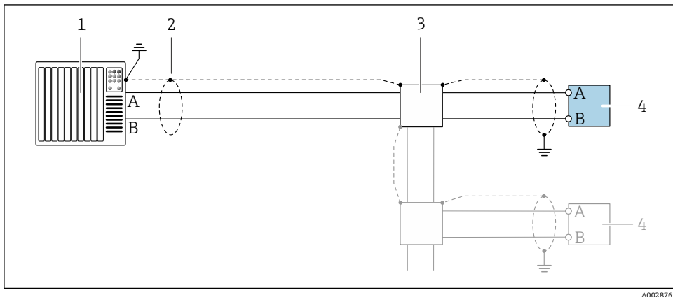
图 5 接线示例，Modbus RS485，非防爆区和防爆区（Zone 2；Cl. I, Div. 2）
