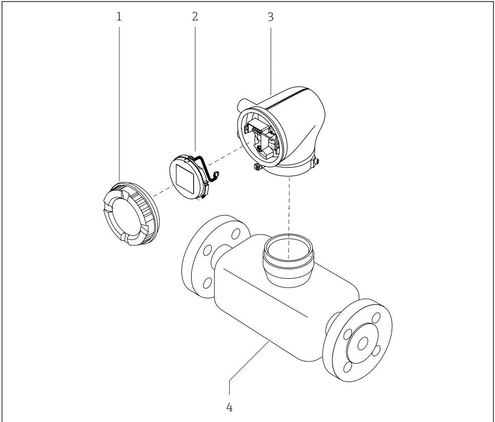
图 1 仪表主要结构部件
