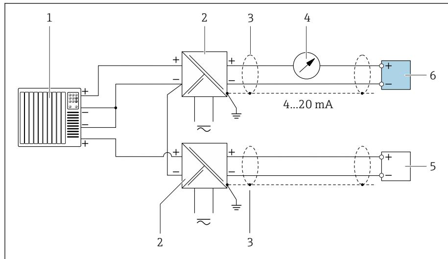
10 Exemple de raccordement pour entrée HART avec "moins" commun (passive)
