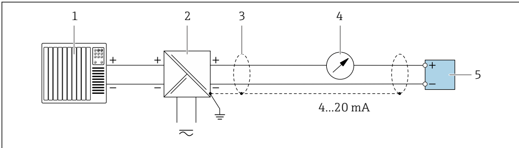
图 9 接线实例：4...20 mA HART 电流输出（无源信号）
