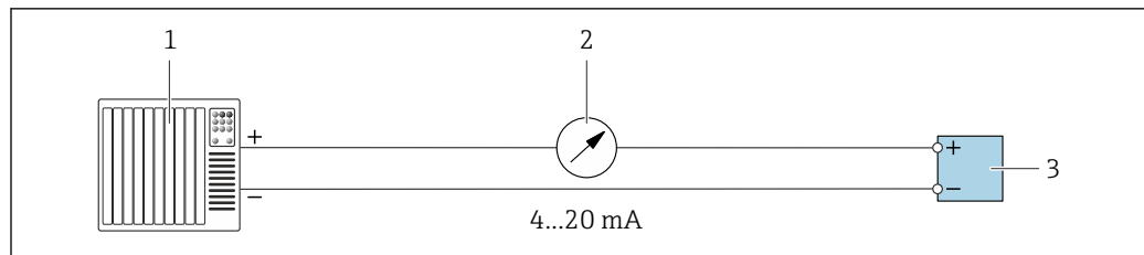
11 接线实例: 4...20 mA 电流输出 (有源信号)
