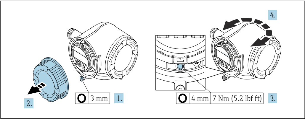
图 5 非防爆型外壳
