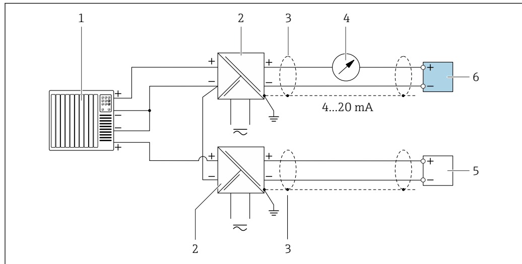
10 接线实例：HART 输入，公共端接负极（无源信号）
