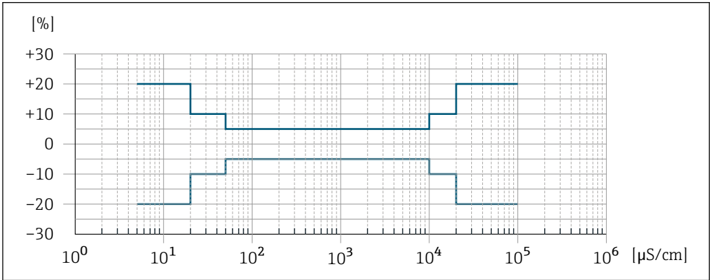
图 37 测量误差 (可选: 订购选项“电导率测量标定”, 选型代号 CW)
