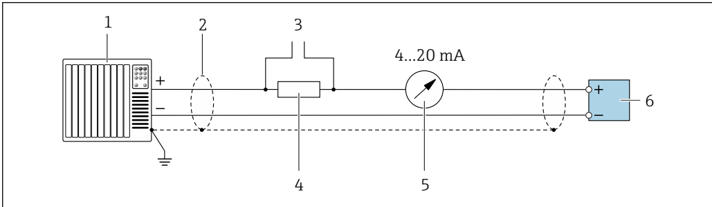
图 8 接线实例：4...20 mA HART 电流输出（有源信号）
