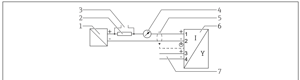
17 Blockdiagramm 2-Draht: 4 ... 20 mA HART, Schaltausgang
