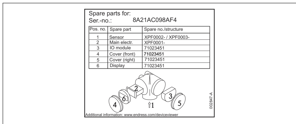
42 Beispiel für Ersatzteiltonschild im Anschlussraumdeckel
