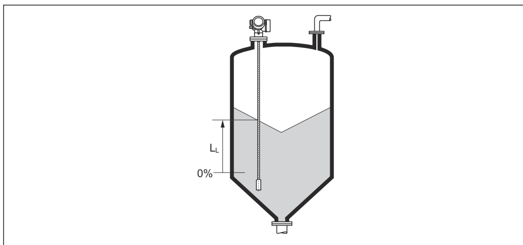
49 Füllstand bei Schüttgutmessungen
