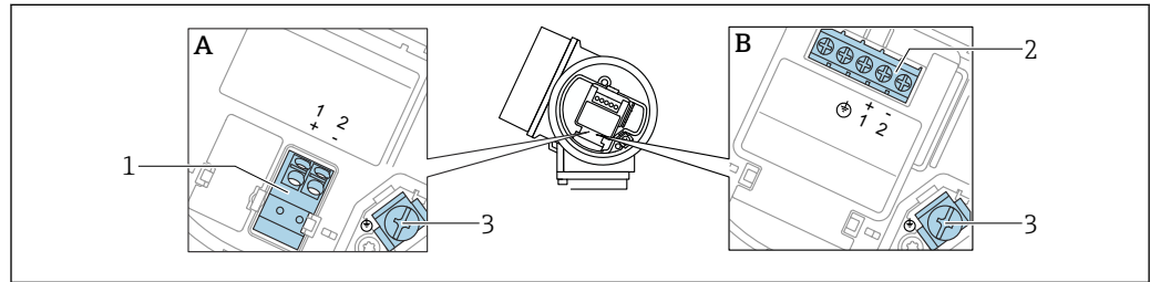
14 Klemmenbelegung 2-Draht: 4 ... 20 mA HART
