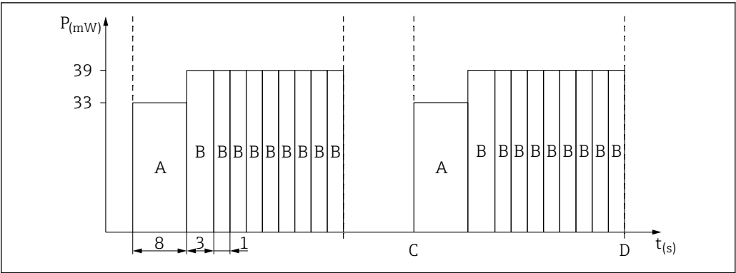
5 通过 RTU 启动或结束连续测量模式时的功耗 A 启动 B 测量 C 接通电源 D 切断电源
