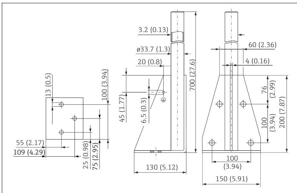
53 安装架 (短) 的外形尺寸。测量单位 mm (in)
