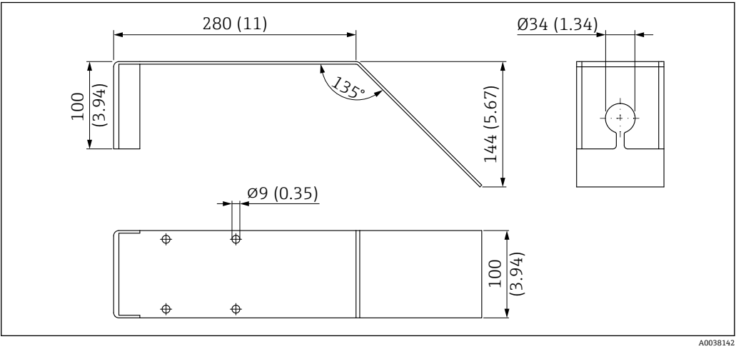
图 58 水平安装架（适用污水井）的外形尺寸。测量单位 mm (in)
