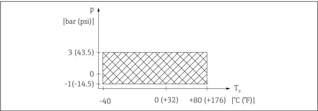
图 22 FMR20: 允许过程温度和过程压力
