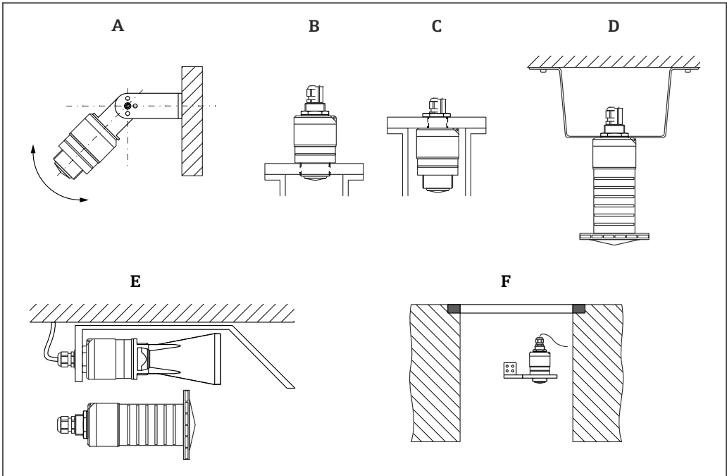
图 10 安装在墙壁上、罐顶上或安装短管中
