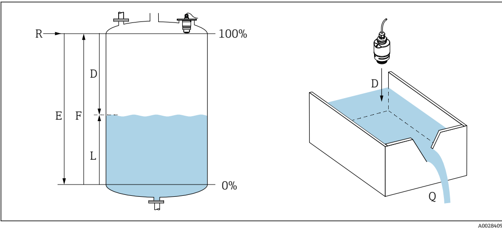
图 1 液位/流量标定参数
