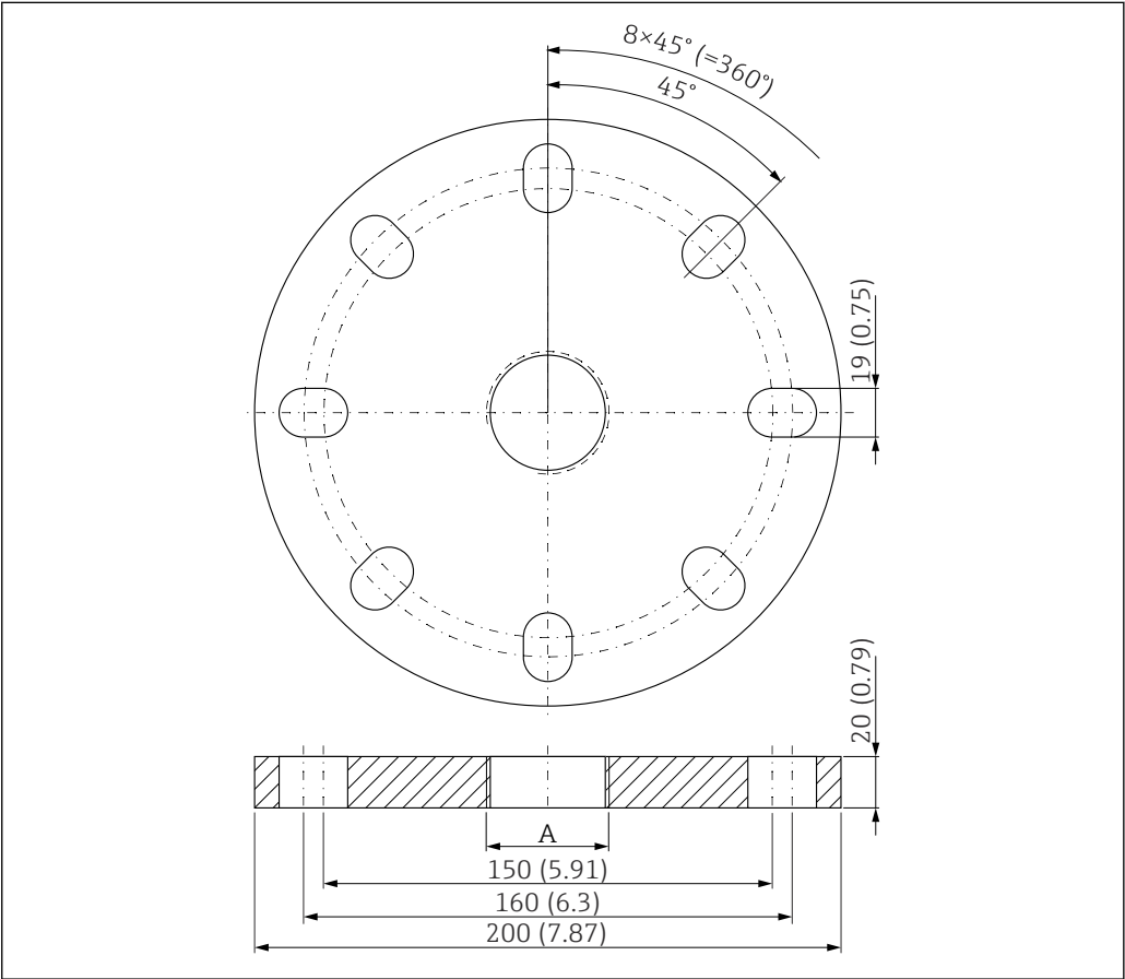
42 UNI 3"/DN80/80 法兰的外形尺寸; 单位: mm (in)
