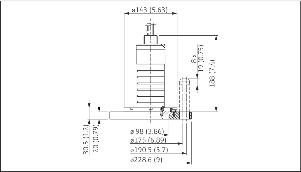
29 80 mm (3 in)口径天线的外形尺寸，安装有 4"/DN100 松套法兰；单位：mm (in)
