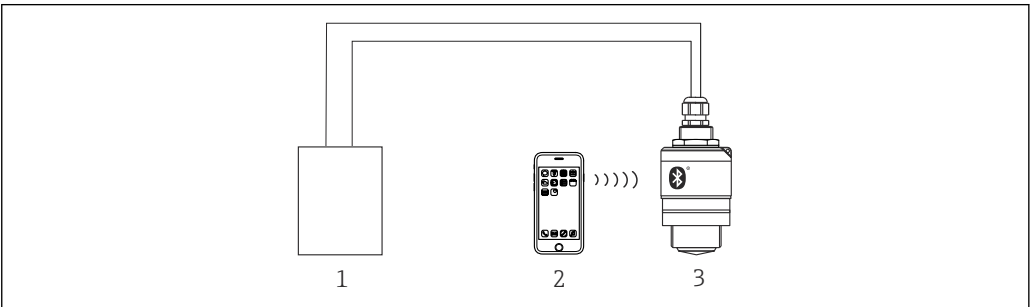
图 33 通过 Bluetooth®蓝牙无线技术实现远程操作
