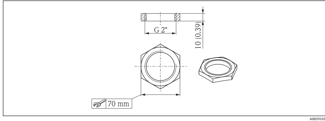
图 37 锁紧螺母的外形尺寸；单位：mm (in)
