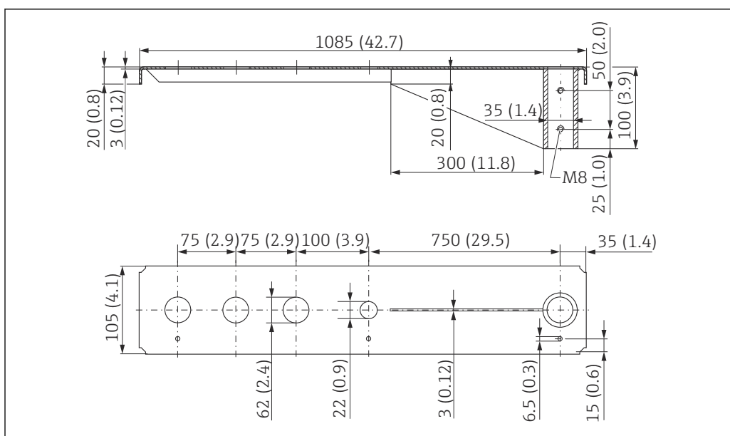
52 安装在 G 2" 传感器顶部过程连接上的旋转悬臂 (长) 的外形尺寸。测量单位 mm (in)
