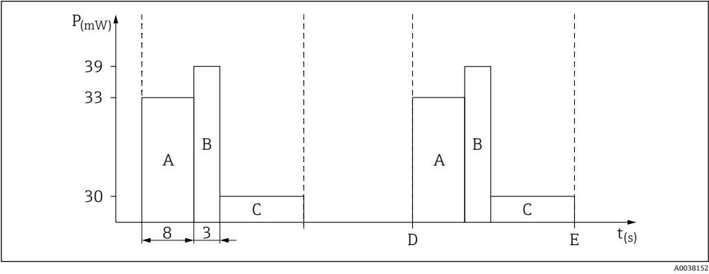
图 3 通过 RTU 启动或结束单次采样模式时的功耗
