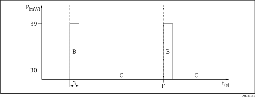
图 4 始终开启单次采样模式时的功耗
