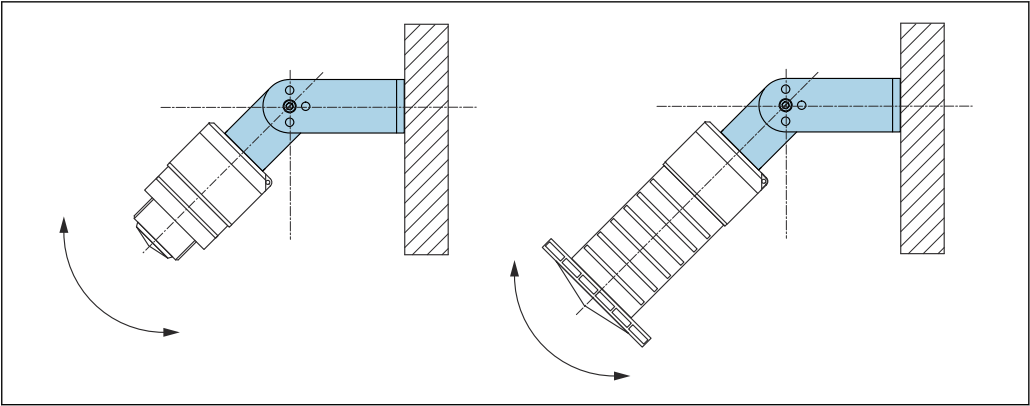
图 18 使用墙装架安装（可调节）
