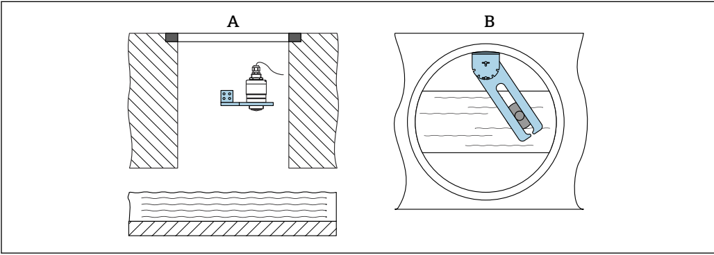
图 21 安装在水井中（可旋转、可调节） A 使用悬臂和墙装架安装 B 悬臂（可旋转、可调节）（例如在水渠正上方定位设备）
