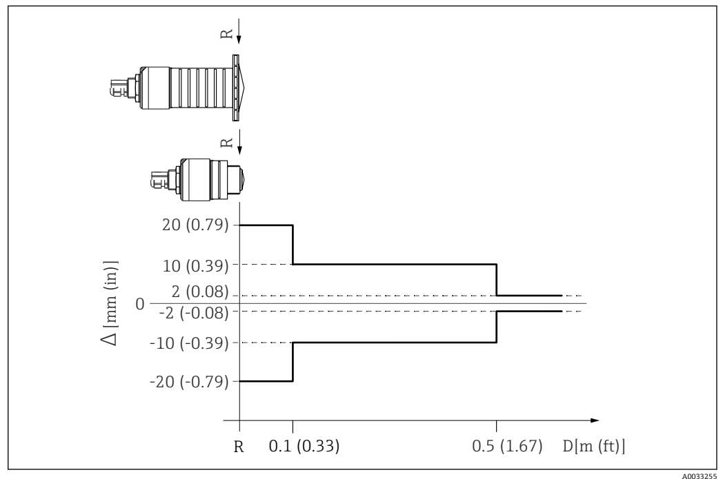
9 近距离测量时的最大测量误差 (以标准型仪表为例)
