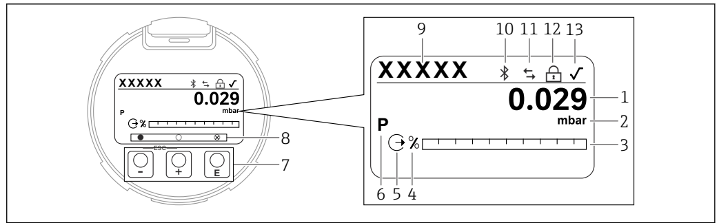
4 Grafische Anzeige mit optischen Bedientasten.
