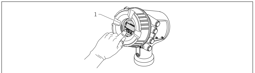
图 17 Micropilot NMR81、NMR84 的现场操作
