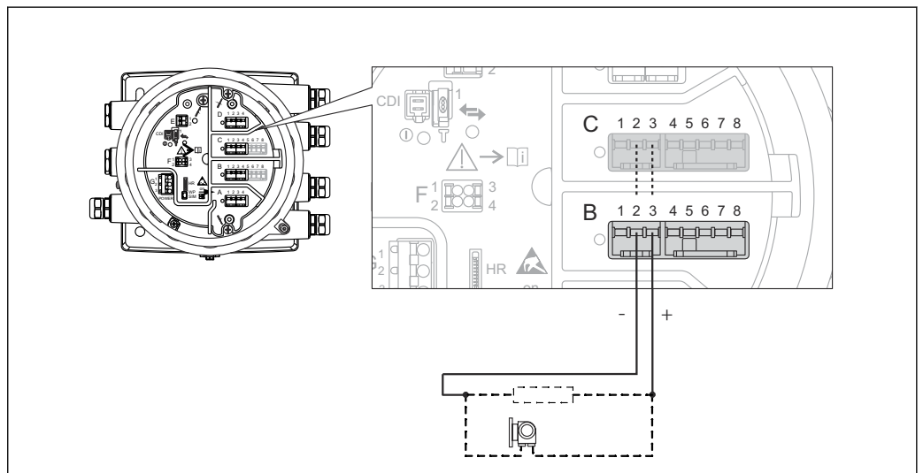
8 有源输入或有源输出：使用接线端子 2 和 3
