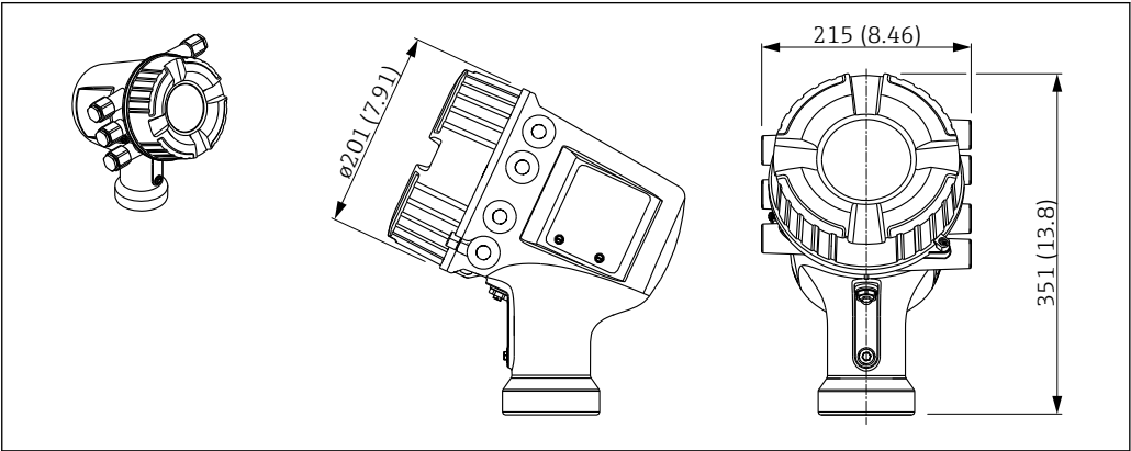
13 电子腔外壳的外形尺寸示意图；单位：mm (in)；图中未标识电缆入口的转接头。
