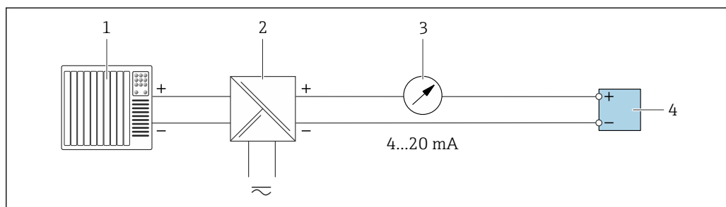
20 Przykład podłączenia dla wyjścia prądowego 4...20 mA (pasywnego)
