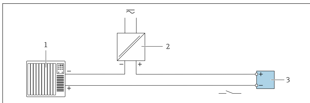
▣ 25 Przykład podłączenia dla wyjścia przekaźnikowego (pasywnego)
