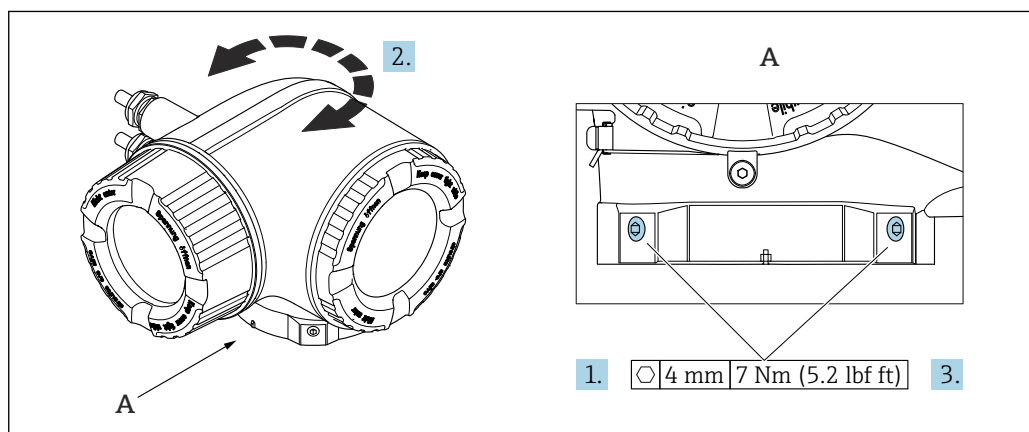
15 Wersja obudowy do stref zagrożonych wybuchem
