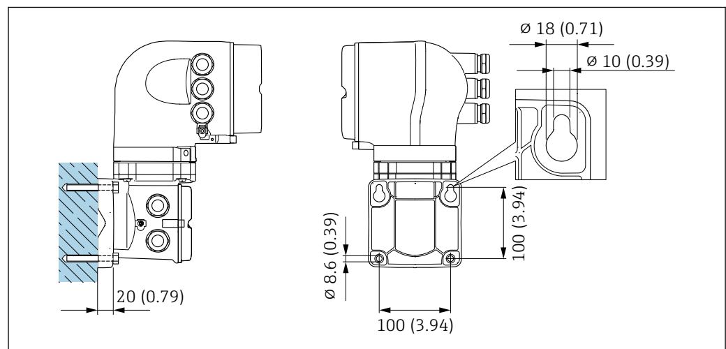
13 Jednostka: mm (cale)
