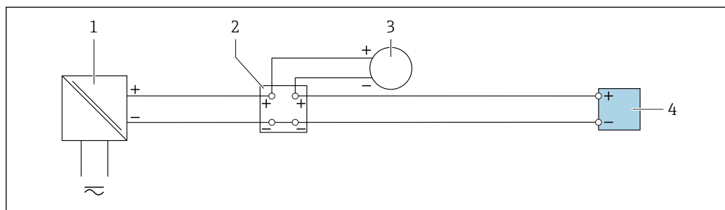
▣ 26 Przykład podłączenia dla wejścia prądowego 4...20 mA
