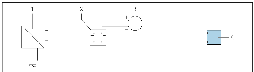
▣ 21 Przykład podłączenia dla wejścia prądowego 4...20 mA
