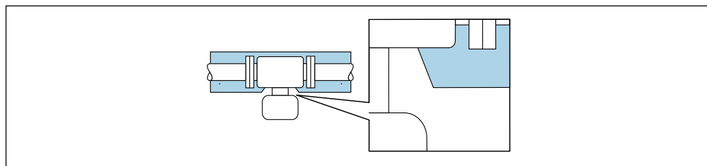
6 Izolacja termiczna rurociągu i szyjka wydłużona nieosłonięta
