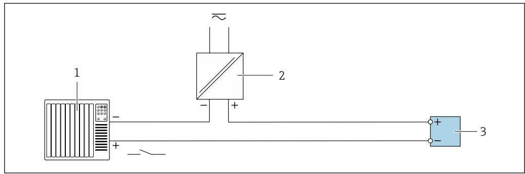
22 Przykład podłączenia dla wersji z wejściem statusu
