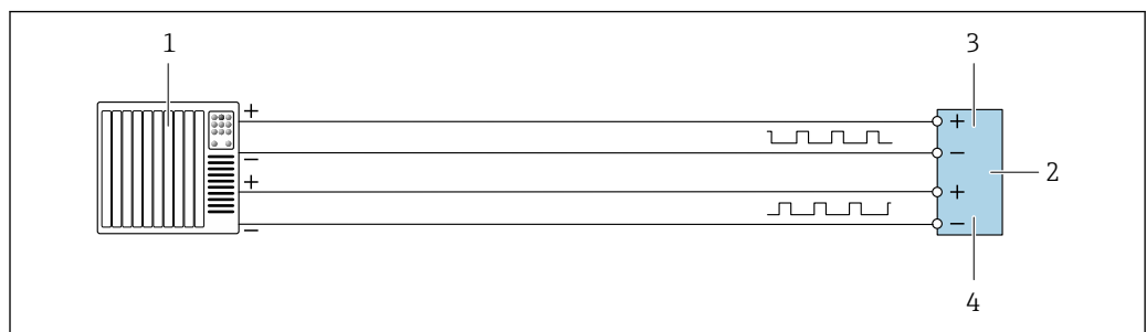
18 Przykład podłączenia dla podwójnego wyjścia impulsowego (aktywnego)
