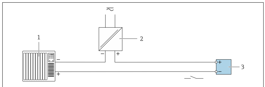
▣ 20 Przykład podłączenia dla wyjścia przekaźnikowego (pasywnego)
