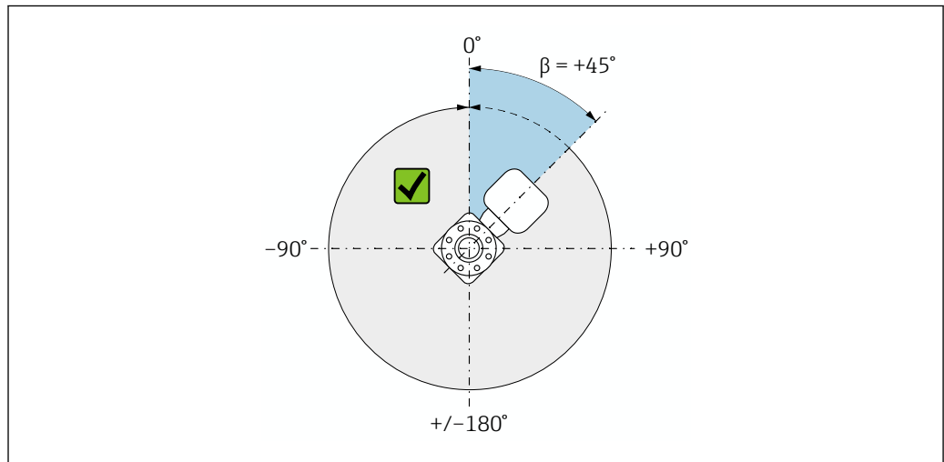
8 Widok z góry zgodnie z kierunkiem przepływu
