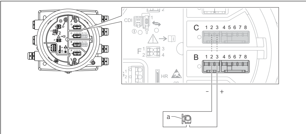
图 14 输入模式下的有源模拟量输入/输出模块
