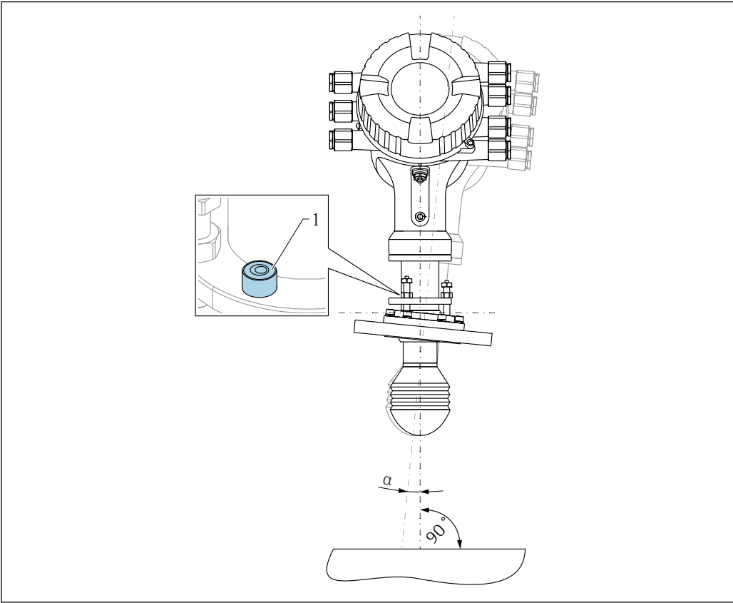
图 5 100 mm (4") 天线的天线角度调节装置
