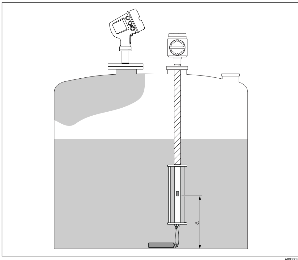
图 29 Prothermo NMT53x: 罐底测温元件位置
