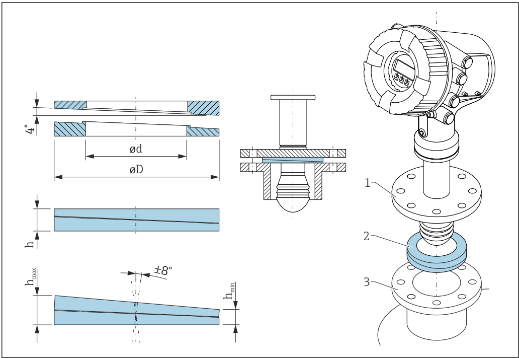
48 可调角度密封圈用于调节天线位置，角度调节范围为 \pm 8^\circ
