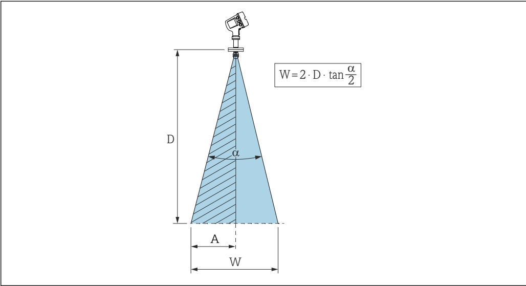
图 3 波束角 \alpha 、距离 D 和波束直径 W 的相互关系。距离 A 是距离罐壁（或其他设备）的最小距离。距离 A 为波束直径 W 的一半
