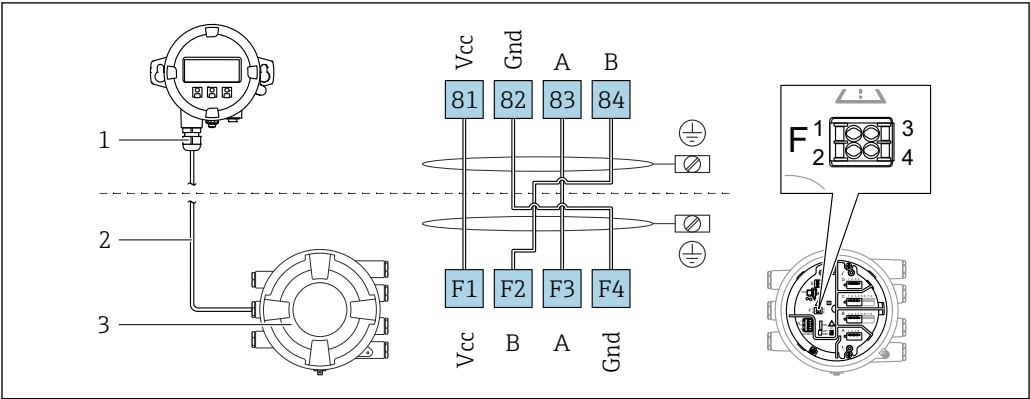
图 8 分离型显示单元与操作单元 DKX001 连接至雷达液位测量设备 (NMR8x、NMS8x 或 NRF8x) 1 分离型显示与操作单元 2 连接电缆 3 雷达液位测量设备 (NMR8x、NMS8x 或 NRF8x)
