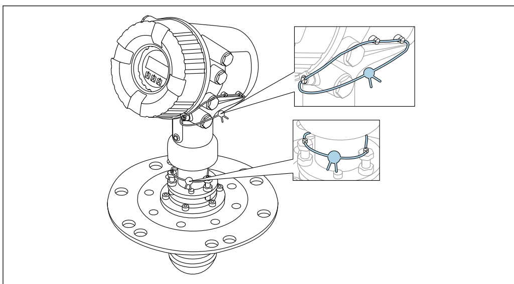
图 23 密封接线腔盖板（顶部）和调节装置（底部）
