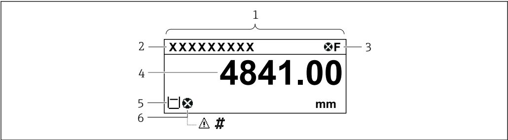
图 18 典型的标准显示界面（测量值显示）
