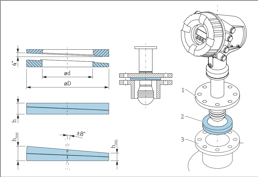
图 4 可调角度密封圈用于调节天线位置，角度调节范围为±8°
