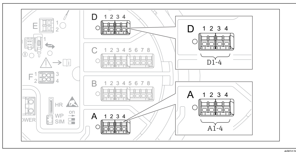
图 9 “Modbus”模块、“V1”模块或“WM550”模块的名称（实例）：这些模块可能位于插槽 B 或 C 中，与设备具体型号相关。
