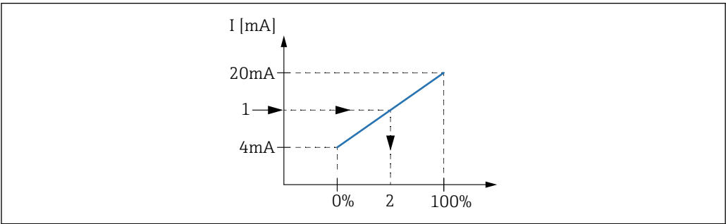
图 32 按 4...20 mA 输入调整过程变量
