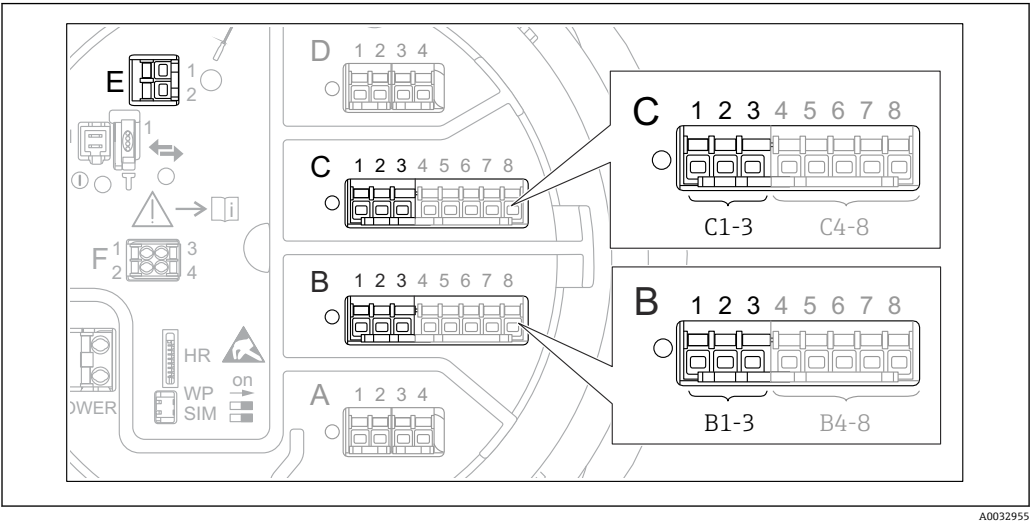
图 28 HART 回路的可能接线端子 B 插槽 B 中的模拟量输入/输出模块 (与设备具体型号相关→ 图 21) C 插槽 C 中的模拟量输入/输出模块 (与设备具体型号相关→ 图 21) E HART Ex is 输出 (所有设备型号均提供)
