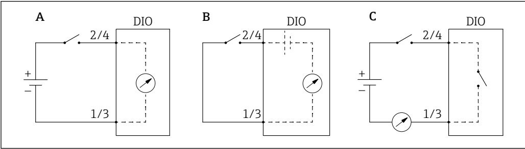
图 52 数字量输入/输出模块的工作模式
