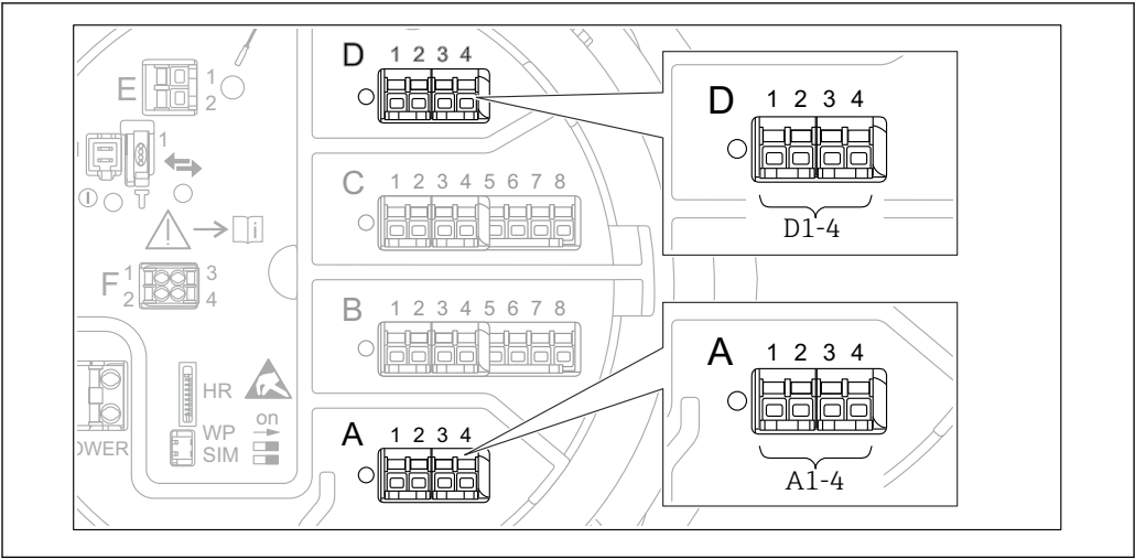
图 41 Modbus 模块的可能安装位置示例；取决于设备型号，上述模块可以安装在插槽 B 或 C 中→ 21。
