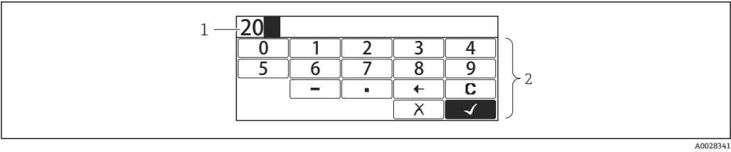
图 21 显示单元上的数字编辑器
