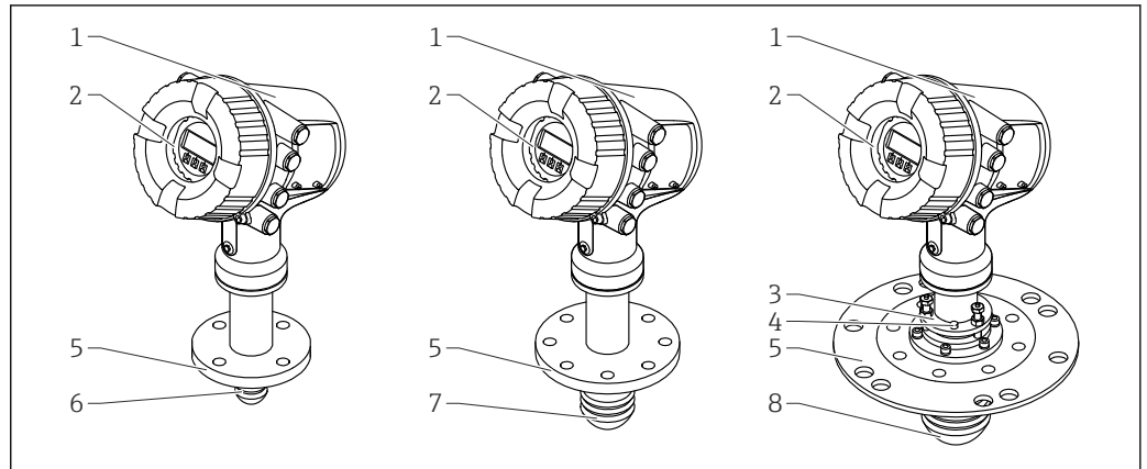
图 1 Micropilot NMR81 的结构示意图
