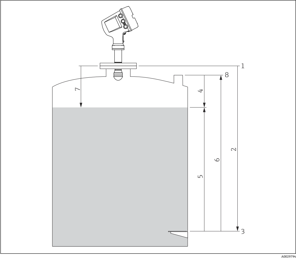
图 27 雷达罐体测量术语
