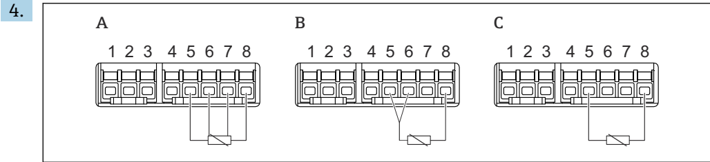
图 34 热电阻连接方式
