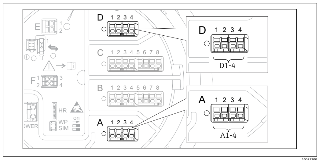
图 43 WM550 模块的可能安装位置（实例）；取决于设备型号，上述模块还可以安装在插槽 B 或 C 中 → 图 21。
