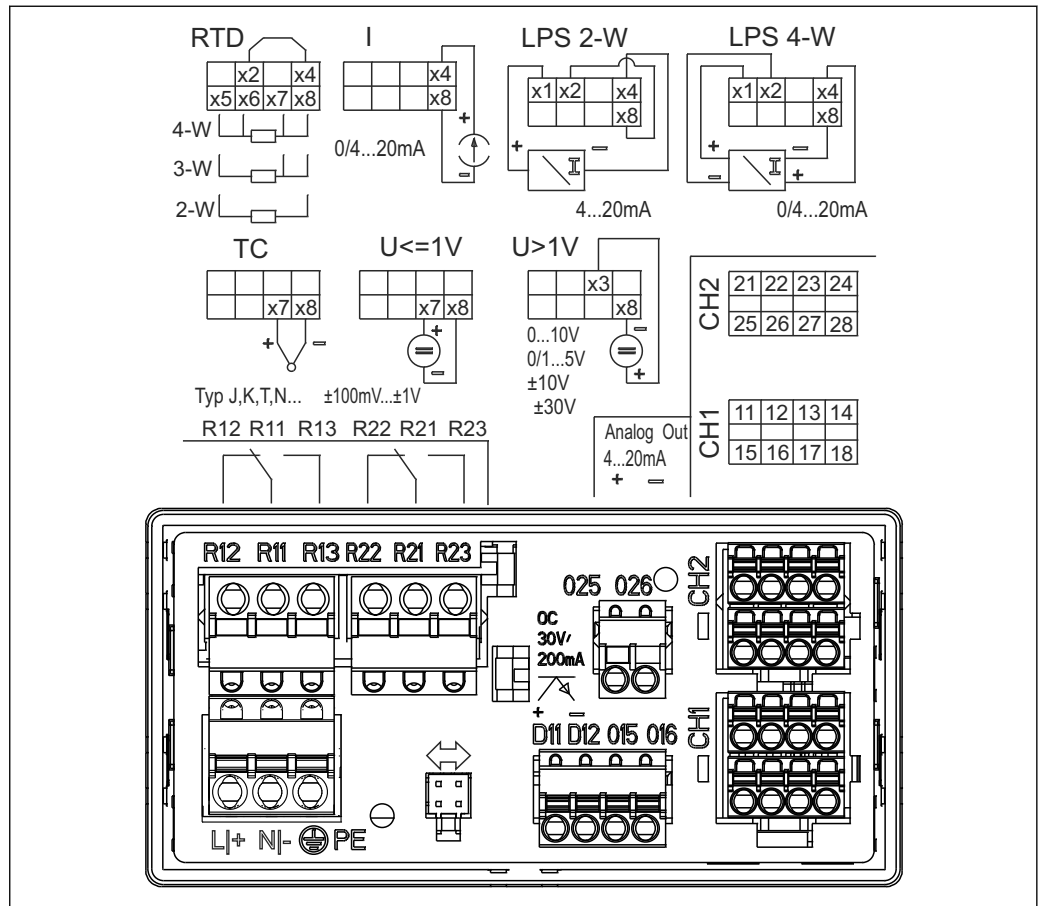
图 13 过程显示仪的接线端子分配 (继电器 (接线端子 Rx1...Rx3) 和通道 2 (接线端子 21...28 和 025/026), 可选); 注: 图示为发生电源故障时的继电器触点位置。
