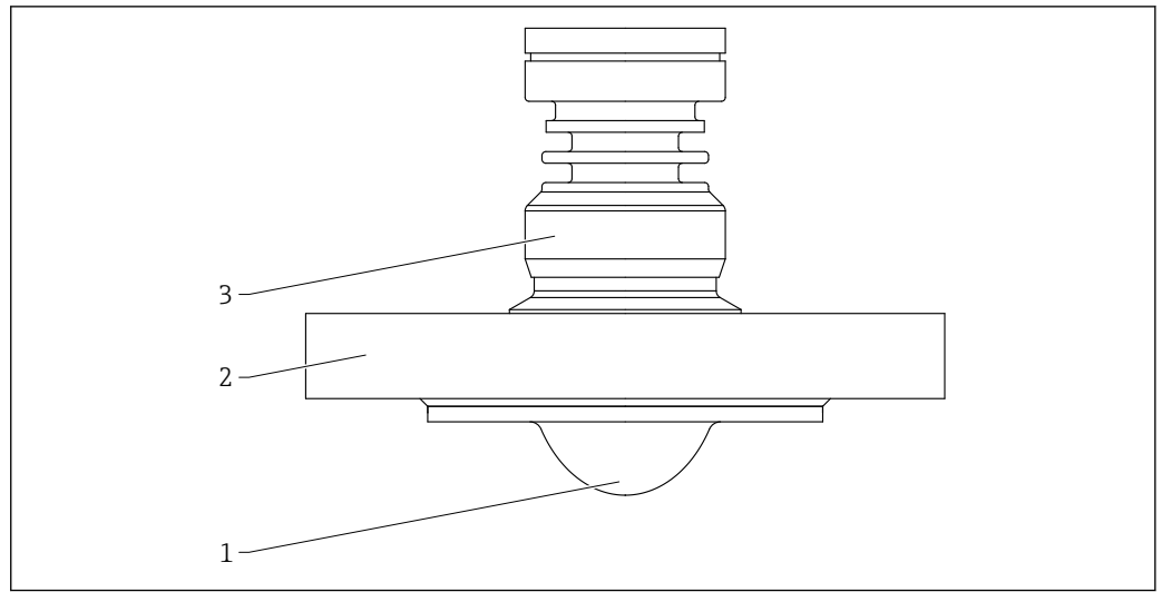
■ 62 Material; antena de montaje enrasado con revestimiento de PTFE, 50 mm (2 in), con brida
