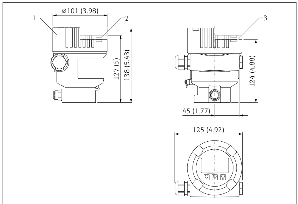
52 Medidas de la caja de aluminio de compartimento único. Unidad de medida mm (in)
