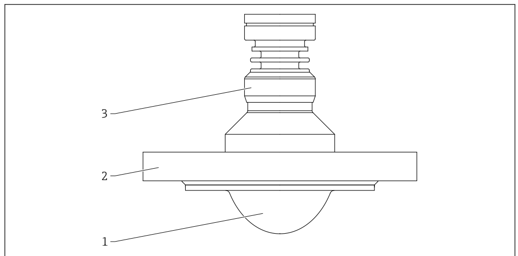
■ 63 Material; antena, montaje enrasado con revestimiento, PTFE, 80 mm (3 in), con brida
