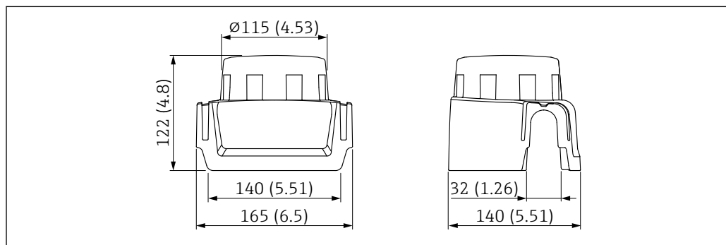
67 Medidas. Unidad de medida mm (in)
