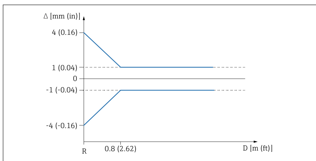
7 Error medido máximo en aplicaciones de rango cercano
