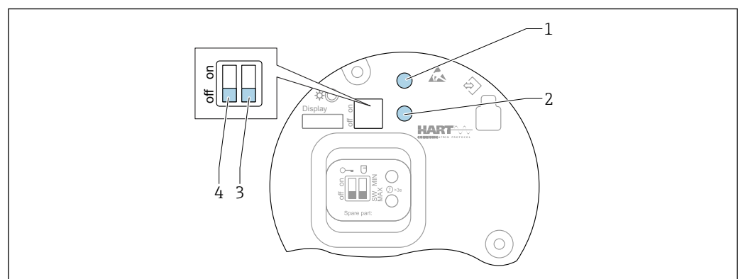
64 Teclas de configuración y microinterruptores en el módulo del sistema electrónico HART
