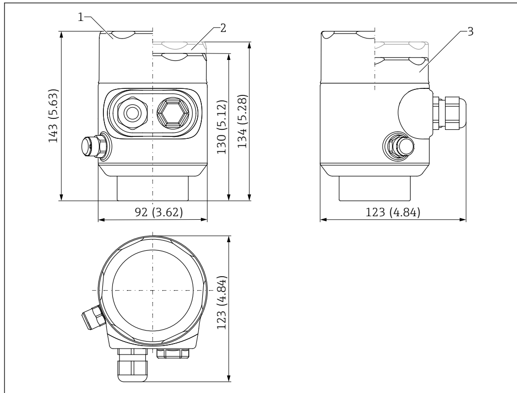
■ 53 Medidas de la caja de compartimento único, 316L, higiene. Unidad de medida mm (in)
