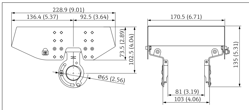
66 Medidas. Unidad de medida mm (in)
