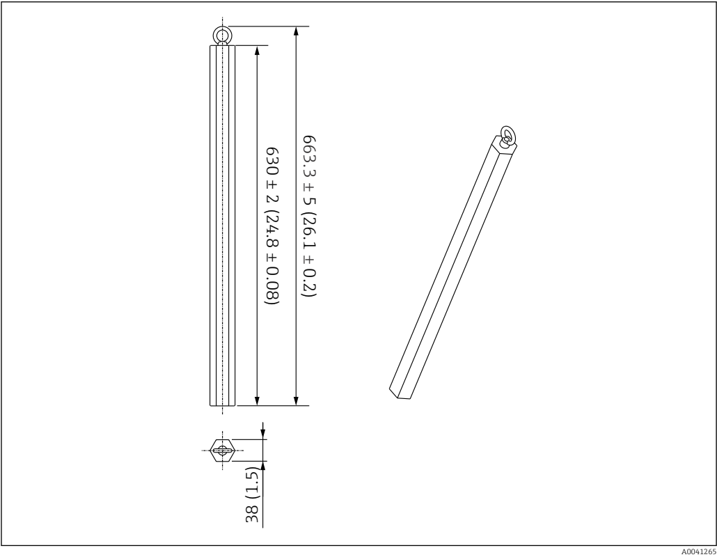
40 Accesorio de instalación. Unidad de medida mm (in)
