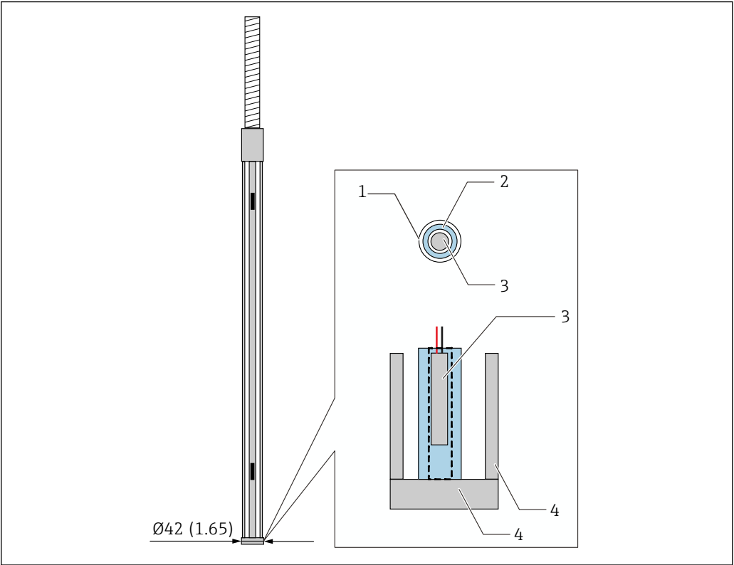
31 Diseño de la sonda de fondo de agua. Unidad de medida mm (in)
