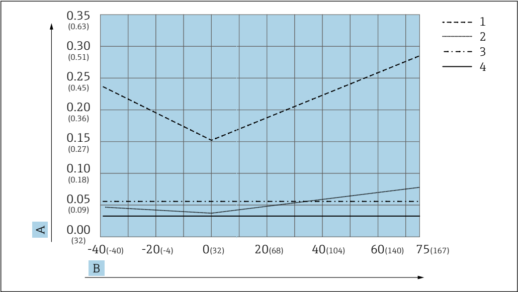
10 Precisión total, rangos de temperatura estándar, unidad de temperatura grado °C (°F)
