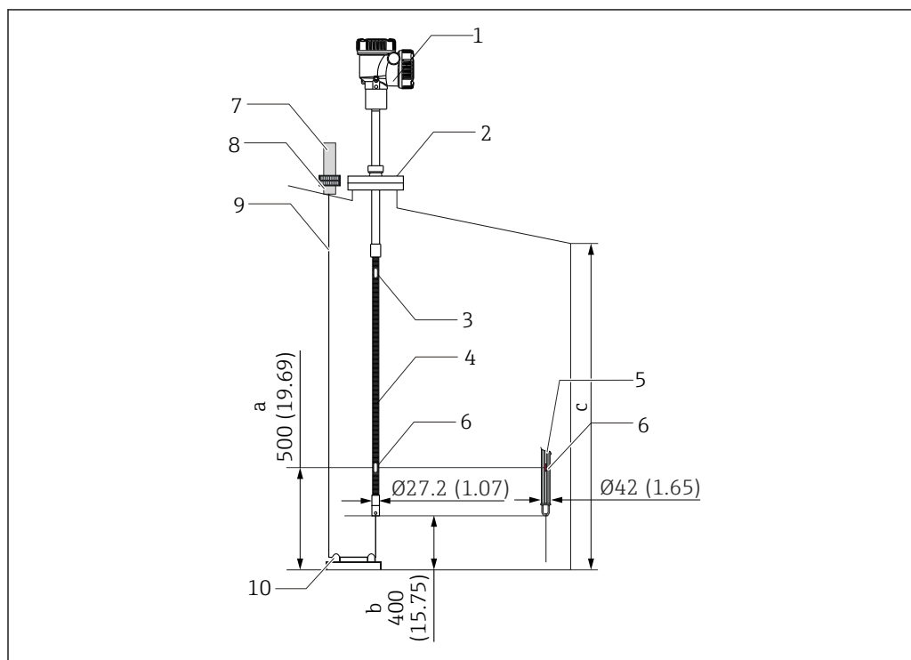
■ 18 Método de anclaje superior. Unidad de medida mm (in)
