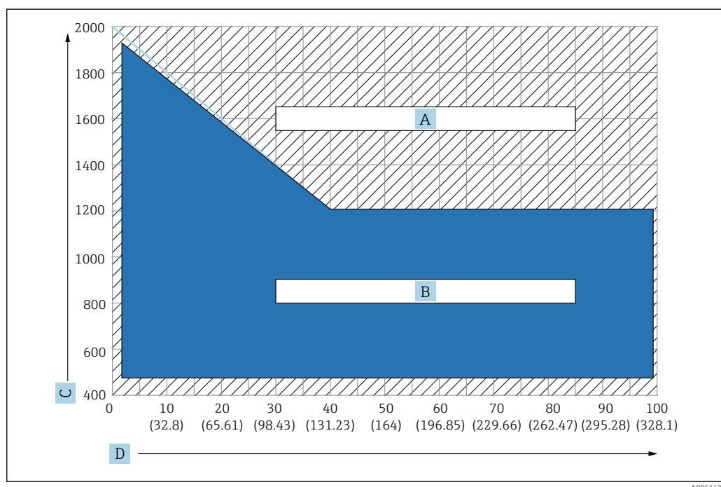
41 Gráfico de selección del contrapeso de anclaje, C: unidad de densidad [kg/m 3 ], D: unidad de longitud m/(ft)
