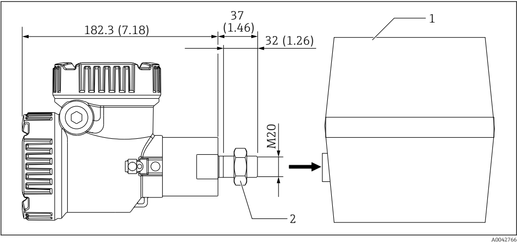
28 Opción 2: convertidor (Varec 1700, conexión roscada M20). Unidad de medida mm (in)
