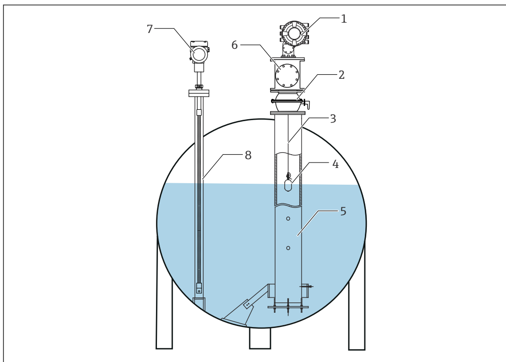
24 Termopozo para un depósito presurizado
