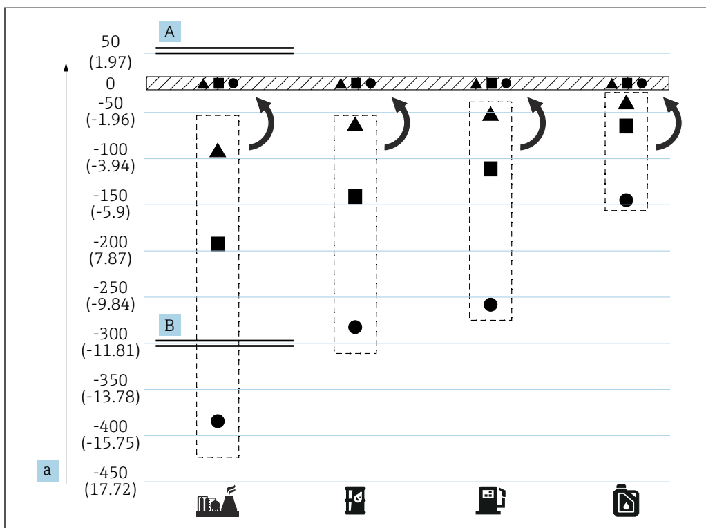
33 Efecto de la compensación de tres capas
