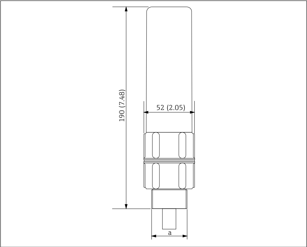
43 Medidas del anclaje superior. Unidad de medida mm (in)
