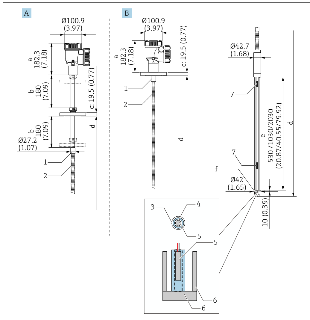
30 Convertidor + sonda de temperatura + sonda de fondo de agua
