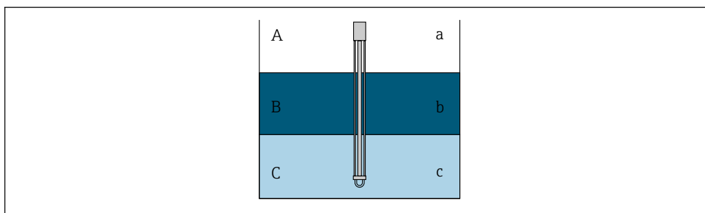
32 Medición de nivel de agua en tres capas
