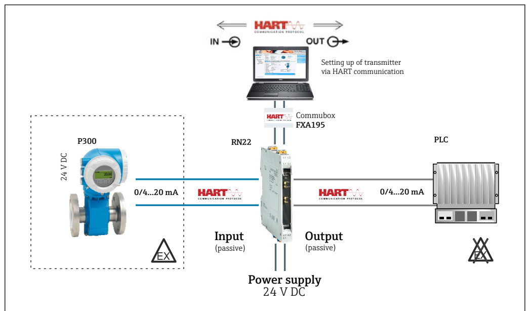
18 使用 RN22 有源安全栅进行防爆危险区流量测量
