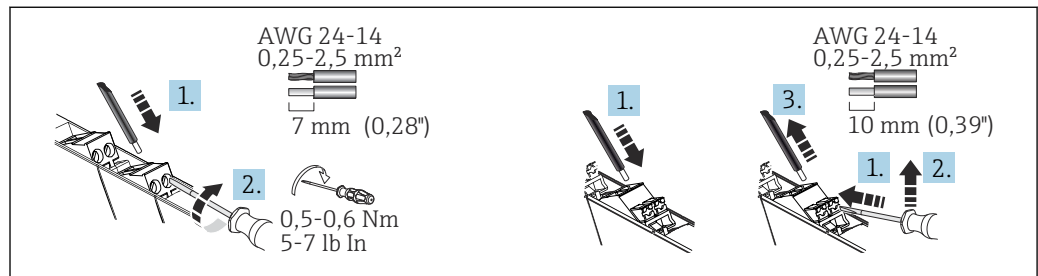
图 9 螺纹式接线端子 (左) 和直推式接线端子 (右) 电气连接图
