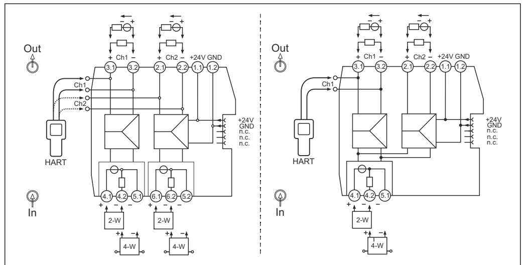
图 6 接线端子分配：单通道型和双通道型 (左图)，信号倍增器 (右图)
