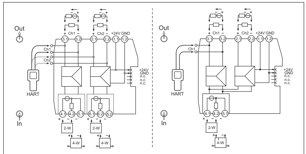
图 8 接线端子分配：单通道型和双通道型（左图），信号倍增器（右图）
