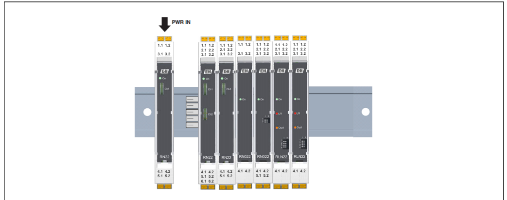
图 12 通过组内任意一件设备直接馈电
