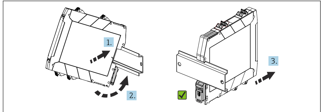
图 3 DIN 导轨上安装的设备
