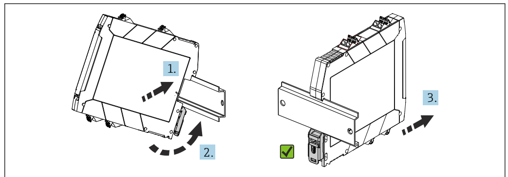
图 10 DIN 导轨上安装的设备
