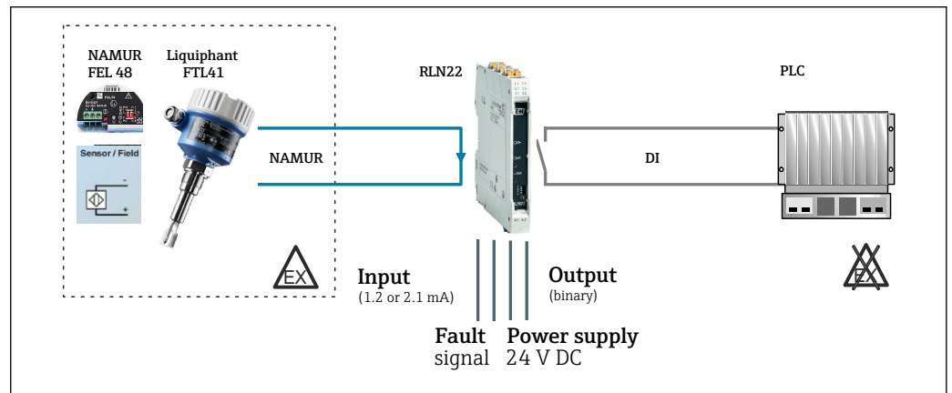
图 20 NAMUR 限定值检测，Liquiphant FTL41 配备了 FEL48 NAMUR 评估单元（用于防爆危险区）
