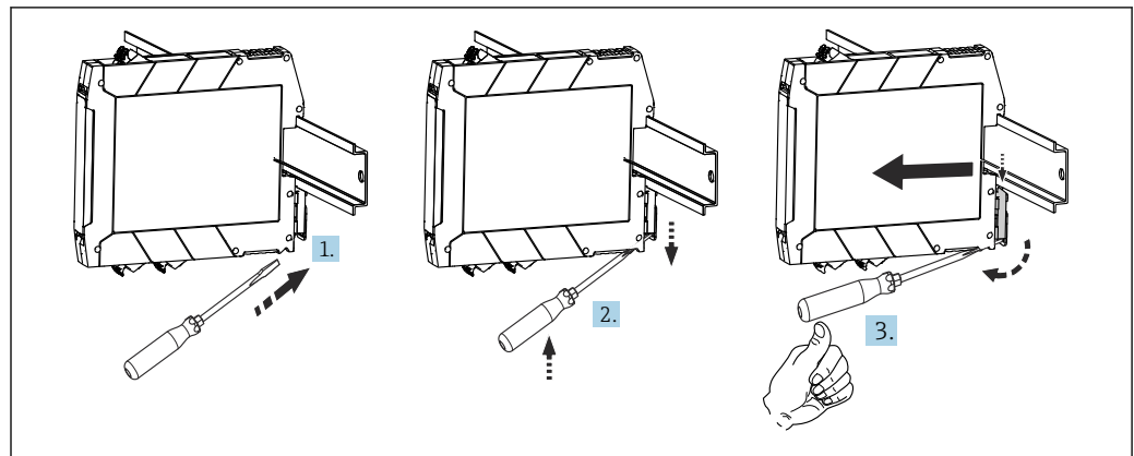
图 4 拆卸 DIN 导轨盘装型设备
