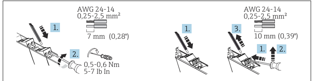
图 5 螺纹式接线端子 (左) 和直推式接线端子 (右) 的电气连接操作
