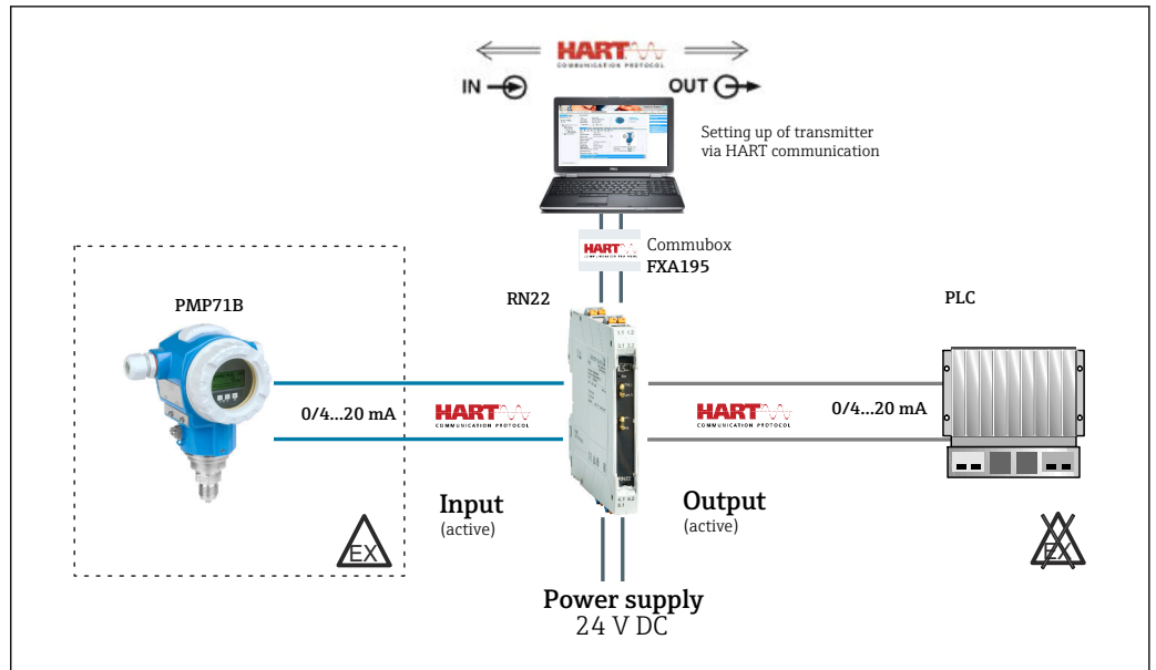
17 使用 RN22 有源安全栅进行防爆危险区压力测量
