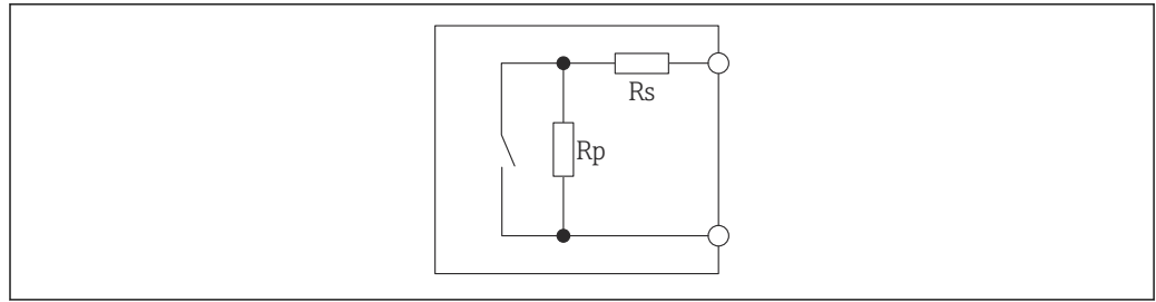
图 22 电阻性电路，用于监测线路状态（短路和断路）
