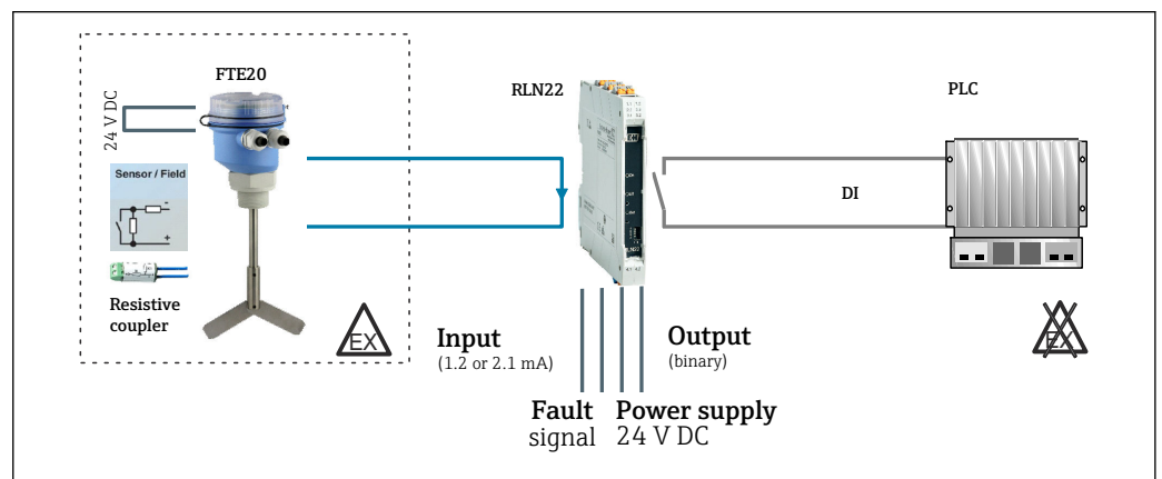
图 21 NAMUR 限定值检测，带 FTE20 阻旋式物位开关，用于监测防爆危险区线路状态
