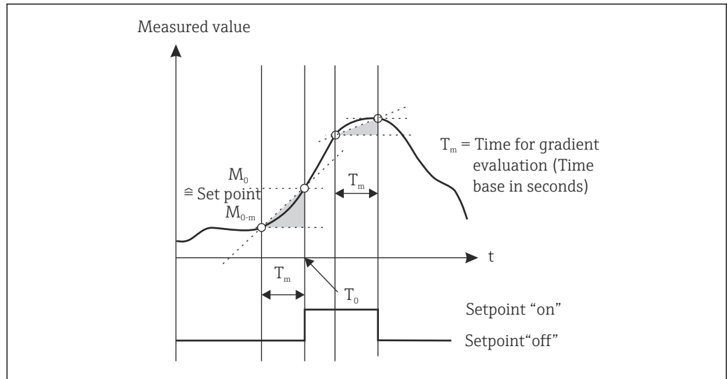
9 Режим работы Gradient
