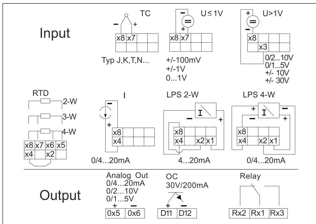
15 Назначение клемм преобразователя процесса (реле (клеммы Rx1–Rx3) и канал 2 (клеммы 21–28 и O25/O26), опционально). Примечание. Изображено положение контактов реле при нарушении предельного значения или сбое питания
