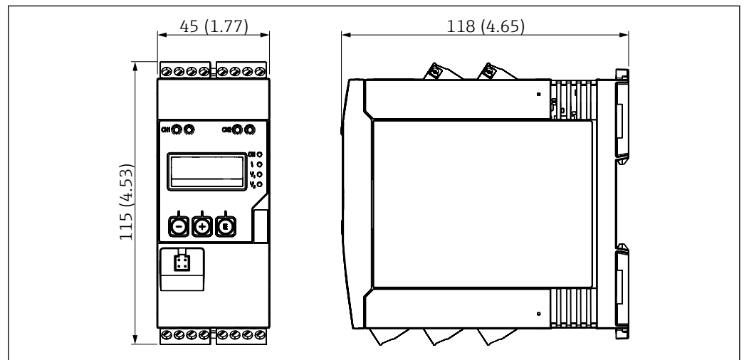
1 Размеры преобразователя процесса в мм (дюймах)
