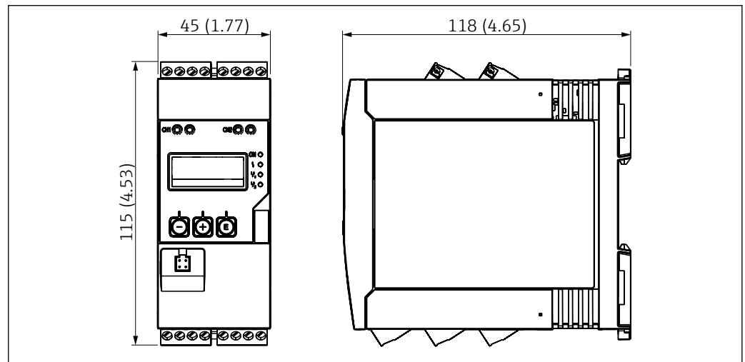
16 Размеры преобразователя процесса в мм (дюймах)
