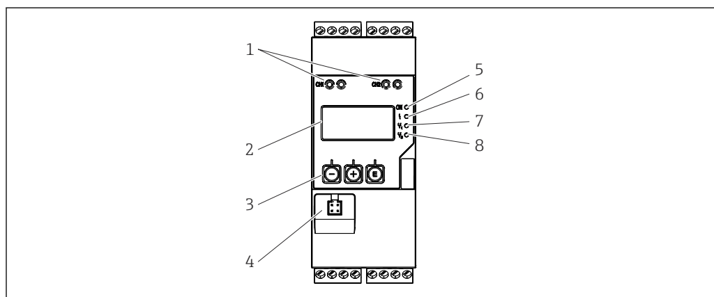
■ 17 Дисплей и элементы управления преобразователя процесса
