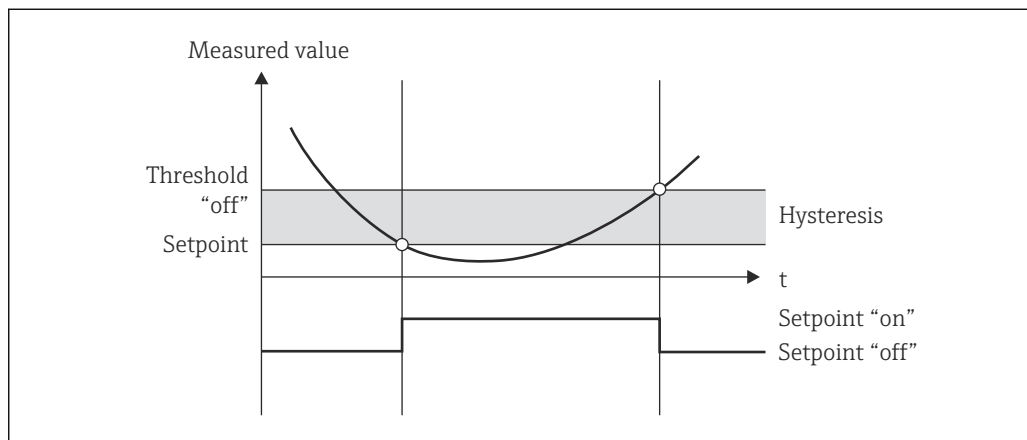
7 Режим работы Min
