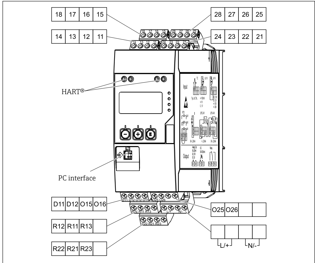
2 Назначение клемм преобразователя процесса (канал 2 и реле являются опциональными)
