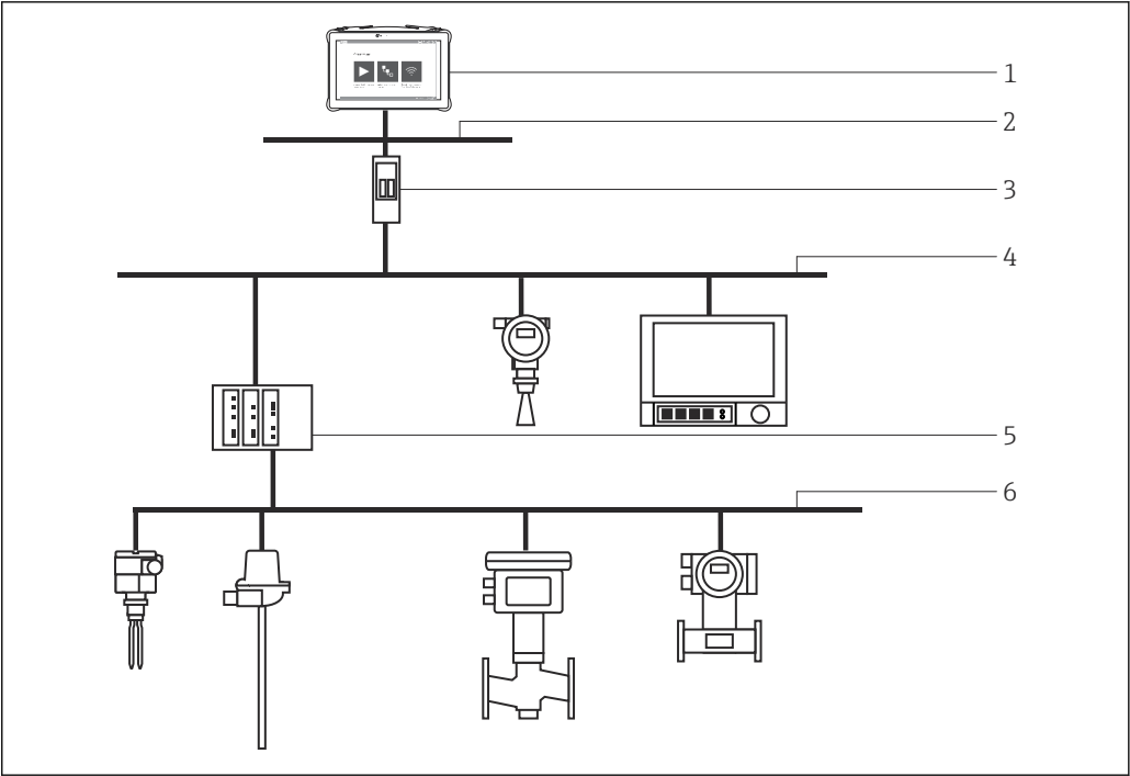
图 6 通过 Fieldgate SFG500 建立 PROFIBUS 点到总线连接
