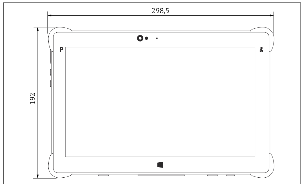
图 10 正视图
