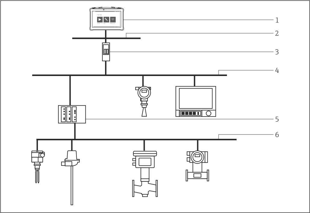
6 PROFIBUS-Punkt-zu-Bus-Verbindung über Fieldgate SFG500
