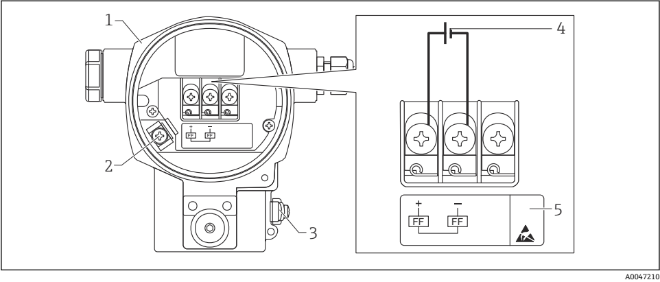
1 FOUNDATION Fieldbus 型设备电气连接示意图
