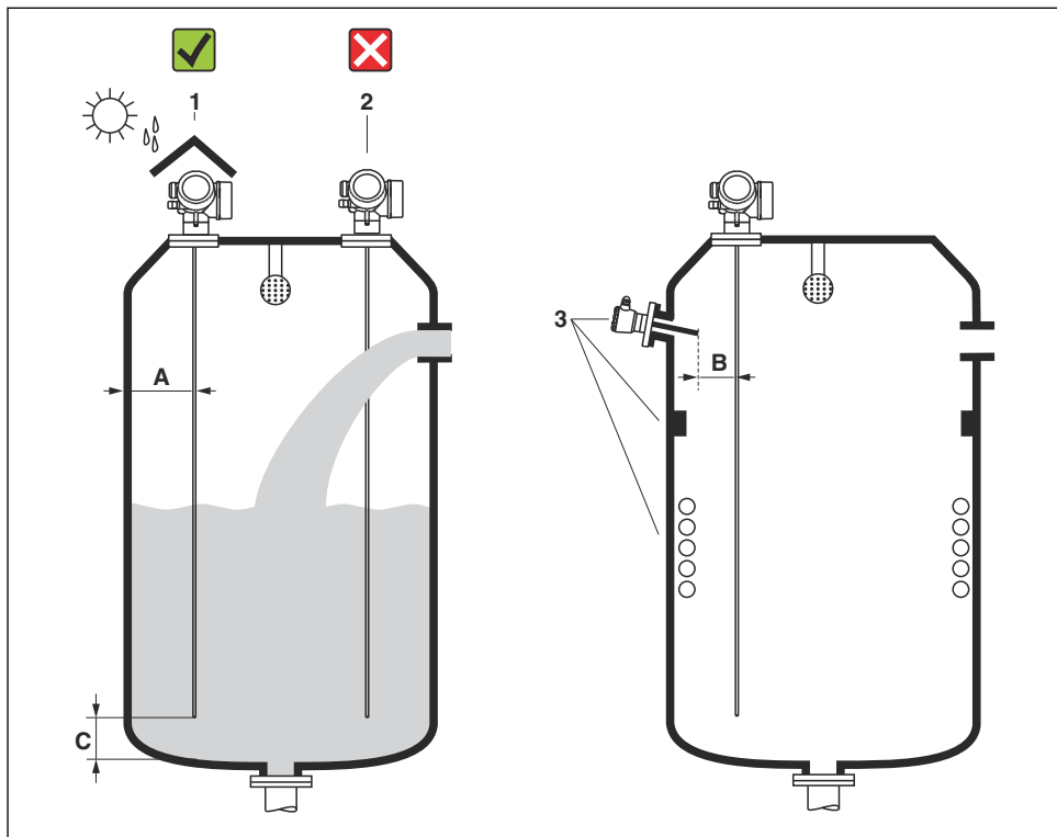
图 1 Levelflex 的安装条件
