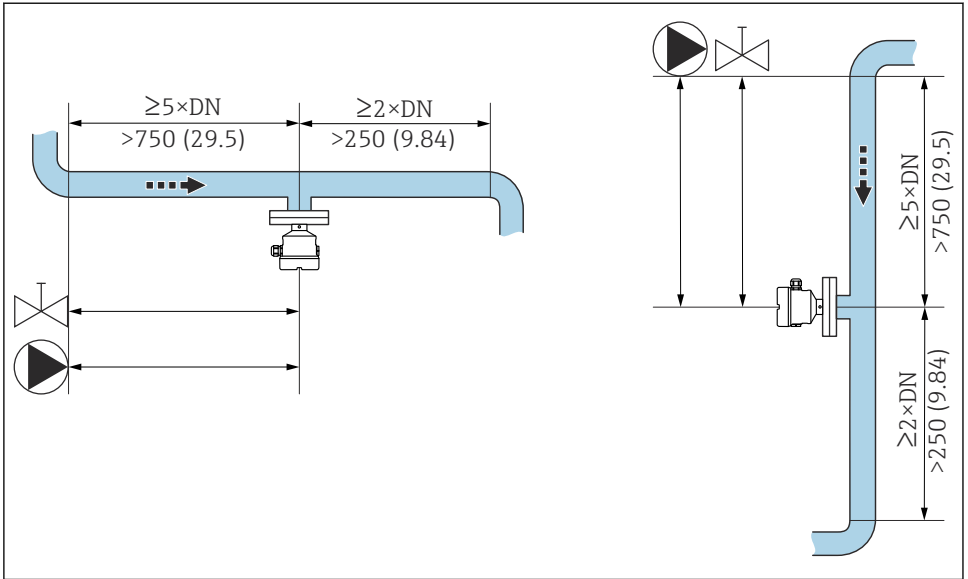
图 4 前直管段的安装。测量单位 mm (in)
