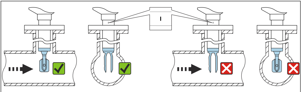
图 9 安装在管道中（注意叉体安装位置和标记）
