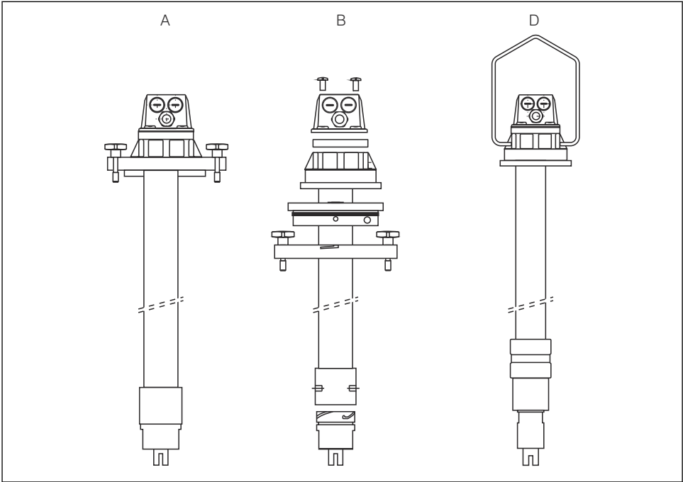
3 安装在浸入式安装支架中（安装方式 A、B 和 D）
