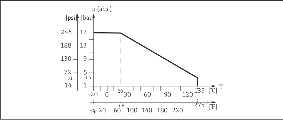
图 7 温压曲线
