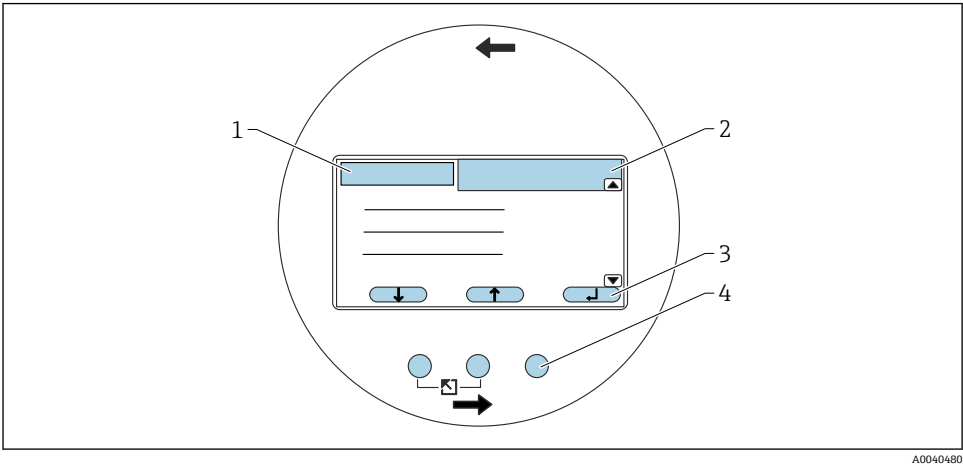
图 10 显示与操作单元
