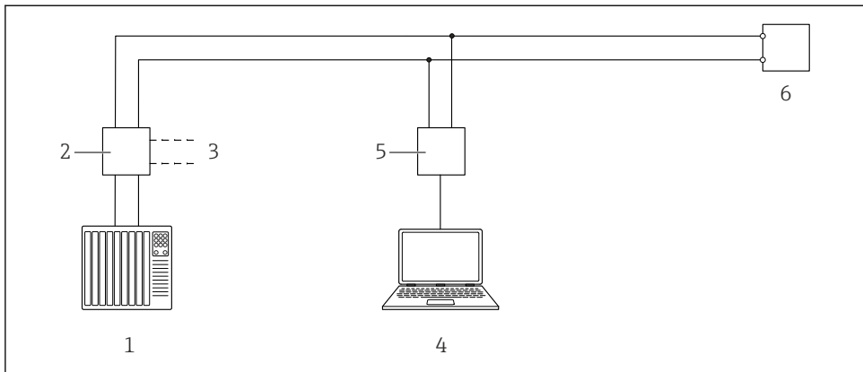
图 8 通过 HART 协议远程控制
