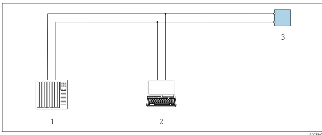
31 Opzioni per funzionamento a distanza mediante protocollo Modbus RS485 (attivo)
