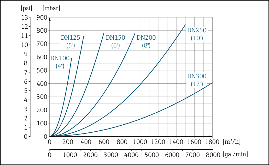
45 Perdita di carico DN 100 ... 300 (4 ... 12") per codice d'ordine per "Design", opzione C "Flangia fissa, tubo di misura ristretto, tratti in entrata/uscita 0 x DN"
