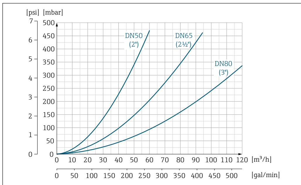
44 Perdita di carico DN 50 ... 80 (2 ... 3") per codice d'ordine per "Design", opzione C "Flangia fissa, tubo di misura ristretto, tratti in entrata/uscita 0 x DN"
