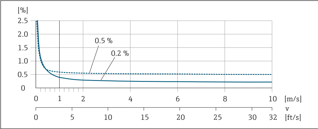
40 Errore di misura massimo in % v.i.
