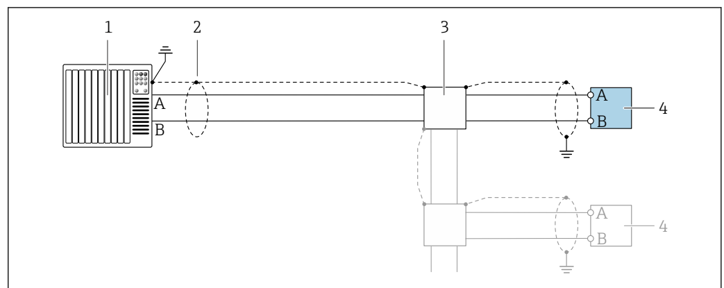
17 Esempio di connessione per Modbus RS485, area sicura e Zona 2/Div. 2
