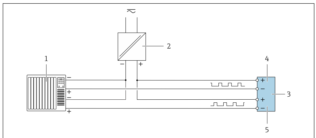
23 Esempio di connessione per doppia uscita impulsiva (passiva)
