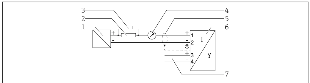
図 12 ブロック図、2線式：4~20 mA HART、スイッチ出力
