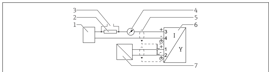
図 16 ブロック図、4線式：4~20 mA HART（10.4~48 V DC ）
