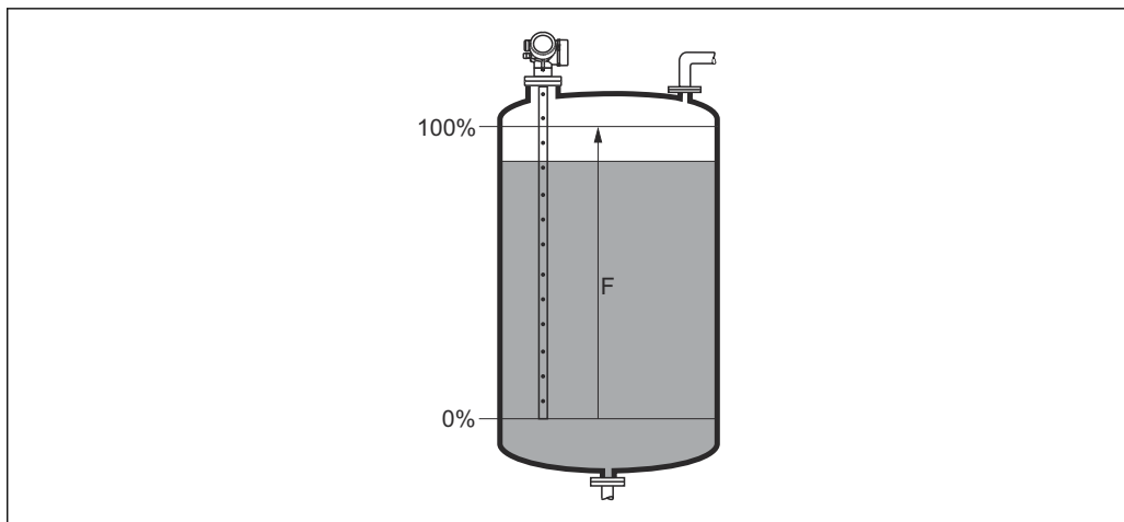
図 43 液体レベル測定用の満量校正 (F)
