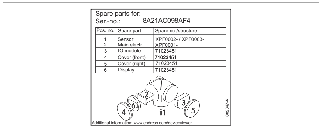
☞ 37 端子接続部カバーのスペアパーツ銘板の例
