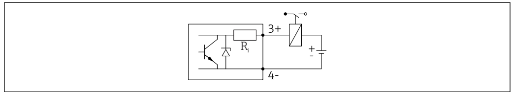
図 19 リレーの接続
