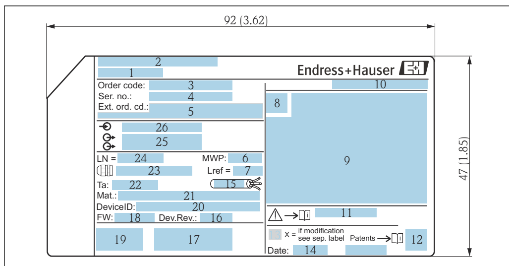
図 3 Levelflex の銘板 ; 単位 : mm (in)
