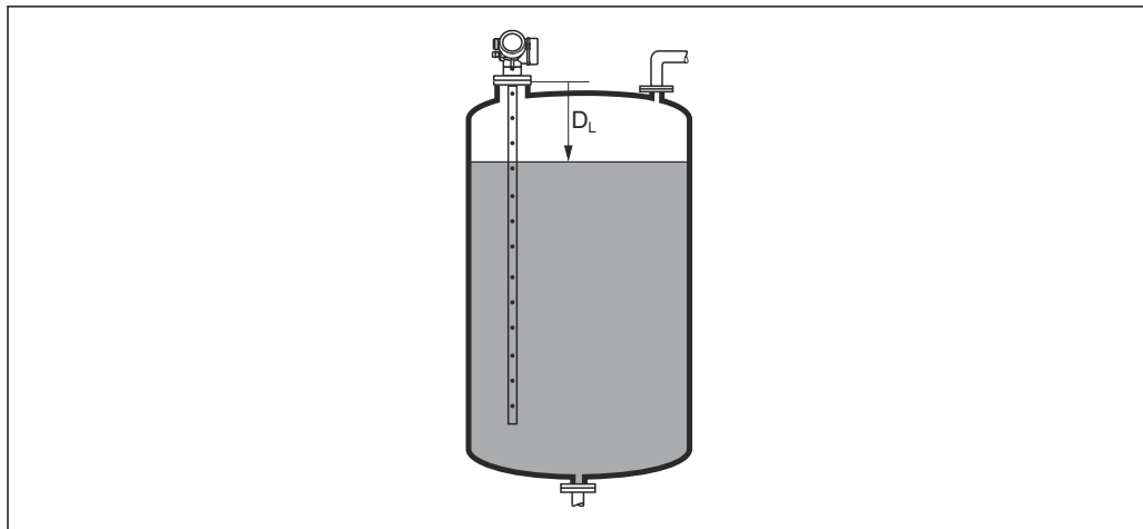
図 45 液体計測の距離
