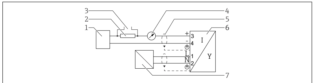
図 18 ブロック図、4 線式：4~20 mA HART (90~253 V AC )
