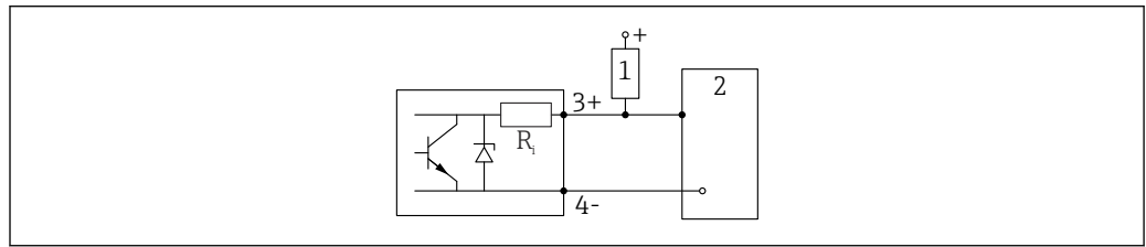
図 20 デジタル入力の接続
