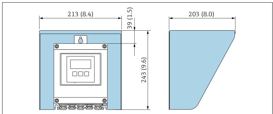
图 36 Proline 500 (数字) 变压器的防护罩的外形尺寸图; 单位: mm (in)
