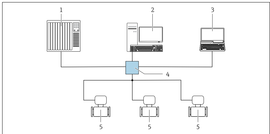
图 56 通过 EtherNet/IP 网络进行远程操作：星形拓扑结构
