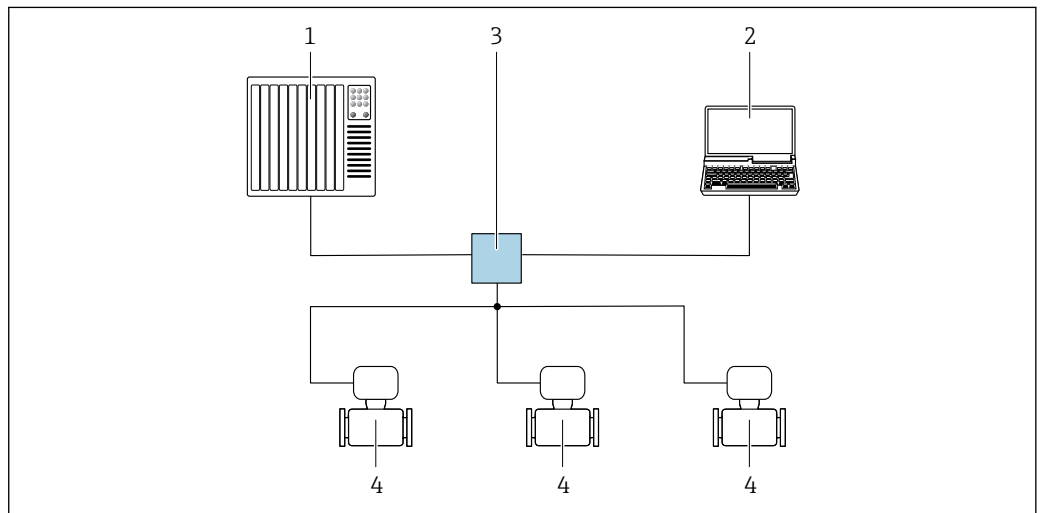
☑ 58 通过 PROFINET 网络进行远程操作：星形拓扑结构
