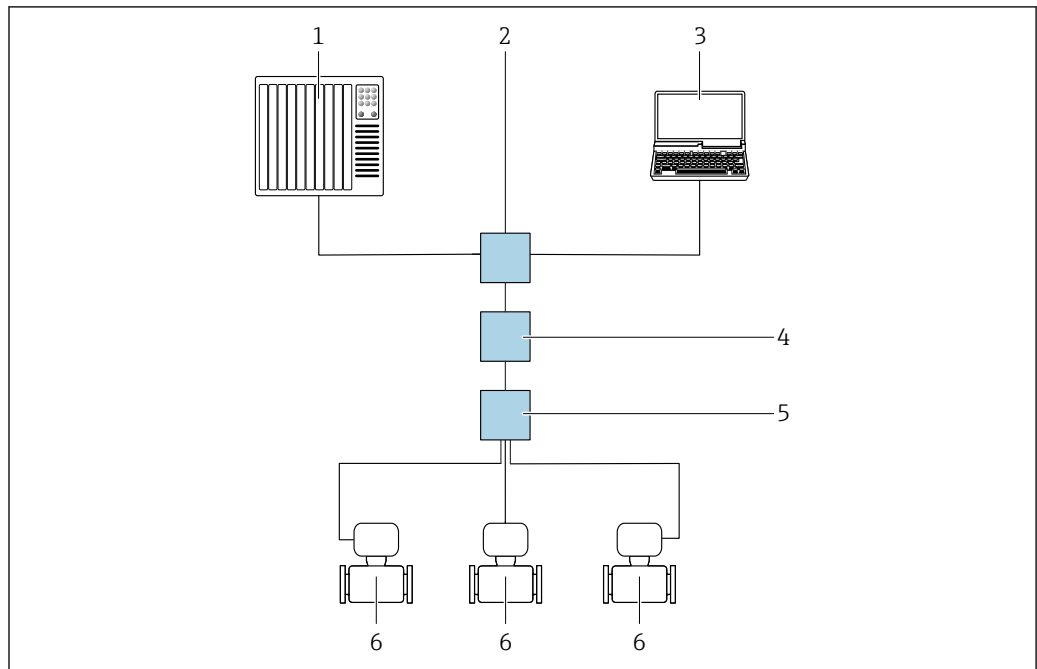
图 60 通过 APL 网络进行远程操作
