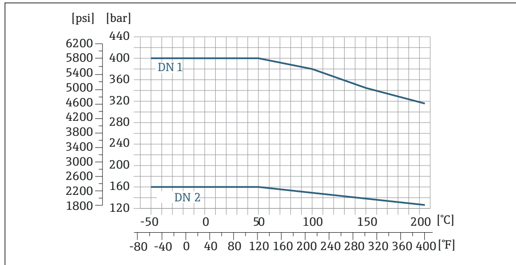
图 34 4-VCO-4 接头材质: 1.4539 (904L) ; 8-VCO-4 接头材质: 1.4539 (904L) ; NPTF 螺纹接头材质: 1.4539 (904L)
