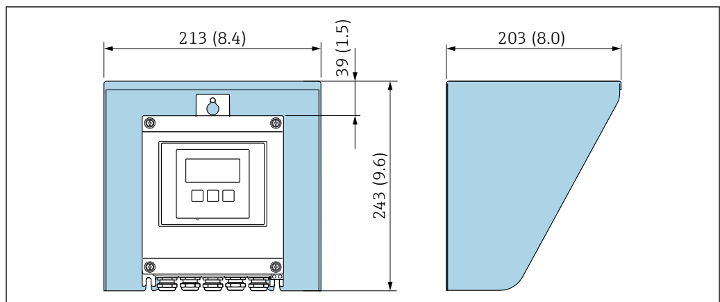
图 42 Proline 500 (数字) 变压器的防护罩的外形尺寸图; 单位: mm (in)
