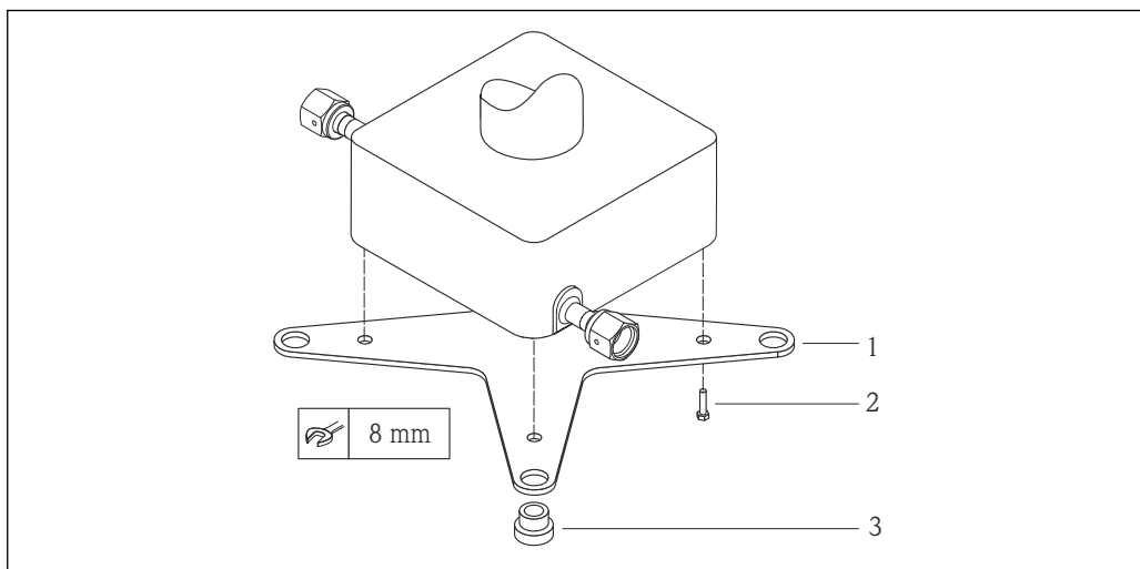
图 27 Cubemass 安装底板的安装套件示意图
