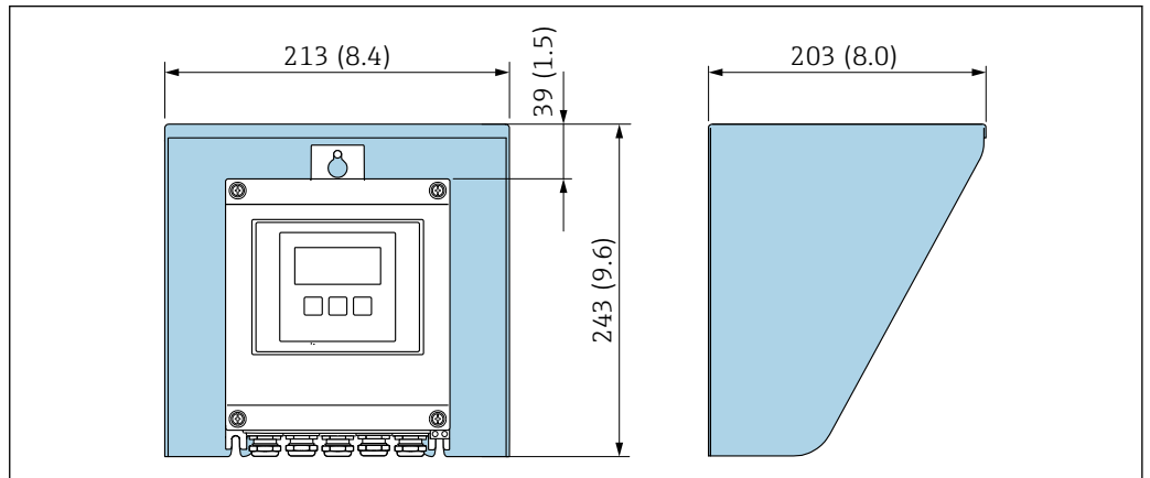
图 29 Proline 500 (数字) 变送器的防护罩的外形尺寸图; 单位: mm (in)
