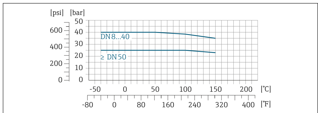
图 36 连接部件材质: 1.4404 (316/316L)
