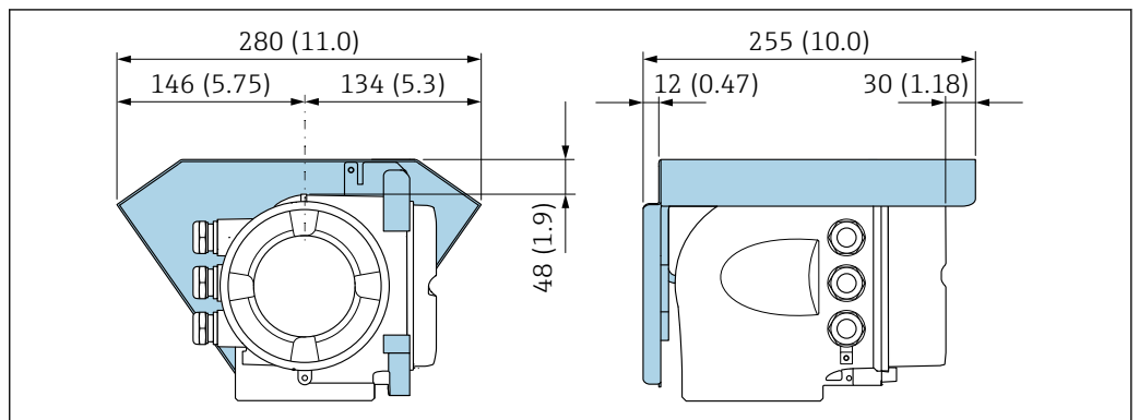
图 30 Proline 500 (模拟) 变送器的防护罩的外形尺寸图; 单位: mm (in)
