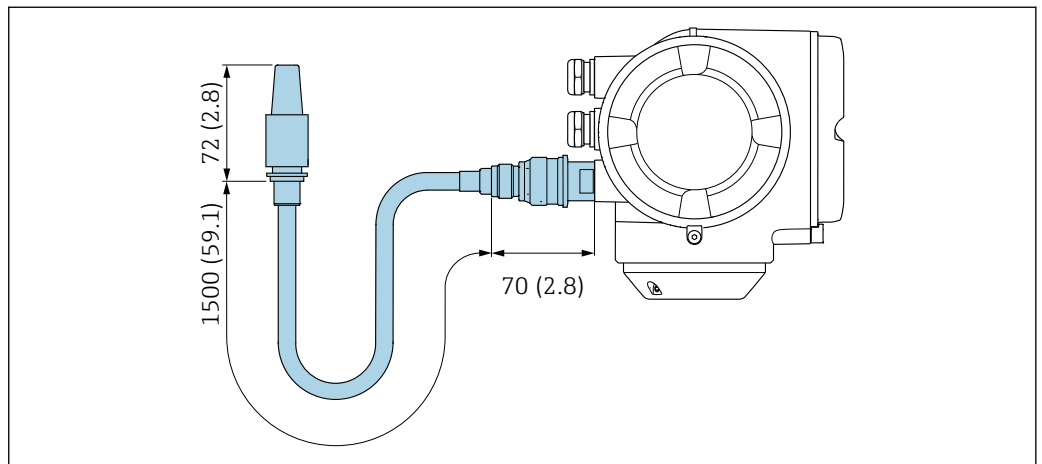
54 单位: mm (in)
