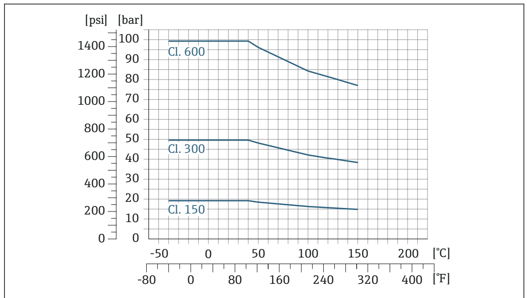
33 法兰材质: 1.4404 (F316/F316L)
