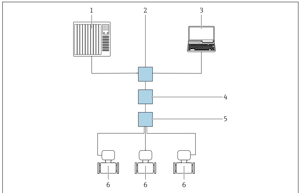
67 通过 APL 网络进行远程操作
