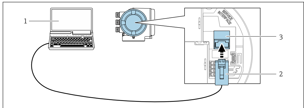
图 69 通过服务接口 (CDI-RJ45) 连接
