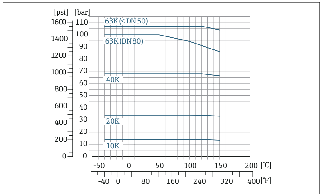
图 34 法兰材质: 1.4404 (F316/F316L)
