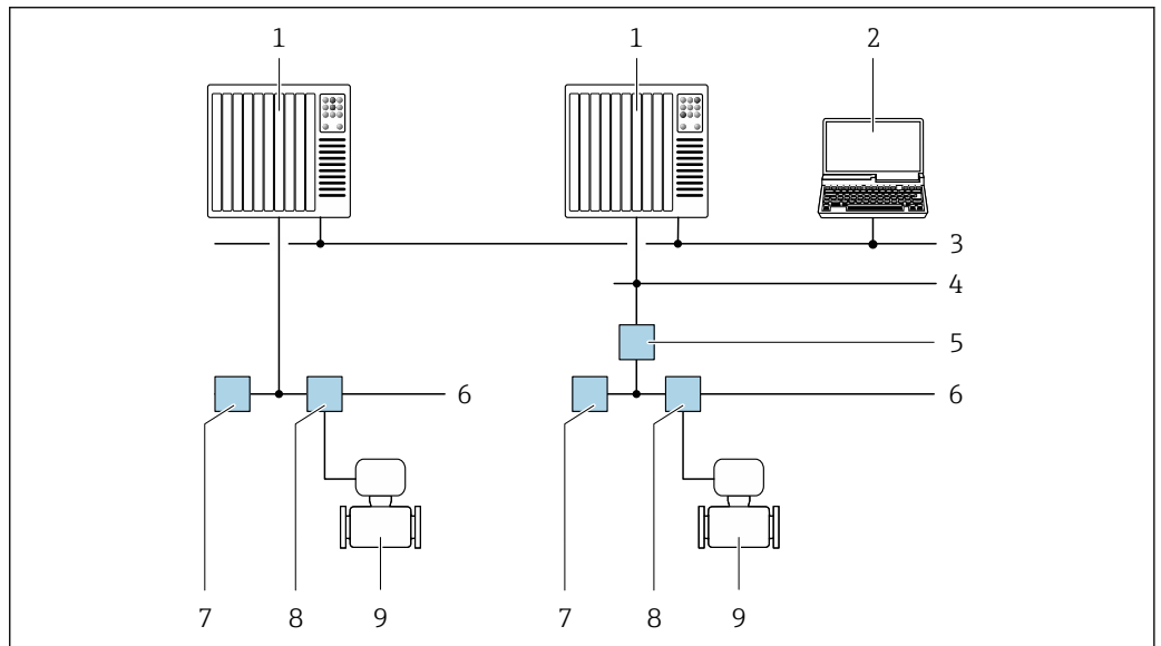
图 59 通过 FOUNDATION Fieldbus 网络进行远程操作
