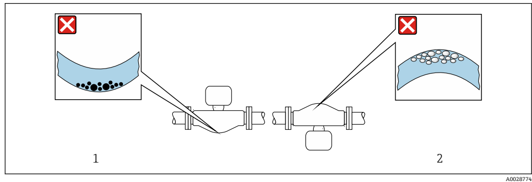
图 24 弯测量管传感器的安装方向
