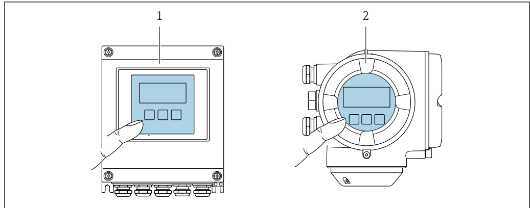
图 56 触控键操作
