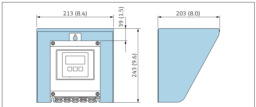
49 Proline 500 (数字) 变送器的防护罩的外形尺寸图; 单位: mm (in)
