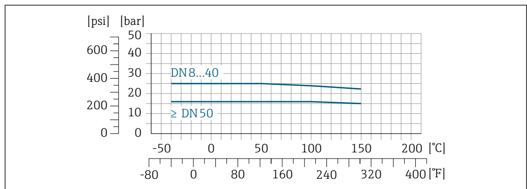
图 35 法兰材质: 1.4404 (316/316L)
