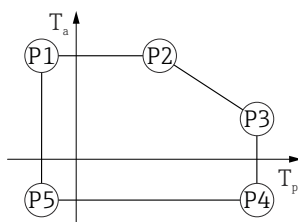
31 Caja de plástico; temperatura de proceso -40 ... +130 °C (-40 ... +266 °F)
