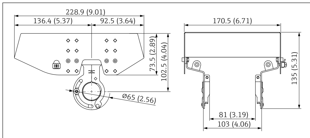
17 Medidas. Unidad de medida mm (in)
