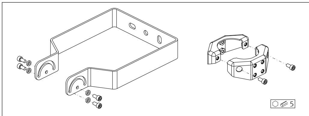
21 Alcance del suministro del soporte de montaje, ajustable
