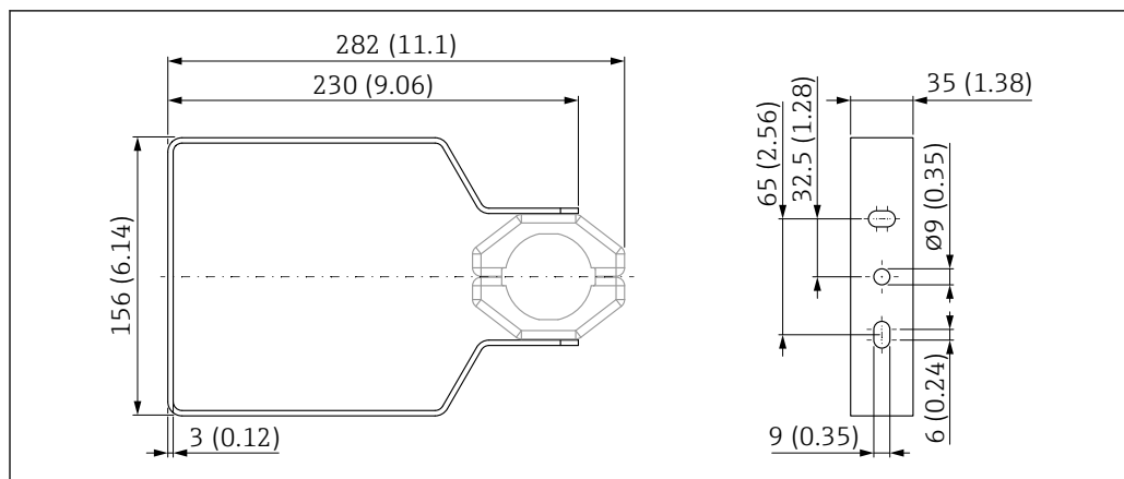
20 Dimensiones del soporte de montaje. Unidad de medida mm (in)
