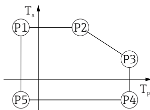
33 Caja de plástico; temperatura de proceso -40 ... +150 °C (-40 ... +302 °F)
