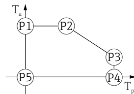
30 Caja de plástico; temperatura de proceso 0 \dots +80 \text{ }^{\circ}\text{C} ( +32 \dots +176 \text{ }^{\circ}\text{F} ) con homologación CSA C/US
