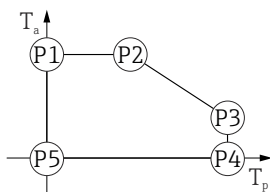
32 Caja de plástico; temperatura de proceso 0 ... +130 °C (+32 ... +266 °F) con homologación CSA C/US
