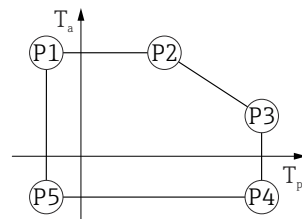
41 Caja de 316L, higiene; temperatura de proceso -40 \dots +200 \text{ }^{\circ}\text{C} ( -40 \dots +392 \text{ }^{\circ}\text{F} )
