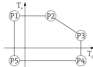
30 Caja de aluminio, recubierta; temperatura de proceso -20 ... +150 °C (-4 ... +302 °F)
