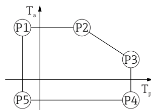
22 Caja de plástico; temperatura de proceso -20\text{ ... }+150\text{ °C} ( -4\text{ ... }+302\text{ °F} )
