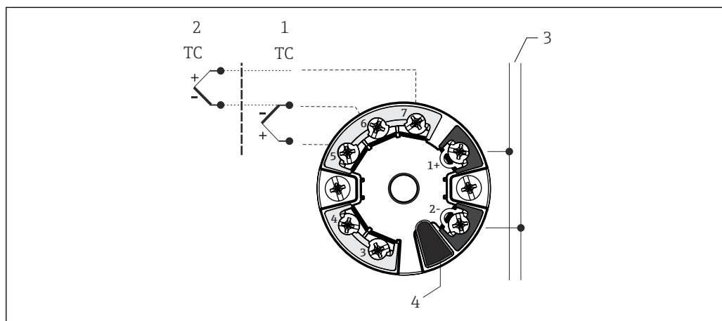
8 Trasmittitore da testa TMT8x (doppio ingresso)
