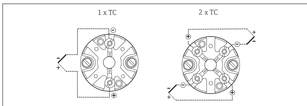
5 Morsettiera montata
