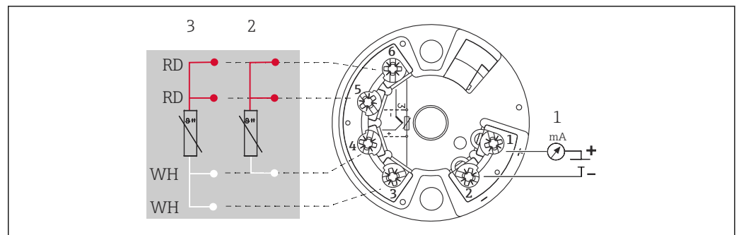
2 Trasmettitore da testa TMT18x (ingresso singolo)
