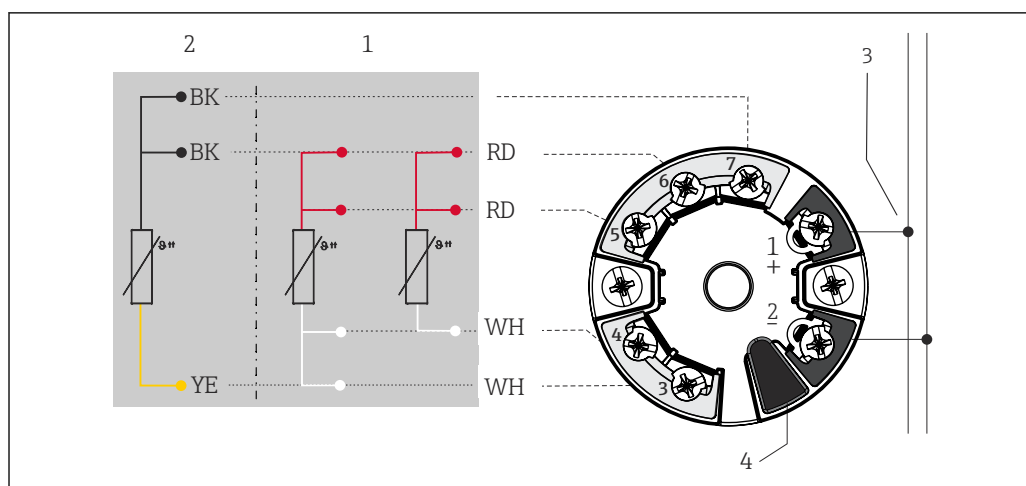
4 Trasmittitore da testa TMT8x (doppio ingresso)
