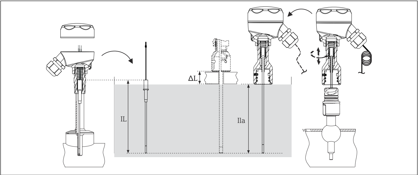
9 Lunghezze dell'inserzione per la taratura dei sensori
