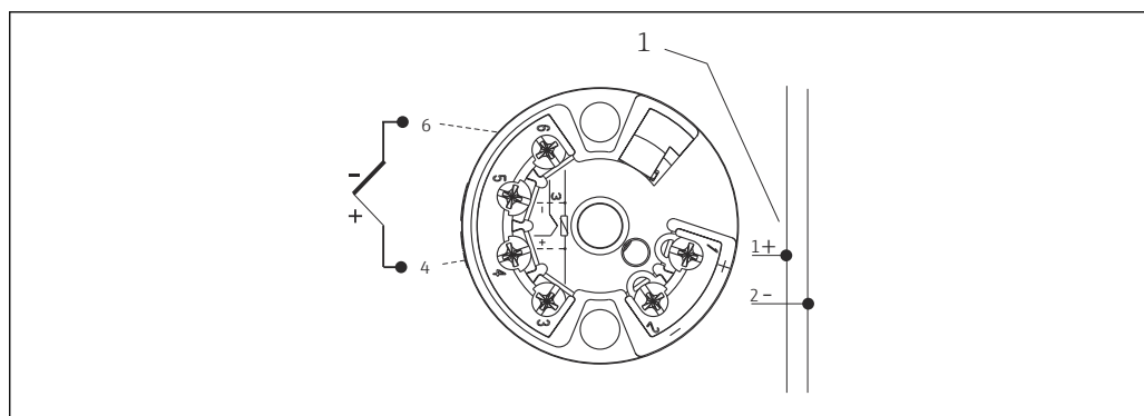
6 Trasmittitore da testa TMT18x (ingresso singolo)
