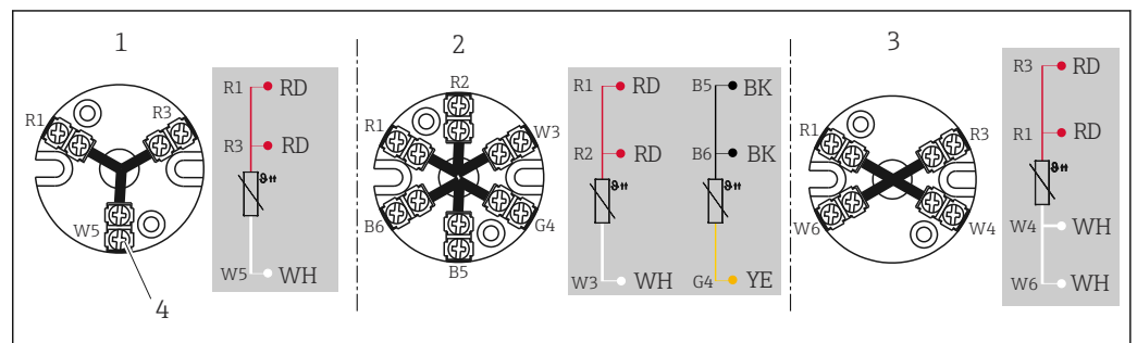
1 Morsettiera montata
