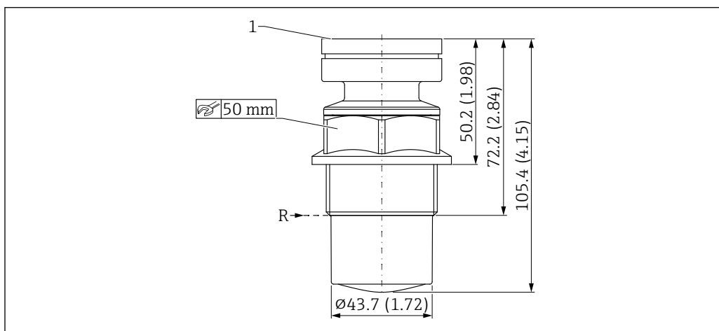
46 Dimensions de l'antenne encapsulée, PVDF, 40 mm (1,5 in). Unité de mesure mm (in)
