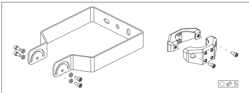
69 Contenu de la livraison de l'étrier de montage, réglable
