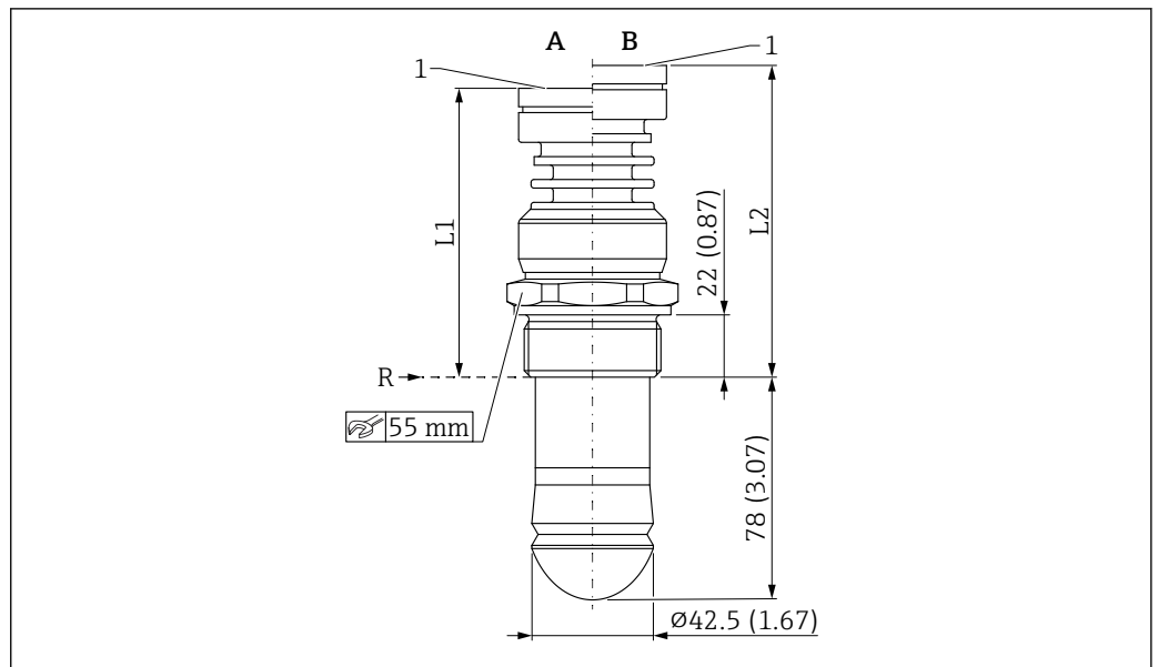
51 Dimensions de l'antenne drip-off 50 mm (2 in), raccord process fileté. Unité de mesure mm (in)
