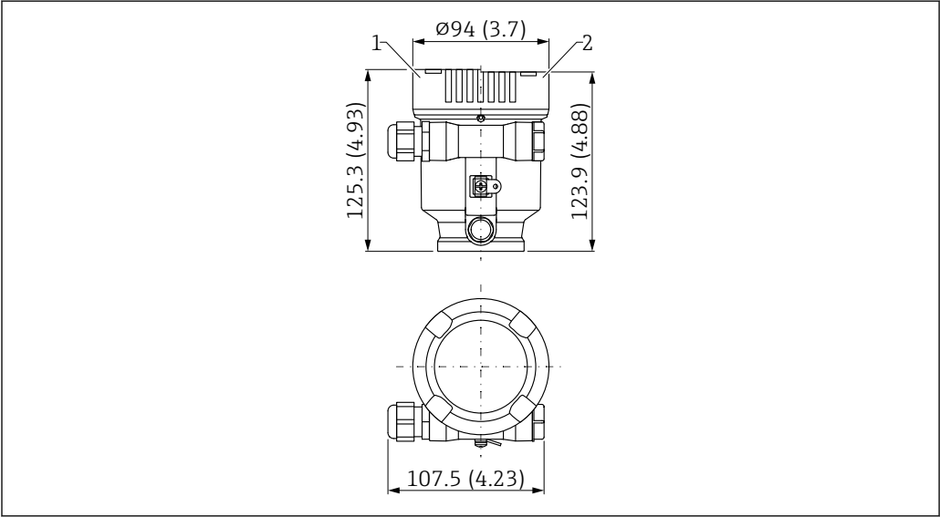
41 Dimensions du boîtier à simple compartiment, plastique (PBT). Unité de mesure mm (in)
