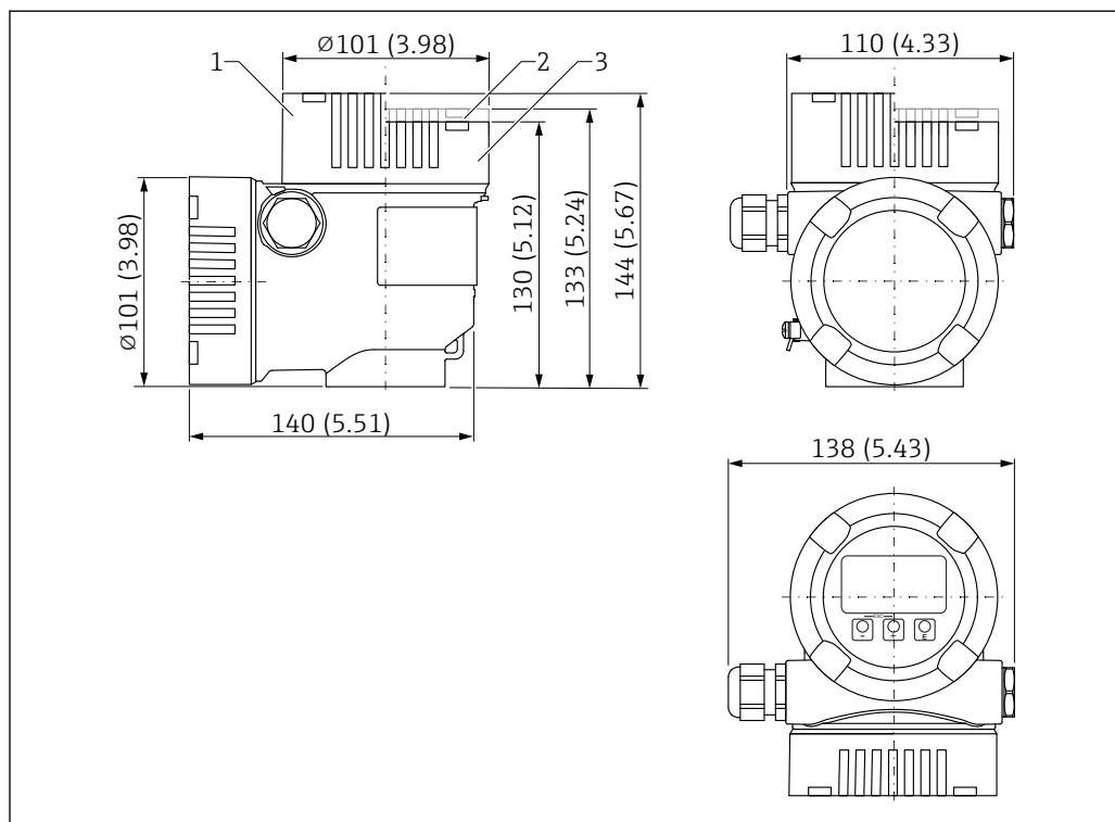
45 Размеры корпуса с двумя отсеками, L-образная форма. Единица измерения мм (дюйм)
