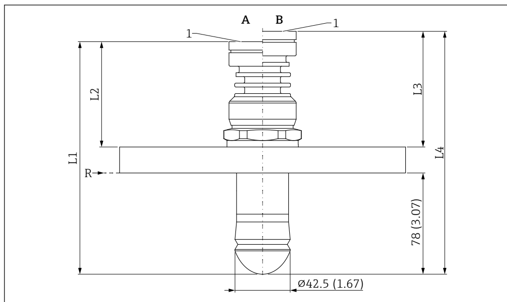
52 Размеры антенны с защитой от конденсата 50 мм (2 дюйм), присоединение к процессу – фланец UNI. Единица измерения мм (дюйм)
