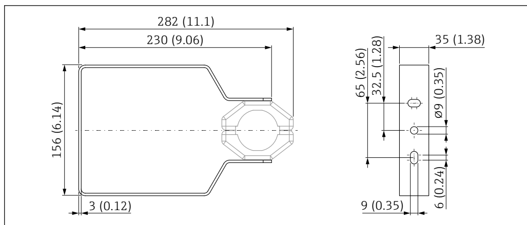
68 Размеры монтажного кронштейна. Единица измерения мм (дюйм)
