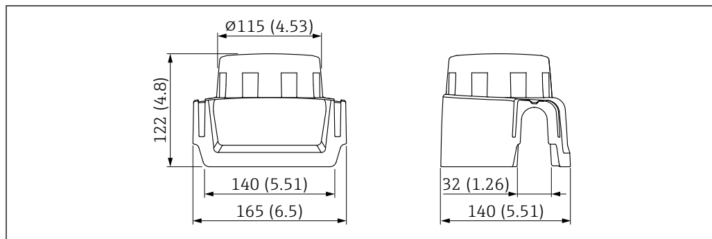
66 Размеры. Единица измерения мм (дюйм)
