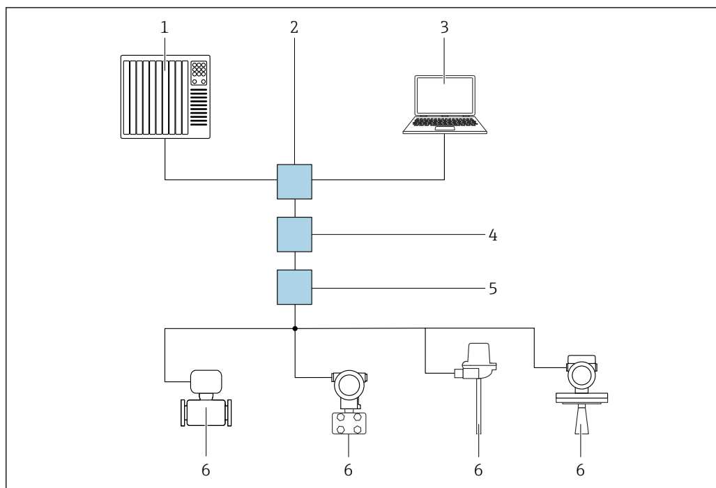
64 Варианты дистанционного управления через сеть PROFINET с Ethernet-APL: топология «звезда»
