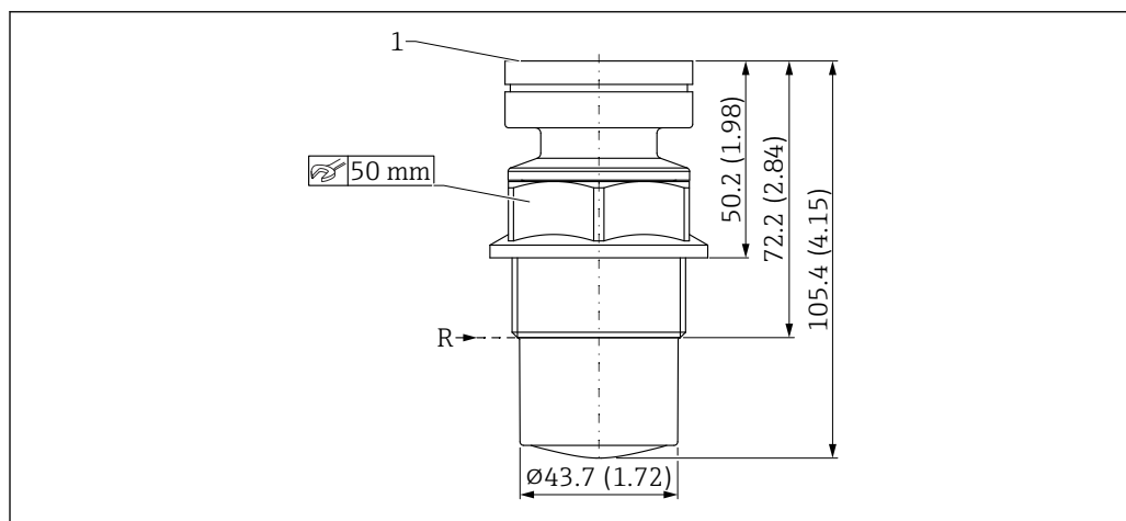
46 Размеры герметизированной антенны, PVDF, 40 мм (1,5 дюйм). Единица измерения мм (дюйм)
