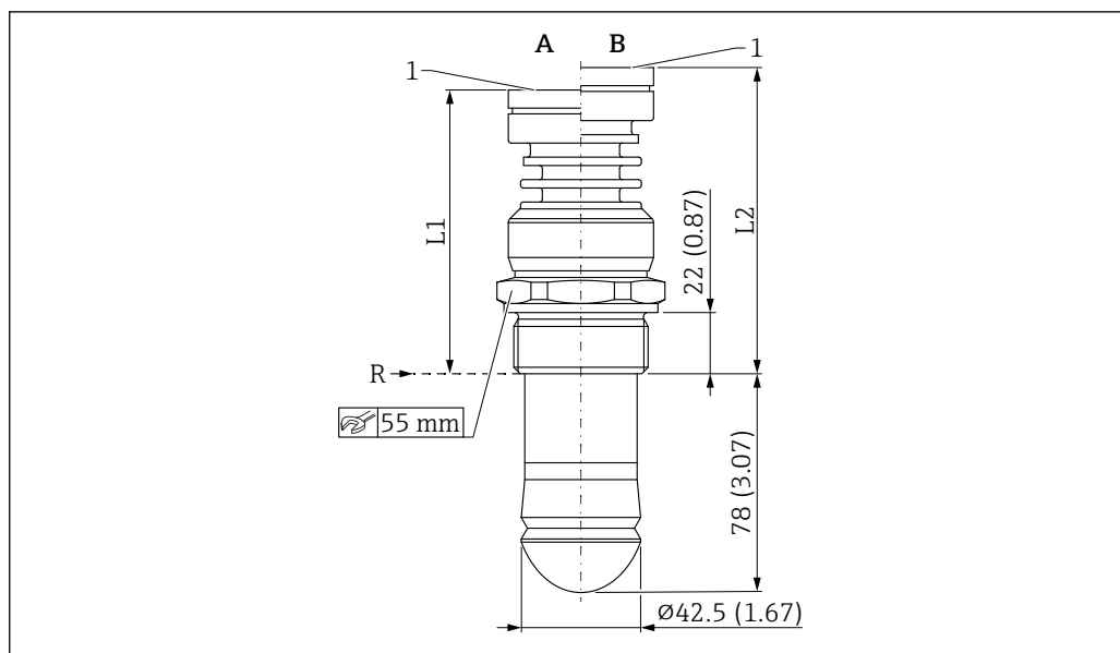
51 Размеры антенны с защитой от конденсата 50 мм (2 дюйм), резьбовое присоединение к процессу. Единица измерения мм (дюйм)
