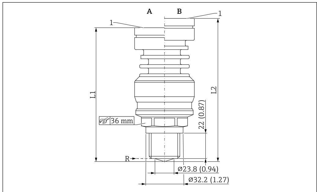
▣ 56 Размеры; встроенная антенна, РЕЕК, 20 мм (0,75 дюйм); присоединение к процессу – резьба 3/4 дюйма. Единица измерения мм (дюйм)
