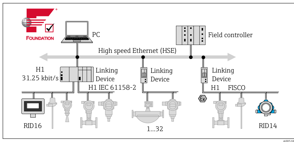
1 Systemintegration über FOUNDATION Fieldbus™
