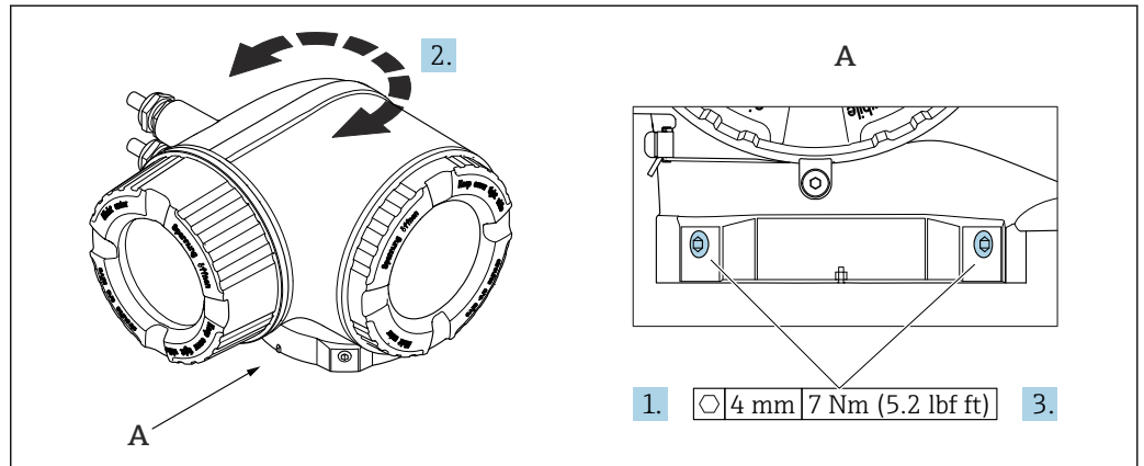
图 15 防爆型外壳
