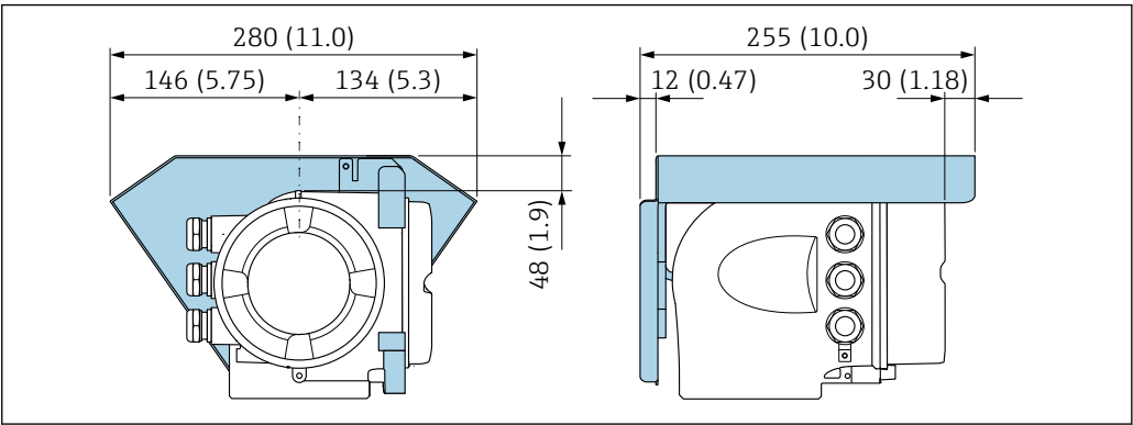
42 Proline 500（模拟）变送器的防护罩的外形尺寸图；单位：mm (in)
