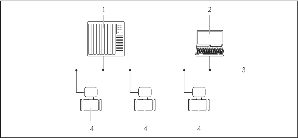
52 通过 PROFIBUS DP 网络进行远程操作
