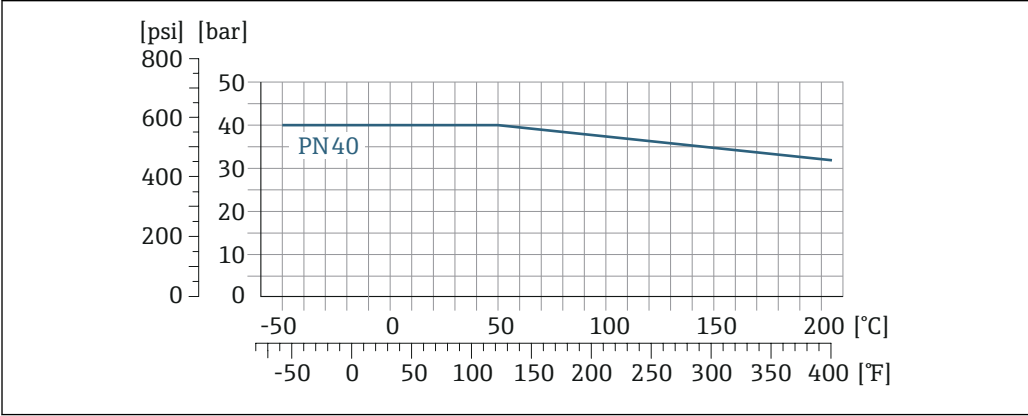
31 法兰材质: 1.4301 (304) ; 接液部件材质: 锆 702、钽
