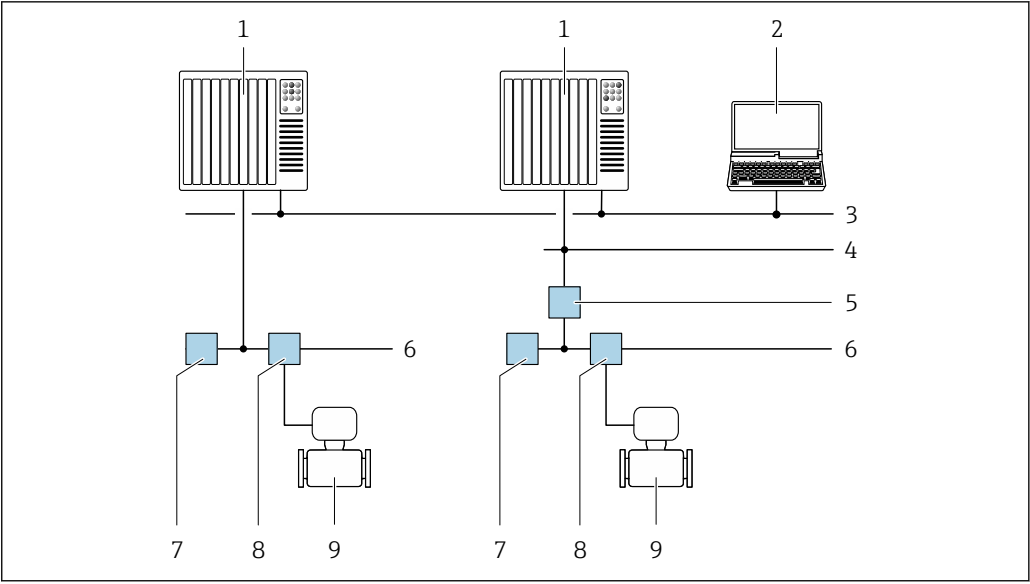
51 通过 FOUNDATION Fieldbus 网络进行远程操作
