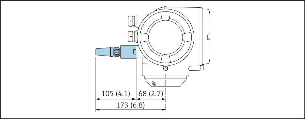
45 单位: mm (in)
