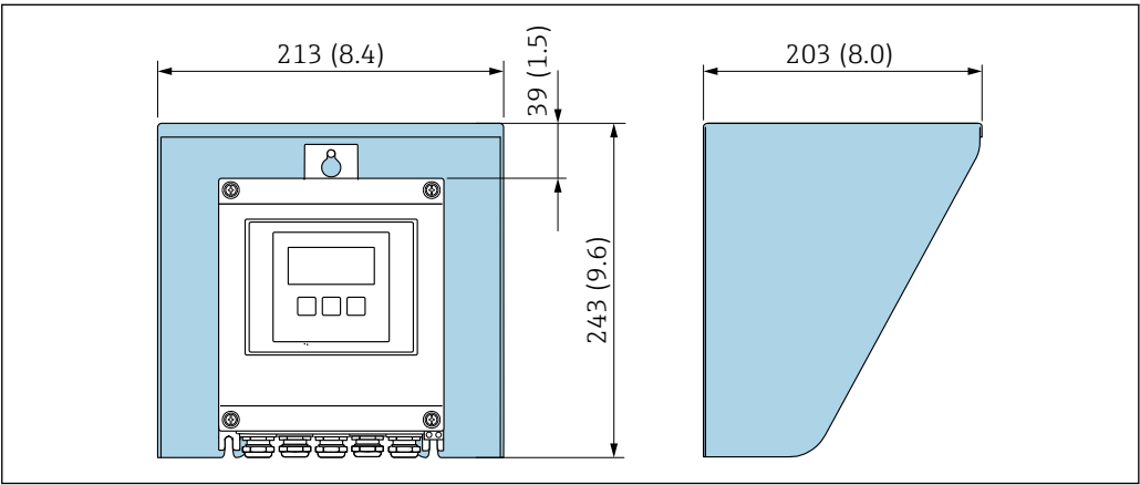
41 Proline 500（数字）变送器的防护罩的外形尺寸图；单位：mm (in)
