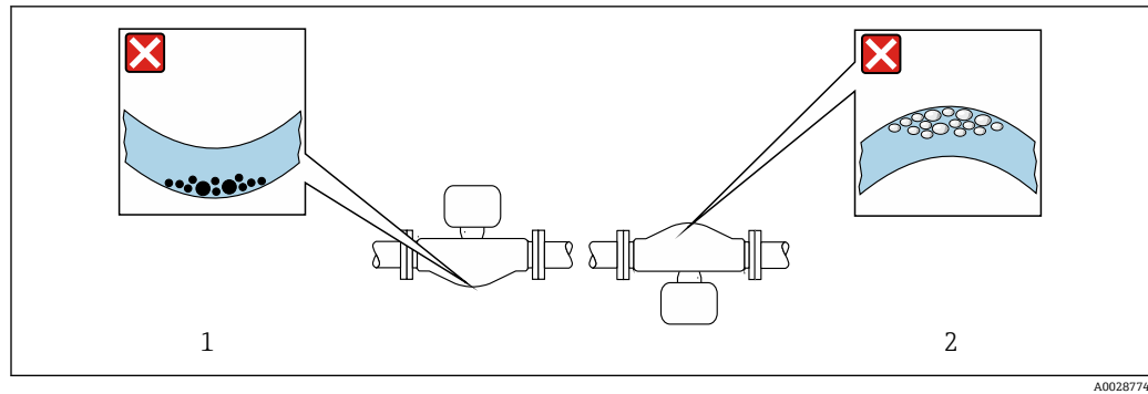
图 23 弯测量管传感器的安装方向
