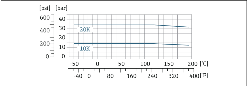
图 33 法兰材质: 1.4301 (304) ; 接液部件材质: 铅 702、铝
