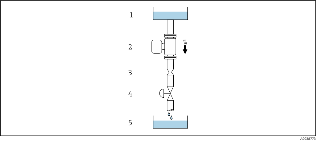
图 22 安装在竖直向下管道中（例如批处理应用）
