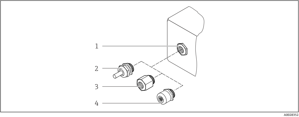
图 47 允许的电缆入口/缆塞
