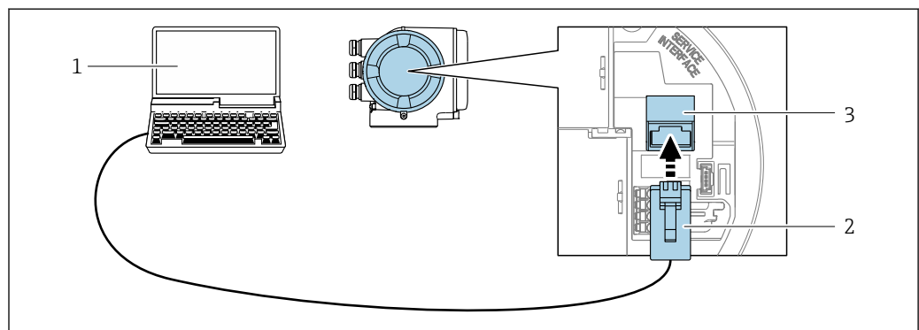
图 61 通过服务接口 (CDI-RJ45) 连接
