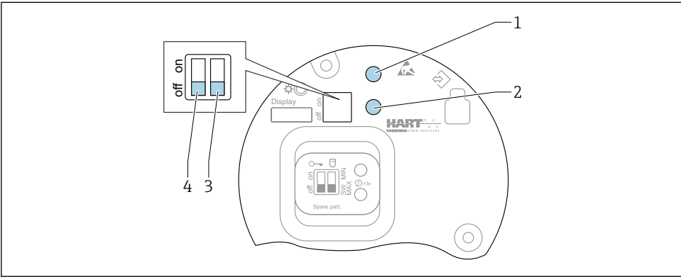
图 7 HART 电子插件上的操作按键和 DIP 开关
