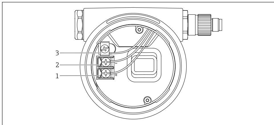
图 4 接线腔中的接线端子和接地端
