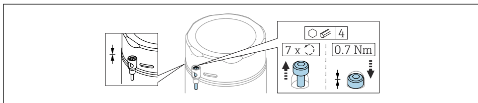
图 2 带锁定螺丝的外壳盖；卫生型外壳（仅适用于粉尘防爆场合）
