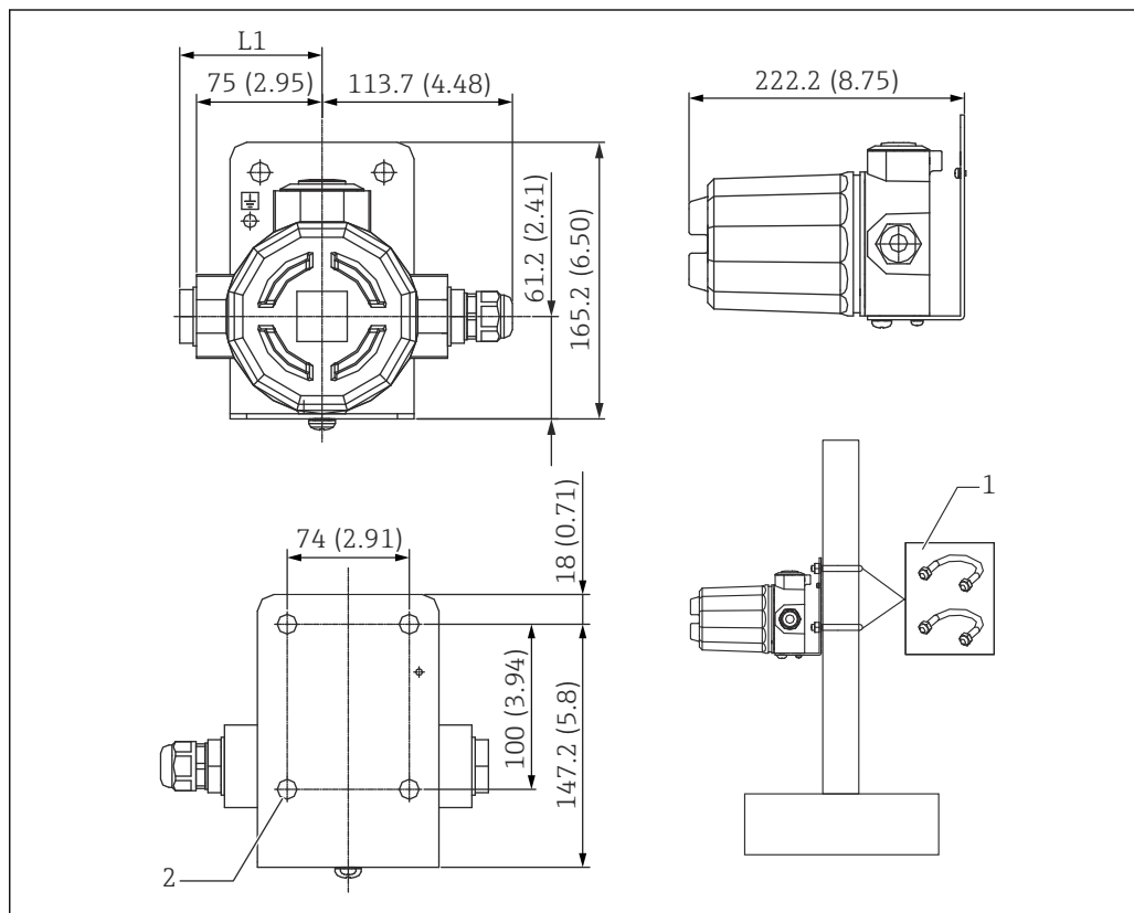
10 Внешний вид коробки датчика I/F Ex с взрывозащитой категории Ex [ia]. Единица измерения мм (дюйм)
