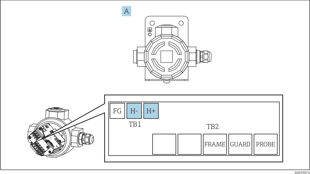
20 Искробезопасная клеммная коробка
