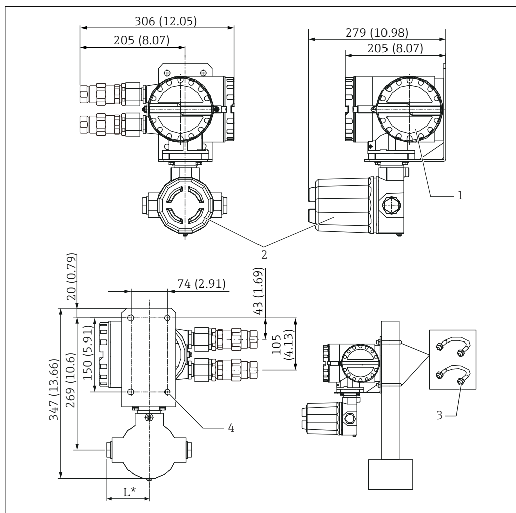
8 Внешний вид преобразователя NRR261. Единица измерения мм (дюйм)
