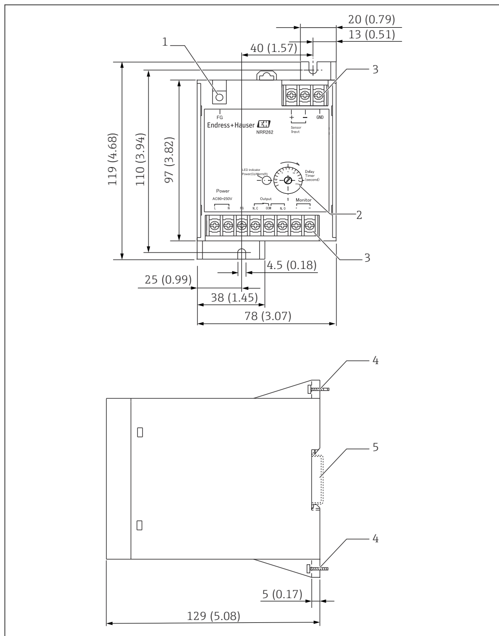
9 Внешний вид преобразователя NRR262. Единица измерения мм (дюйм)
