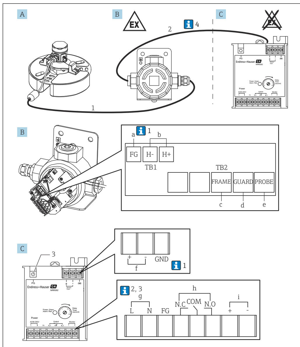
17 Подключение проводов к преобразователю NRR262-4/A/B/C с взрывозащитой категории Ex [ia]
