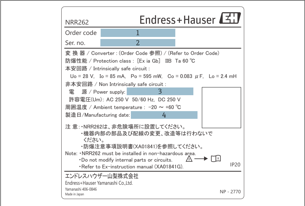
6 Заводская табличка преобразователя NRR262 с сертификатом JPN Ex 1 Код заказа 2 Серийный номер 3 Сетевое напряжение 4 Дата изготовления
