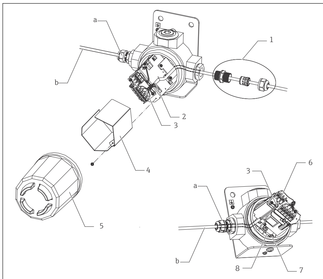
14 Монтаж кабеля, соединяющего датчик NAR300-x6xxxx с коробкой датчика I/F Ex
