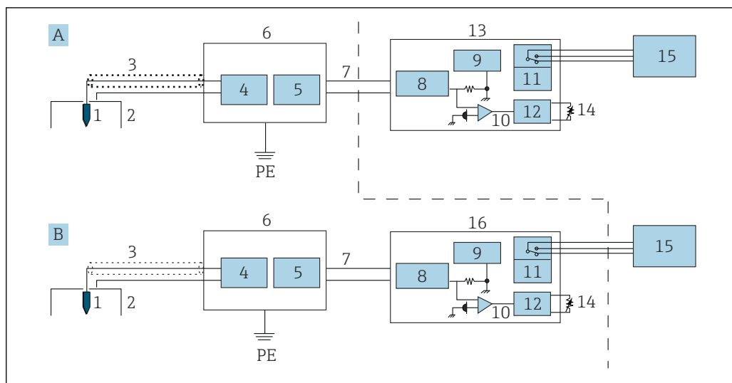
19 Схема соединений
