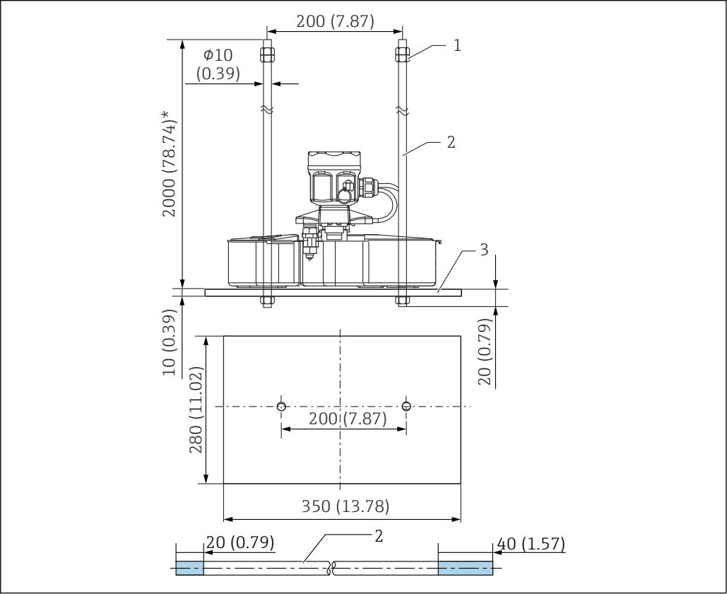
22 Направляющая поплавка
