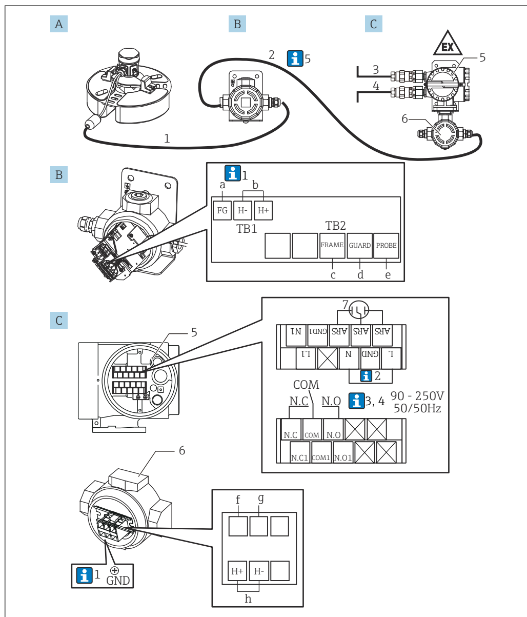
18 Подключение проводов к преобразователю NRR261-5 с взрывозащитой категории Ex d [ia]
