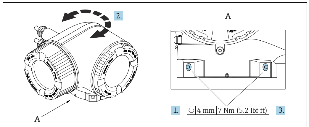
图 15 防爆型外壳
