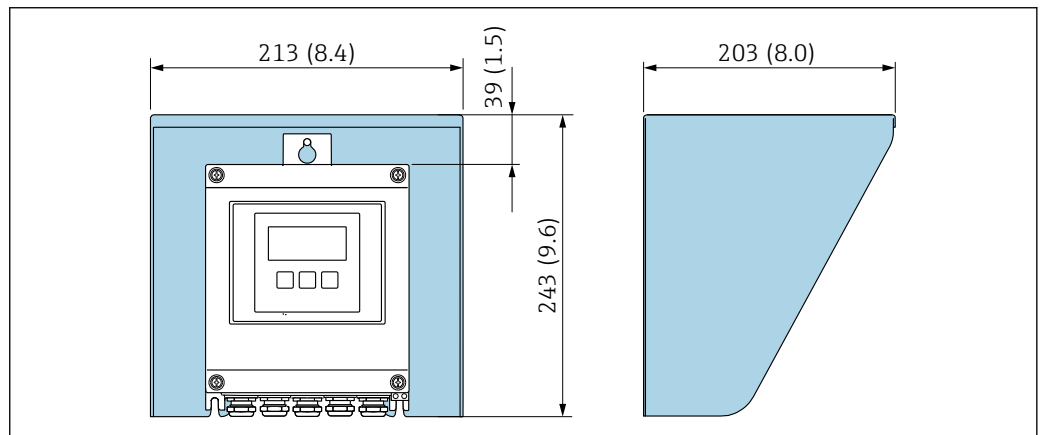
图 28 Proline 500 (数字) 变送器的防护罩的外形尺寸图; 单位: mm (in)
