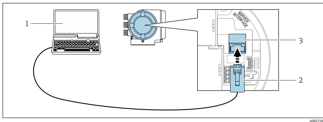
图 64 通过服务接口 (CDI-RJ45) 连接
