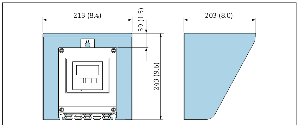
36 Proline 500 (数字) 变送器的防护罩的外形尺寸图; 单位: mm (in)
