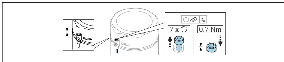
2 Deksel met borgschroef, hygiënische behuizing (alleen voor stofexplosiebeveiliging)
