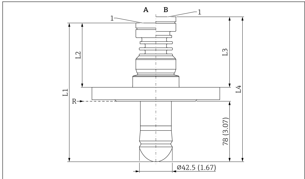
图 59 法兰过程连接的外形尺寸示意图。测量单位 mm (in)
