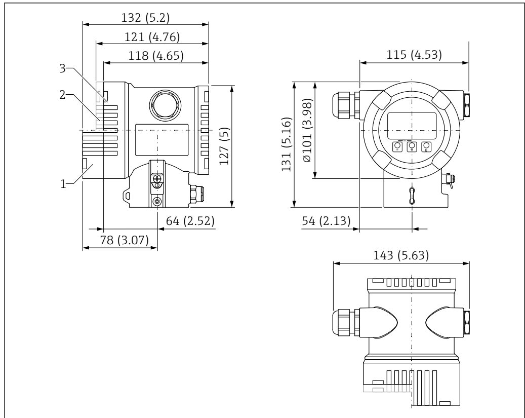
图 56 双腔室外壳的外形尺寸示意图。测量单位 mm (in)
