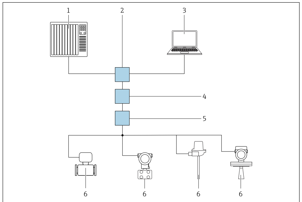
图 68 通过 PROFINET + Ethernet-APL 网络实现远程操作: 星形拓扑结构
