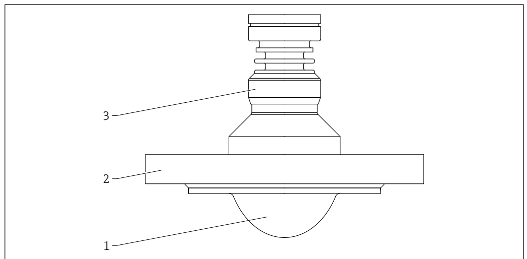
▣ 65 PTFE 涂层天线（齐平安装，80 mm (3 in)口径）的材质；带法兰
