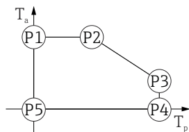
20 Boîtier plastique ; température de process 0 ... +150 °C (+32 ... +302 °F) avec agrément CSA C/US
