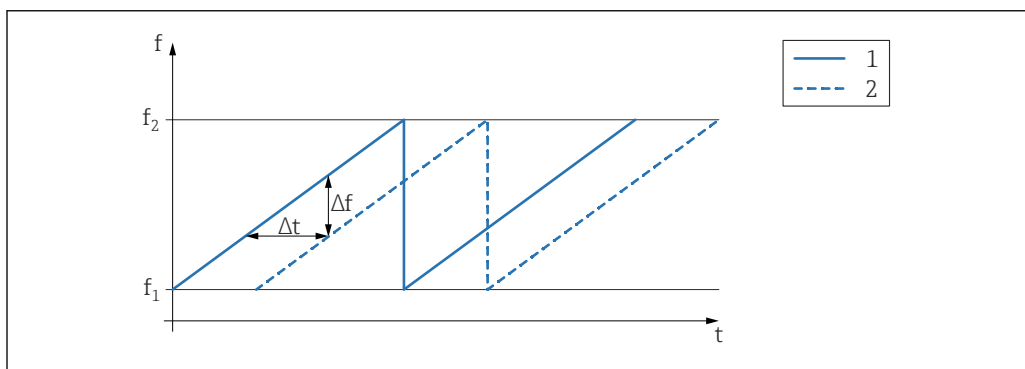
2 Principe FMCW : résultat de la modulation de fréquence
