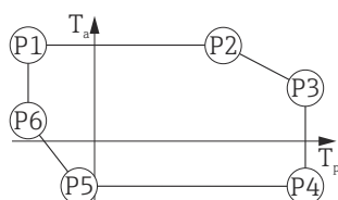
29 Boîtier plastique ; température de process -196 \dots +200 \text{ }^{\circ}\text{C} ( -320 \dots +392 \text{ }^{\circ}\text{F} )
