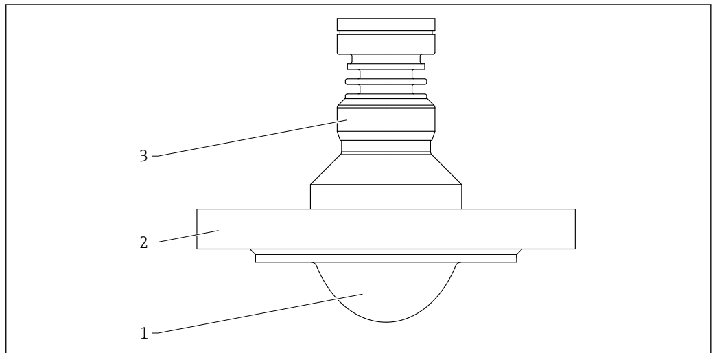
65 Matériau ; antenne, plaquée PTFE, affleurante, 80 mm (3 in), avec bride
