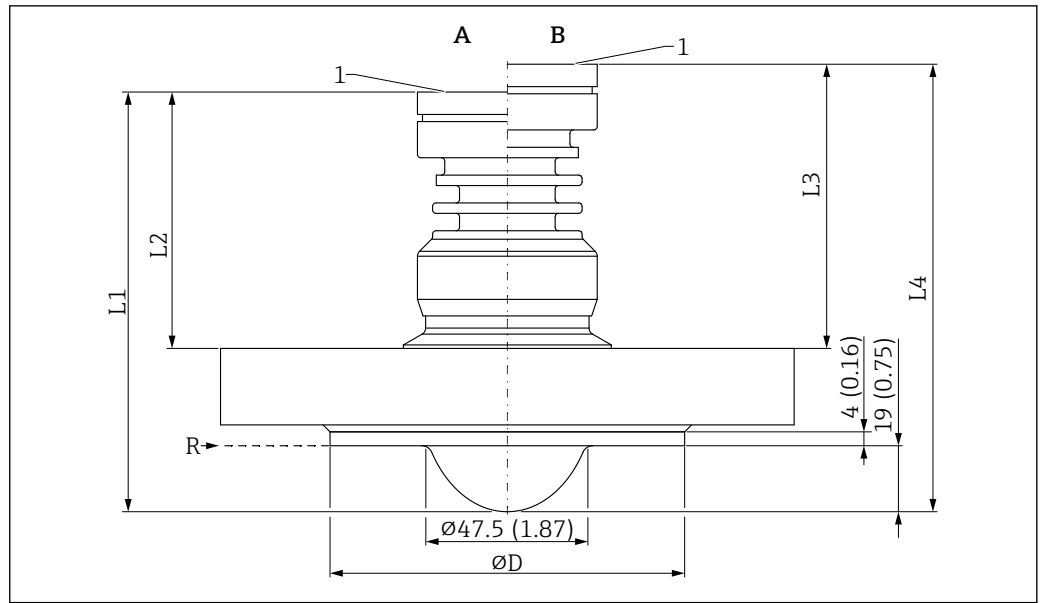
60 Dimensions de l'antenne, plaquée PTFE, affleurante, 50 mm (2 in), avec bride. Unité de mesure mm (in)
