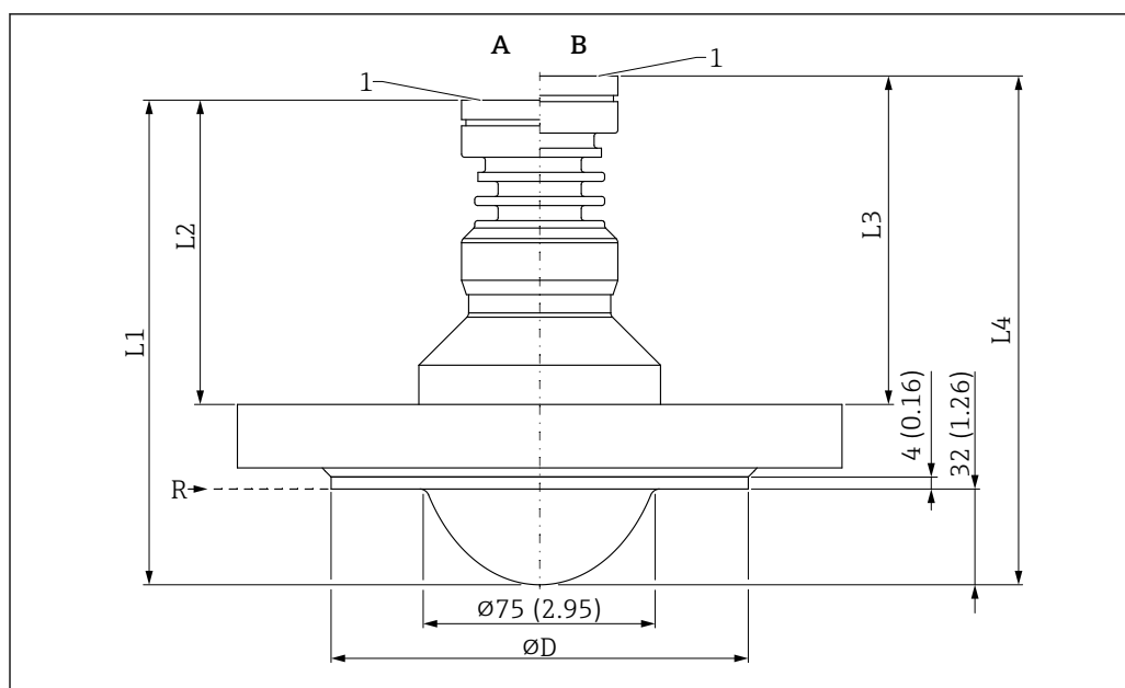
61 Dimensions de l'antenne, plaquée PTFE, affleurante, 80 mm (3 in), avec bride. Unité de mesure mm (in)
