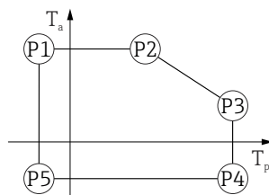
21 Boîtier plastique ; température de process -40 ... +200 °C (-40 ... +392 °F)
