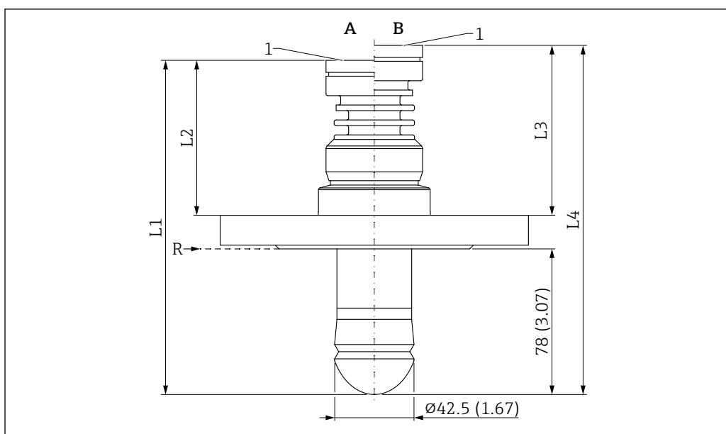
59 Dimensions du raccord process à bride. Unité de mesure mm (in)
