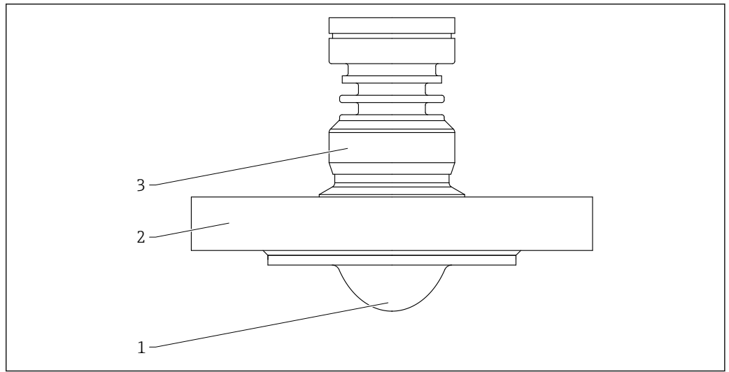
64 Matériau ; antenne, plaquée PTFE, affleurante, 50 mm (2 in), avec bride
