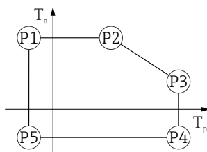
31 Boîtier alu, revêtu ; température de process -20 \dots +150 \text{ }^{\circ}\text{C} ( -4 \dots +302 \text{ }^{\circ}\text{F} )
