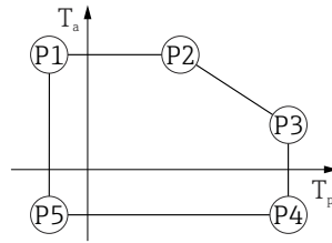
15 Boîtier plastique ; température de process -20 \dots +150 \text{ °C} ( -4 \dots +302 \text{ °F} )
