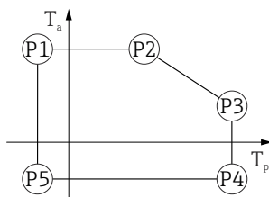
■ 25 Boîtier plastique ; température de process -40 \dots +450 \text{ }^{\circ}\text{C} ( -40 \dots +842 \text{ }^{\circ}\text{F} )
