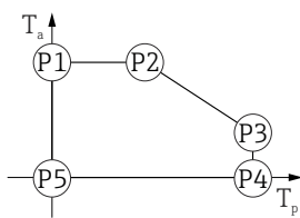
30 Agrément CSA C/US and boîtier plastique ; température de process 0 \dots +200 \text{ }^{\circ}\text{C} ( +32 \dots +392 \text{ }^{\circ}\text{F} )
