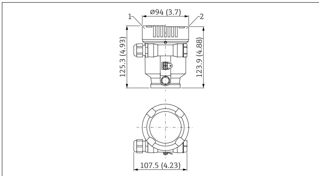
53 Размеры пластмассового корпуса с одним отсеком (PBT). Единица измерения мм (дюйм)
