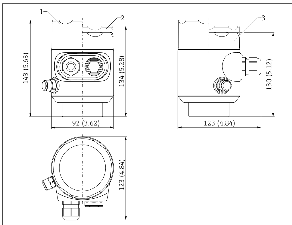
■ 55 Размеры гигиенического корпуса с одним отсеком 316L. Единица измерения мм (дюйм)
