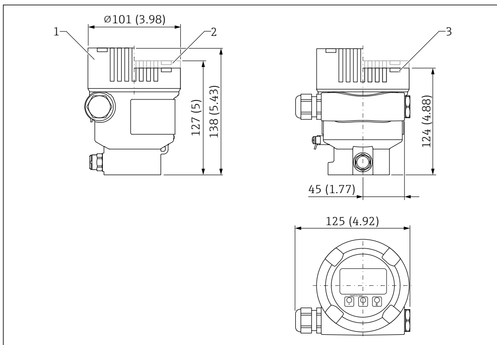
54 Размеры алюминиевого корпуса с одним отсеком. Единица измерения мм (дюйм)
