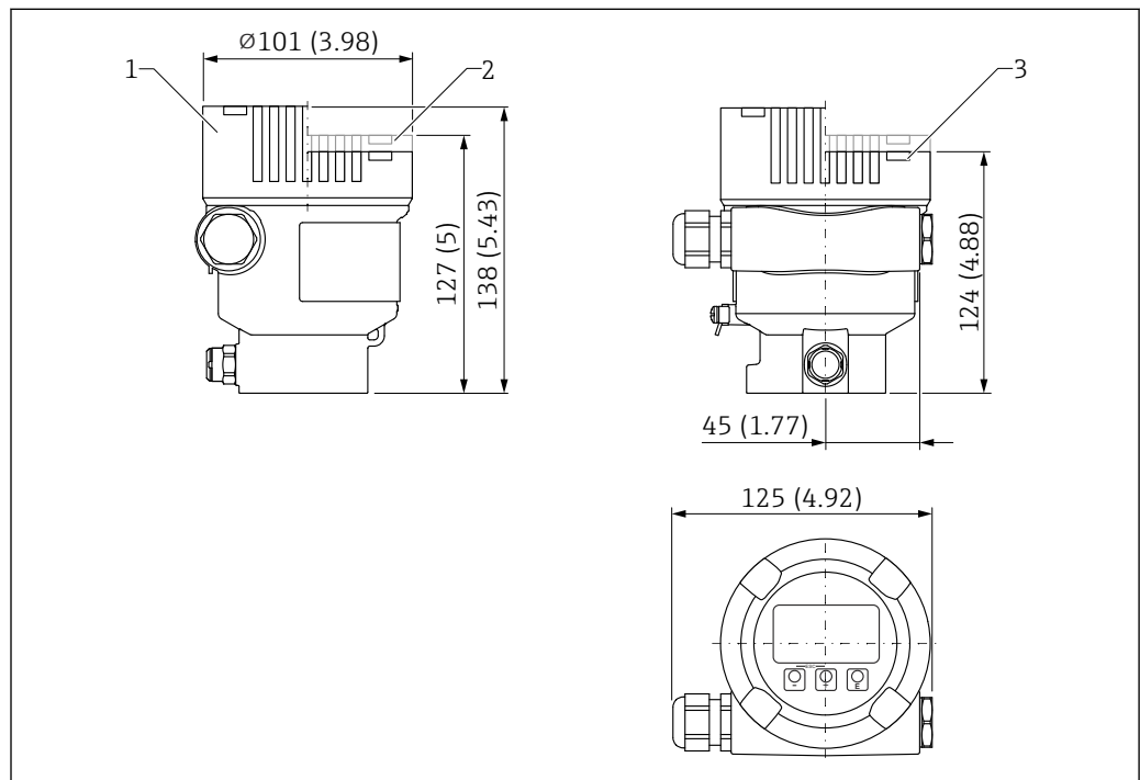
37 Medidas de la caja de aluminio de compartimento único. Unidad de medida mm (in)
