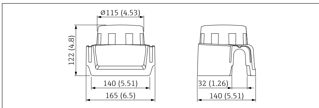
70 Medidas. Unidad de medida mm (in)
