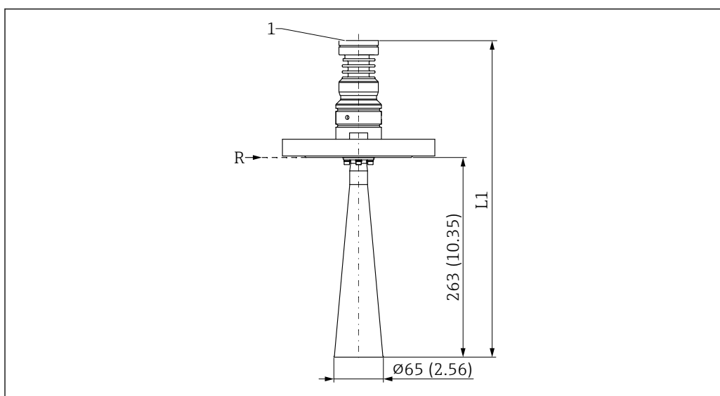
41 Medidas de la antena de trompeta DN 65: conexión a proceso de brida. Unidad de medida mm (in)
