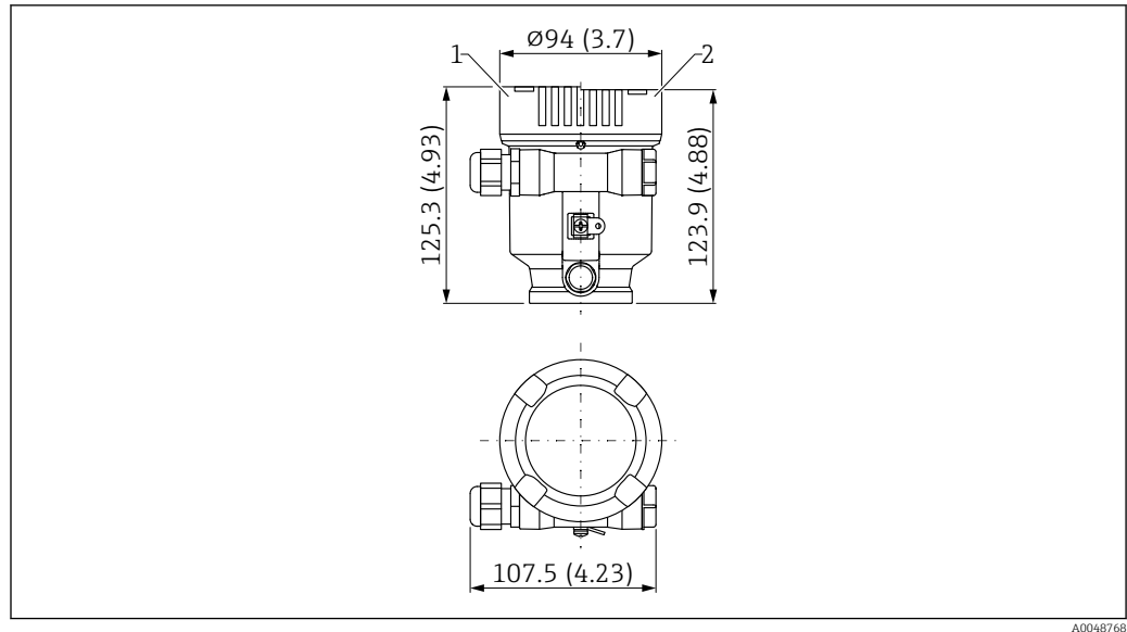
36 Medidas de la caja de compartimento único, plástico (PBT). Unidad de medida mm (in)
