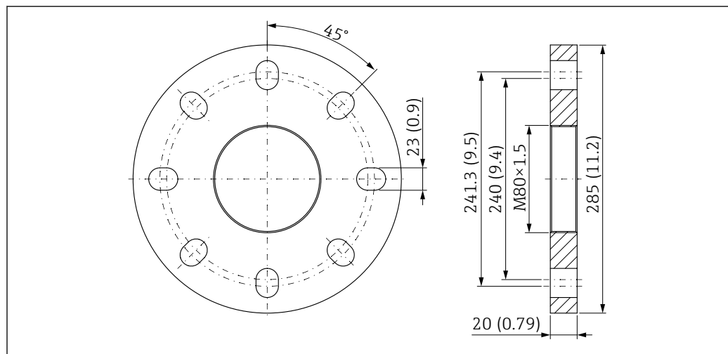
50 UNI brida 6" / DN 150 / 150 A para antena de goteo, PTFE, 50 mm (2 in) con conexión de aire de purga. Unidad de medida mm (in)
