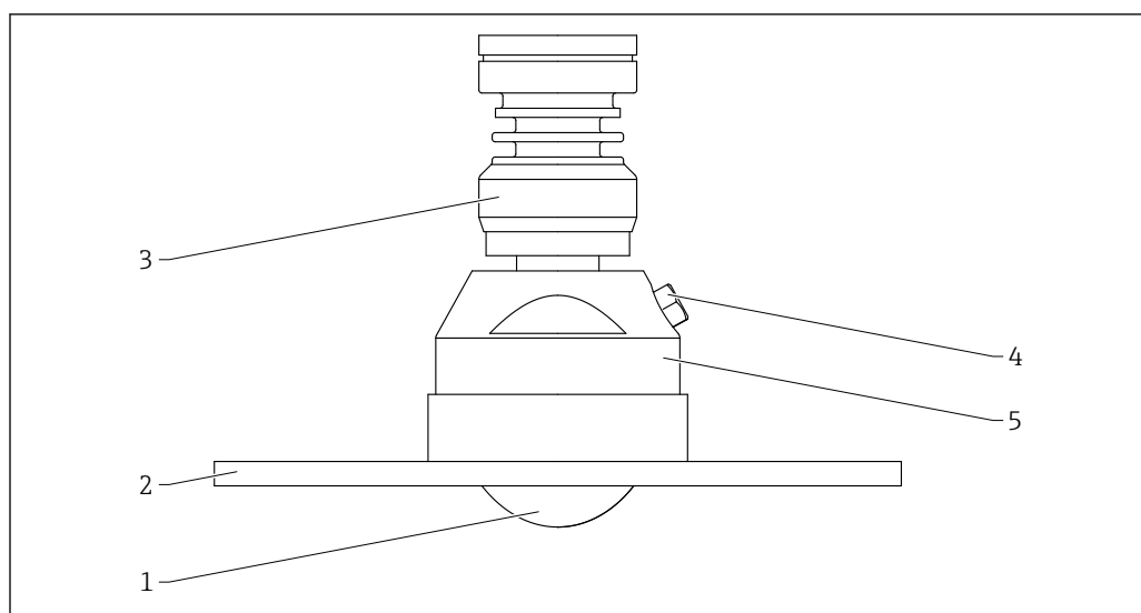
64 Material; antena de montaje enrasado, 80 mm (3 in), con brida UNI y conexión de aire de purga. Unidad de medida mm (in)
