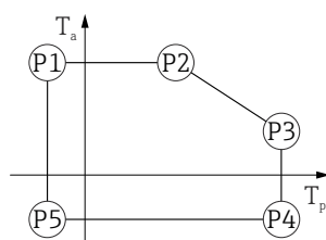
▣ 28 Caja de 316L; temperatura de proceso -40 \dots +80 \text{ }^{\circ}\text{C} ( -40 \dots +176 \text{ }^{\circ}\text{F} )
