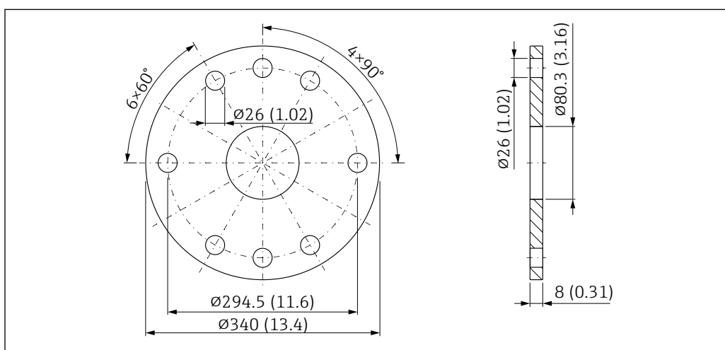
53 Medidas de la brida UNI 8" / DN 200 / 200 A para antenas DN 80 con conexión de aire de purga. Unidad de medida mm (in)
