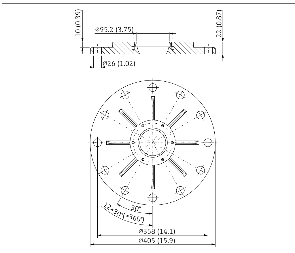
59 Medidas de la brida UNI 10" / DN 250 / 250 A para antenas con unidad de alineación. Unidad de medida mm (in)
