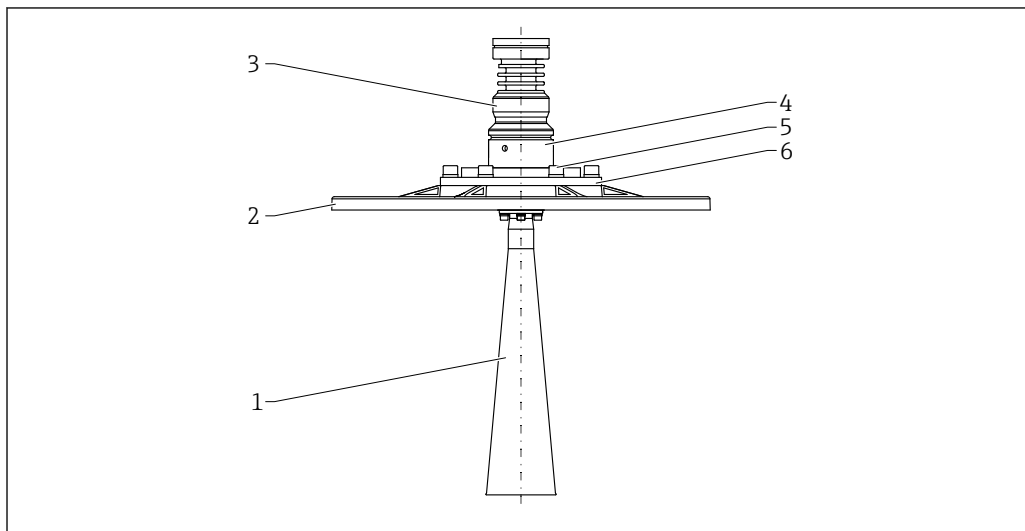
61 Material; antena de trompeta DN 65, con brida UNI y unidad de alineación. Unidad de medida mm (in)
