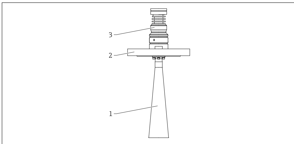
60 Material; antena de trompeta DN 65. Unidad de medida mm (in)
