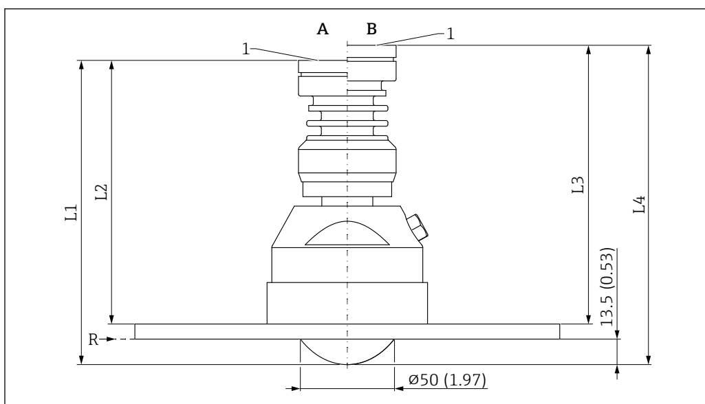
52 Medidas de la antena de montaje enrasado, PTFE, 80 mm (3 in), con brida UNI y conexión de aire de purga. Unidad de medida mm (in)
