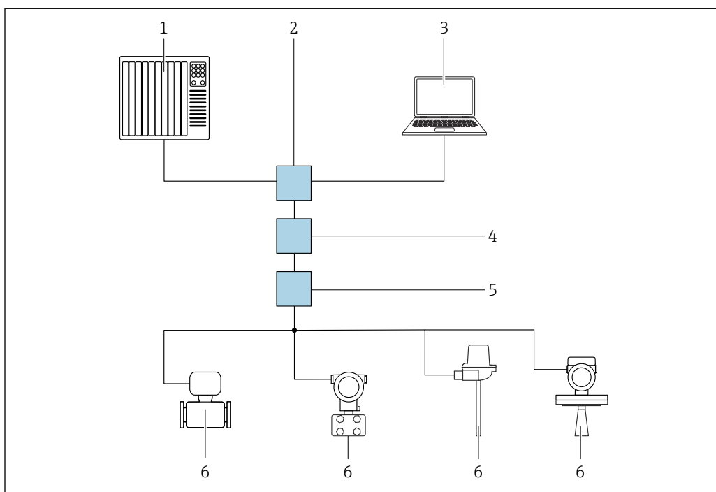
68 Opciones para la configuración a distancia a través de la red PROFINET con Ethernet-APL: topología en estrella
