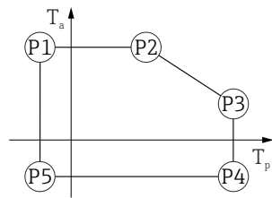
38 Boîtier 316L ; température de process -40 ... +130 °C (-40 ... +266 °F)
