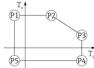
35 Boîtier alu, revêtu ; température de process -40 \dots +80 \text{ }^{\circ}\text{C} ( -40 \dots +176 \text{ }^{\circ}\text{F} )
