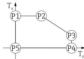
34 Boîtier plastique ; température de process 0 ... +130 °C (+32 ... +266 °F) avec agrément CSA C/US
