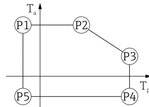
36 Boîtier alu, revêtu ; température de process -40 \dots +130 \text{ }^{\circ}\text{C} ( -40 \dots +266 \text{ }^{\circ}\text{F} )
