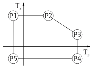
40 Boîtier 316L, app. hygiénique ; température de process -40 ... +130 °C (-40 ... +266 °F)
