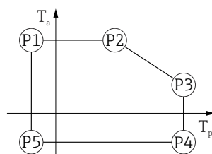
31 Boîtier plastique ; température de process -40 ... +80 °C (-40 ... +176 °F)
