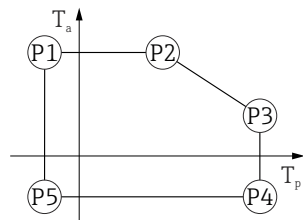
39 Boîtier 316L, app. hygiénique ; température de process -40 ... +80 °C (-40 ... +176 °F)
