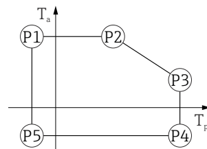
37 Boîtier 316L ; température de process -40 \dots +80 \text{ }^{\circ}\text{C} ( -40 \dots +176 \text{ }^{\circ}\text{F} )
