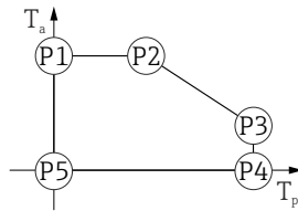
图 32 塑料外壳; 过程温度范围: 0 \dots +80 \text{ }^\circ\text{C} ( +32 \dots +176 \text{ }^\circ\text{F} ), 适用 CSA C/US 认证型仪表
