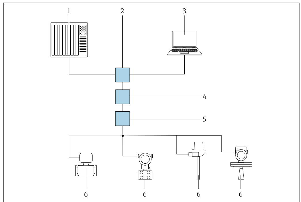
图 13 通过 PROFINET + Ethernet-APL 网络实现远程操作：星形拓扑结构
