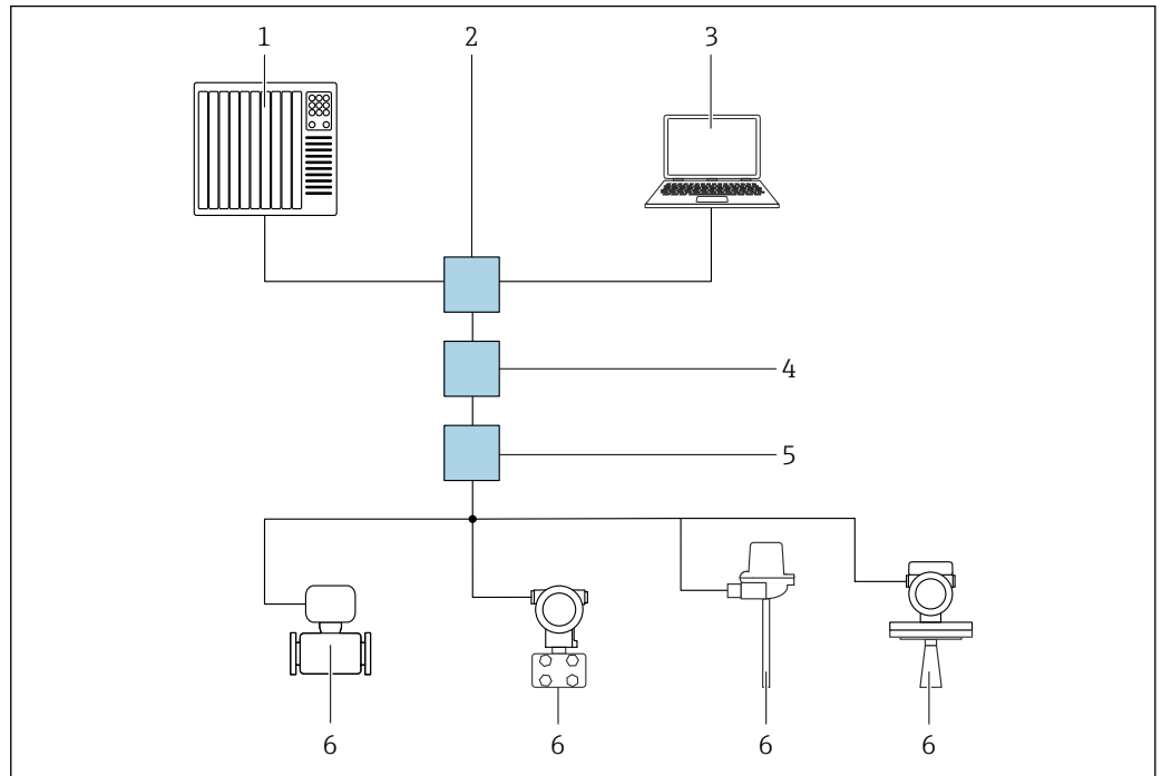
图 17 通过 PROFINET + Ethernet-APL 网络实现远程操作：星形拓扑结构
