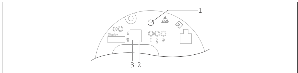
图 11 Ethernet-APL 电子插件上的操作按键和 DIP 开关
