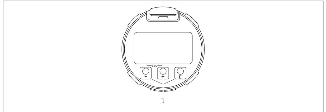
图 12 图形显示屏，带光敏按键 (1)
