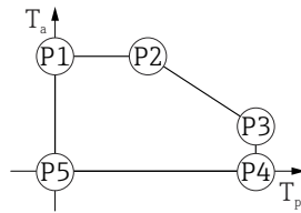
▣ 34 塑料外壳; 过程温度范围: 0 ... +150 °C (+32 ... +302 °F), 适用 CSA C/US 认证型仪表
