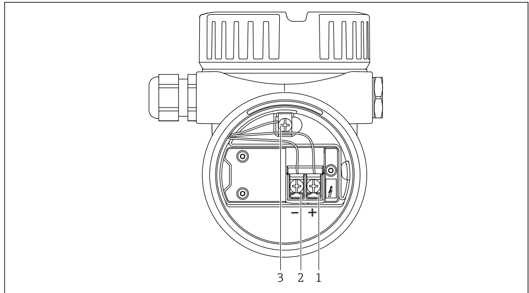
图 9 接线腔中的接线端子和接地端
