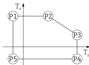
▣ 39 塑料外壳; 过程温度: -40 ... +450 °C (-40 ... +842 °F)
