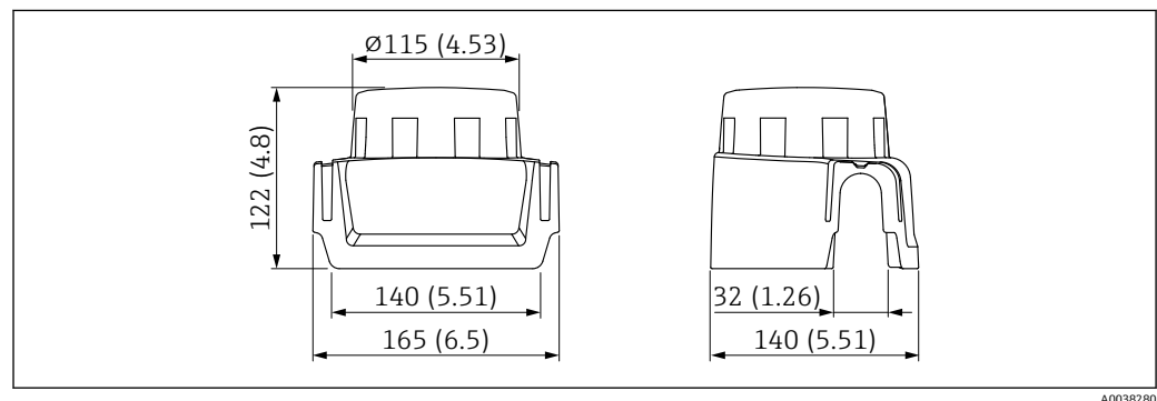
图 27 外形尺寸示意图。测量单位 mm (in)
