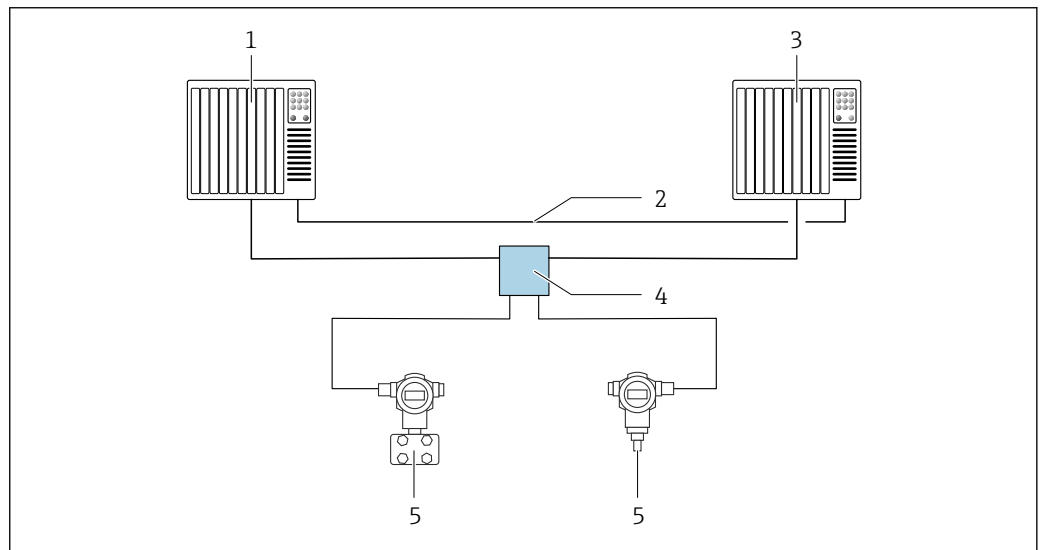
图 18 S2 系统冗余布局实例：星形拓扑结构
