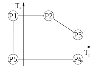
▣ 45 铝外壳, 带涂层; 过程温度: -40 ... +450 °C (-40 ... +842 °F)
