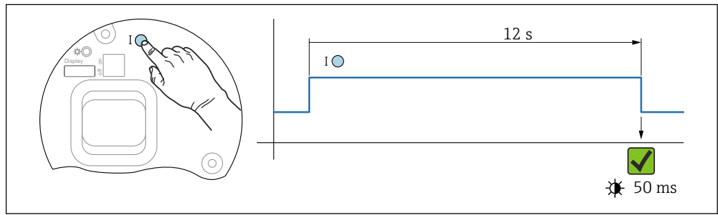
图 25 时序图 - 恢复出厂设置
