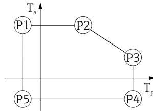
▣ 46 316L 外壳; 过程温度范围: -40 ... +80 °C (-40 ... +176 °F)
