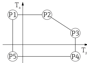
图 33 塑料外壳; 过程温度范围: -40 \dots +150 \text{ }^\circ\text{C} ( -40 \dots +302 \text{ }^\circ\text{F} )
