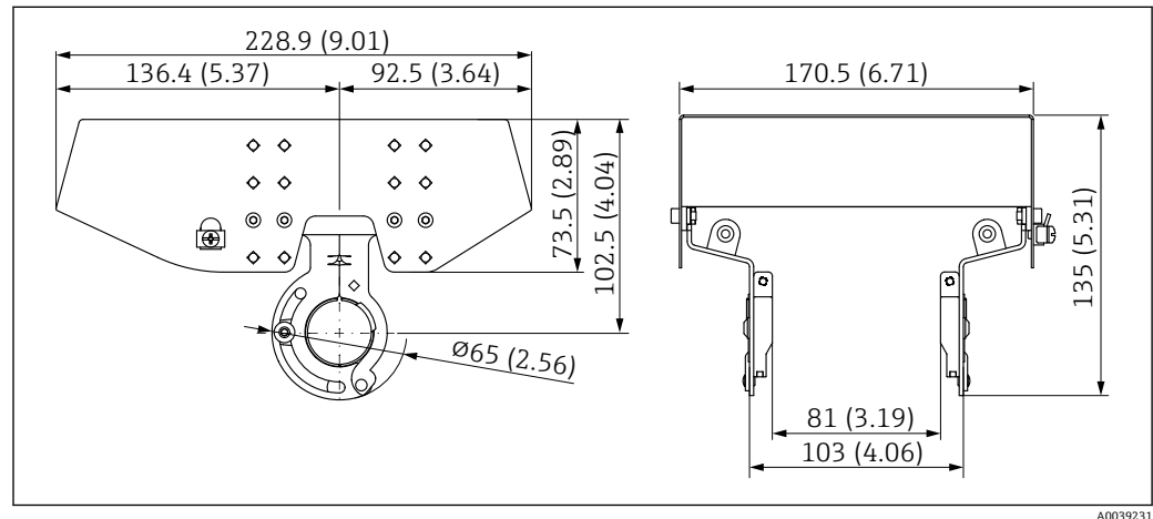
图 26 外形尺寸示意图。测量单位 mm (in)
