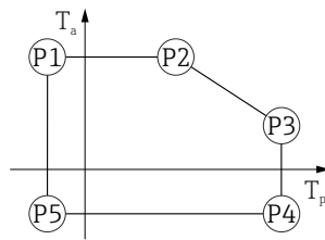
☒ 50 316L 外壳; 过程温度: -40 ... +450 °C (-40 ... +842 °F)
