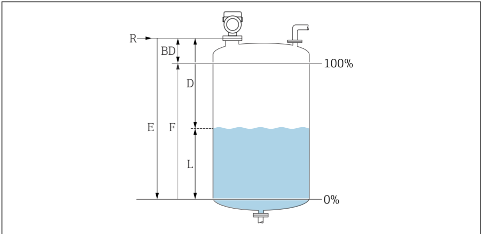
图 21 液位测量的设置参数
