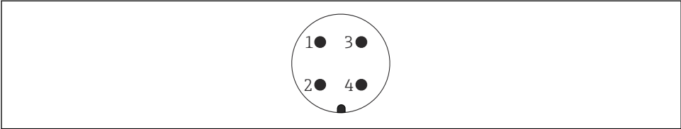
14 7/8"插头的针脚分配
