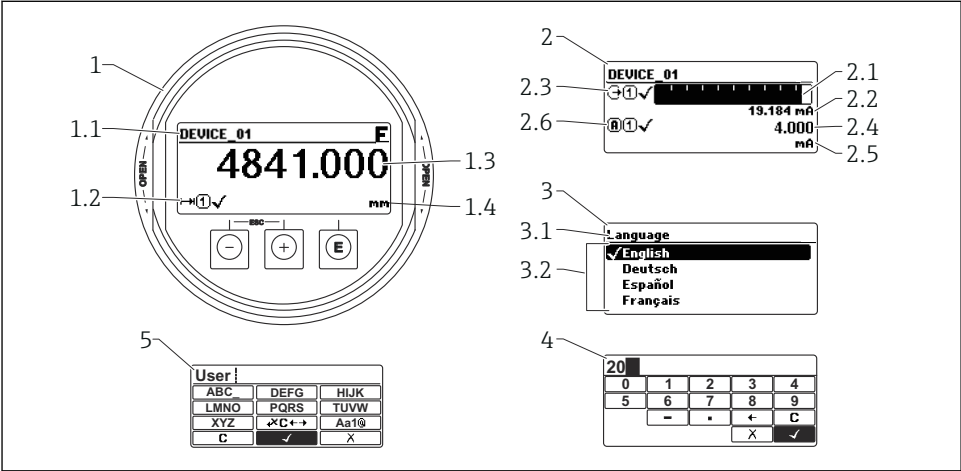
图 18 显示与操作单元的显示格式
