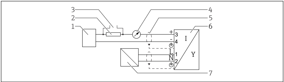
12 接线图：四线制：4 ... 20 mA HART (90 ... 253 V AC )
