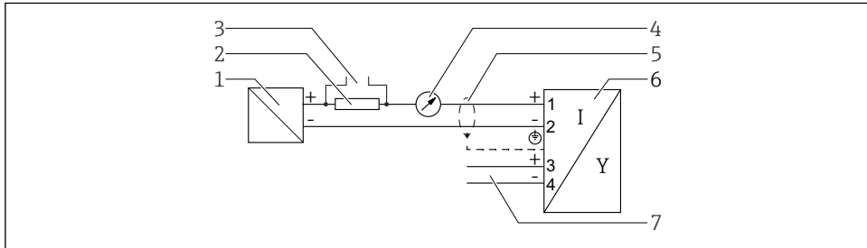
图 6 接线图：两线制：4 ... 20 mA HART，开关量输出
