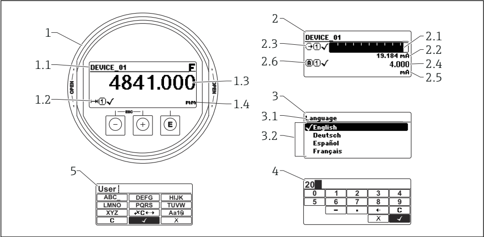
图 19 显示与操作单元的显示格式
