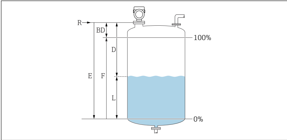
图 22 液位测量的设置参数
