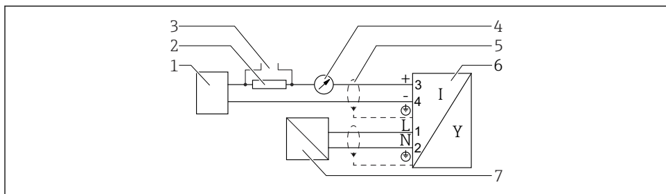
13 接线图: 四线制: 4 ... 20 mA HART (90 ... 253 V AC )
