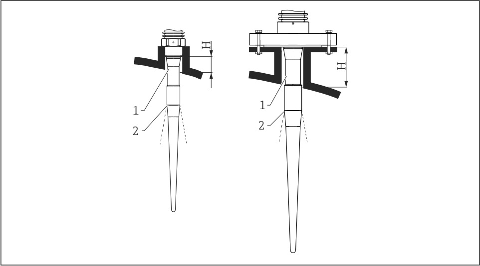
图 2 杆式天线（FMR53）的安装短管高度示意图
