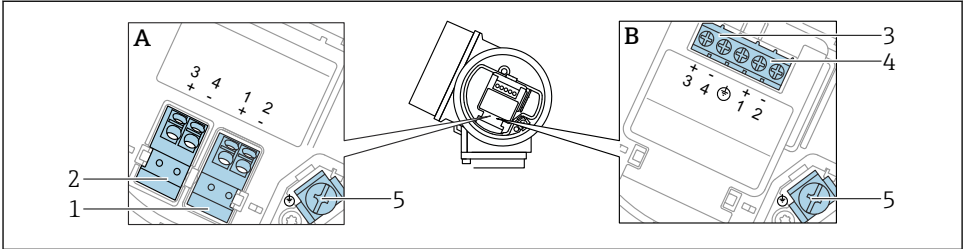
图 6 接线端子分配，两线制：4 ... 20 mA HART，开关量输出
