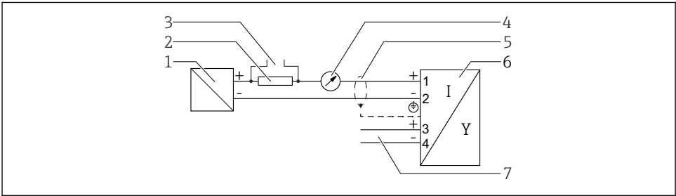
图 7 接线图：两线制：4 ... 20 mA HART，开关量输出
