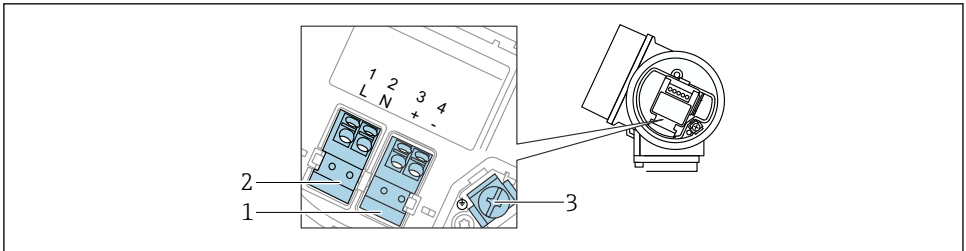
图 12 接线端子分配，四线制：4 ... 20 mA HART (90 ... 253 V AC )
